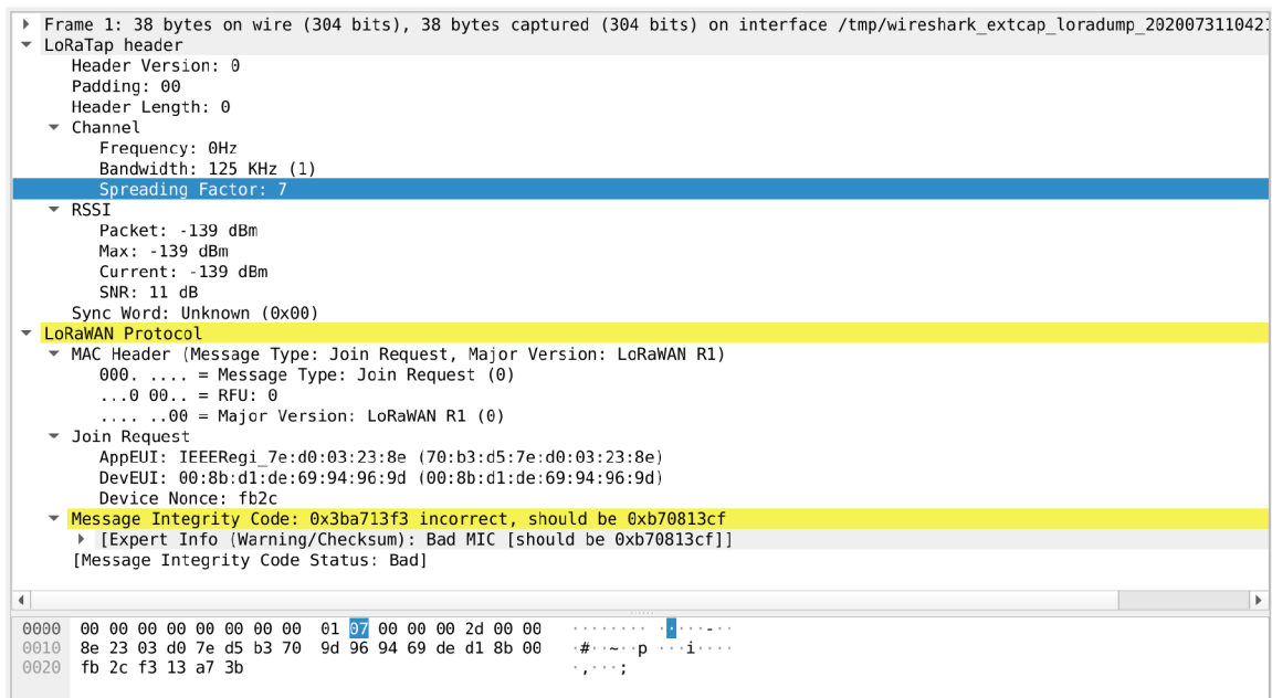
Obrázek 6.3: Wireshark - join-request
