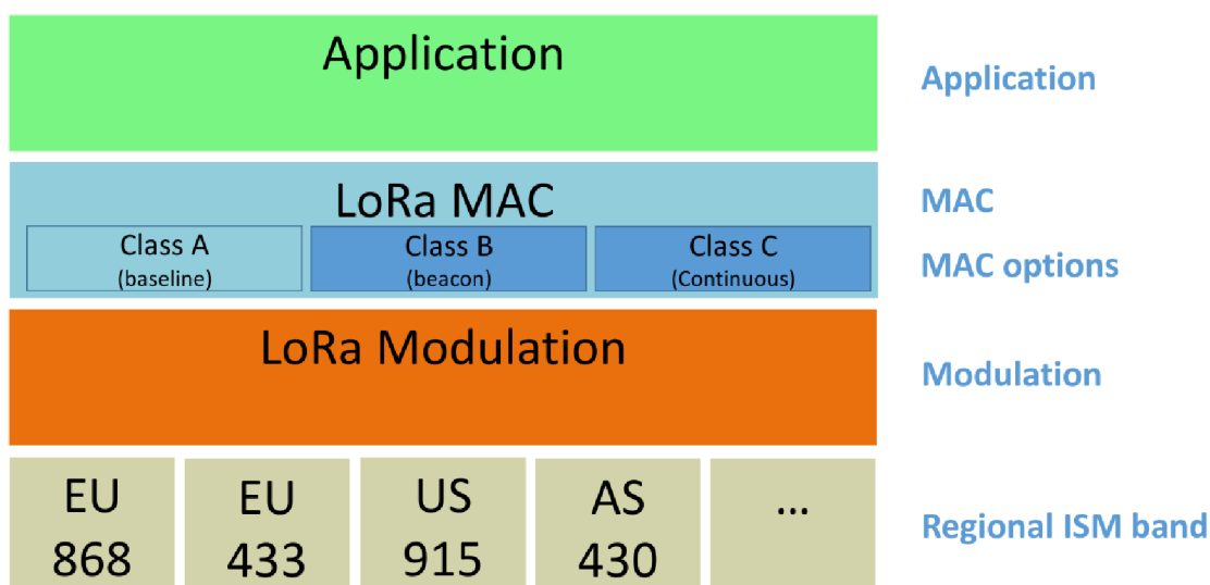
Obrázek 3.2: LoRaWAN - vrstvy [6]
