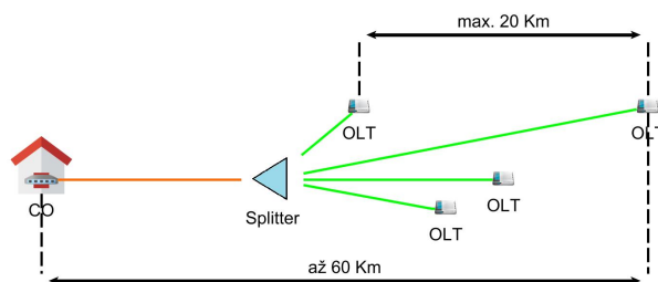
Obr. 1.3: GPON
