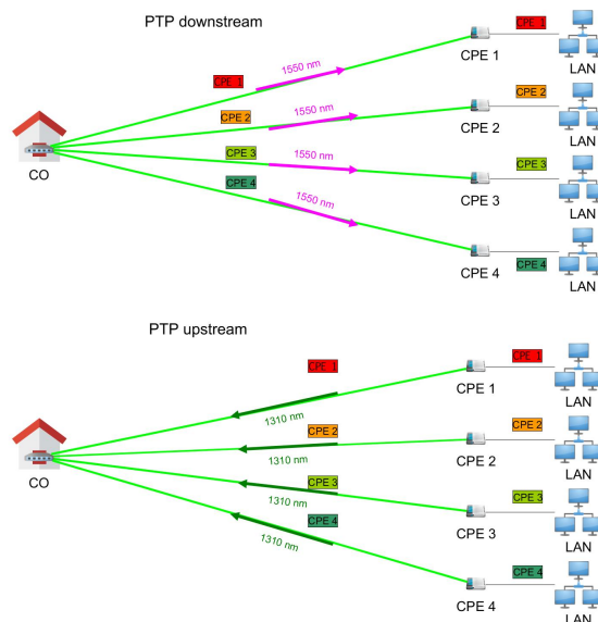
Obr. 1.1: PTP topologie.
