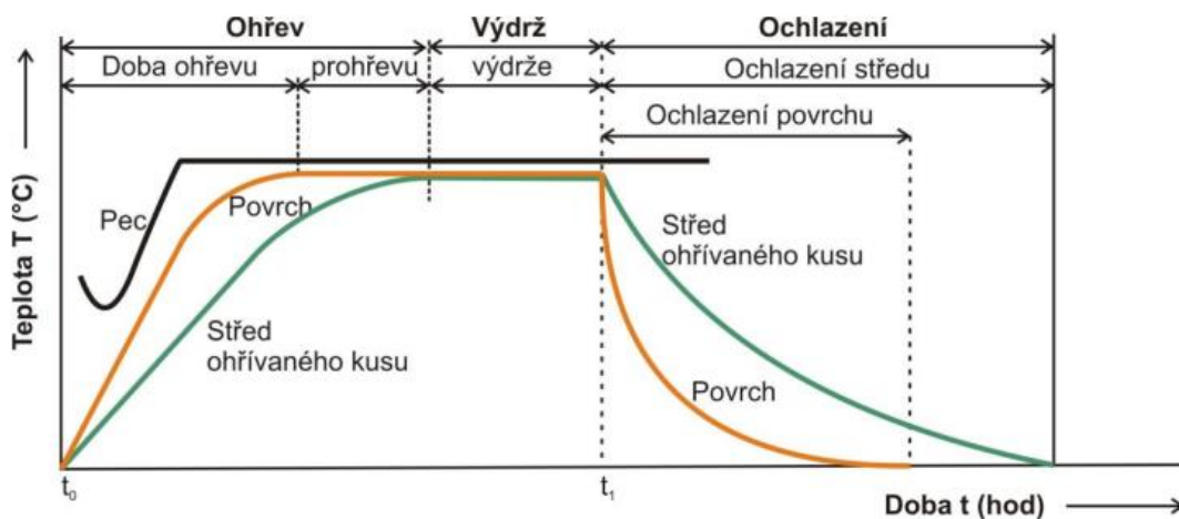
Obr. 13 Schematický popis zpevnování a etap rekrytalizačního žihání [15]
