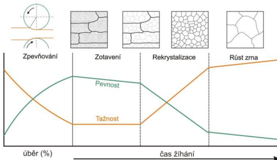
Obr. 15 Schematický popis zpevňování a etap rekrytalizačního žhání [15]
