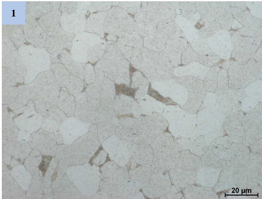
Obr. 27 Struktura drátu – válcovaný stav 1000x zvětšení
