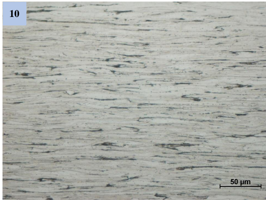
Obr. 29 Struktura drátu – Tepelně zpracován Pb 560 °C 60 m/min 500x zvětšení
