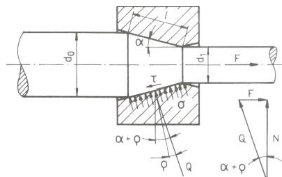
Obr. 2 Rovnováha sil v otvoru průvlatku podle E.Siebela [3]
