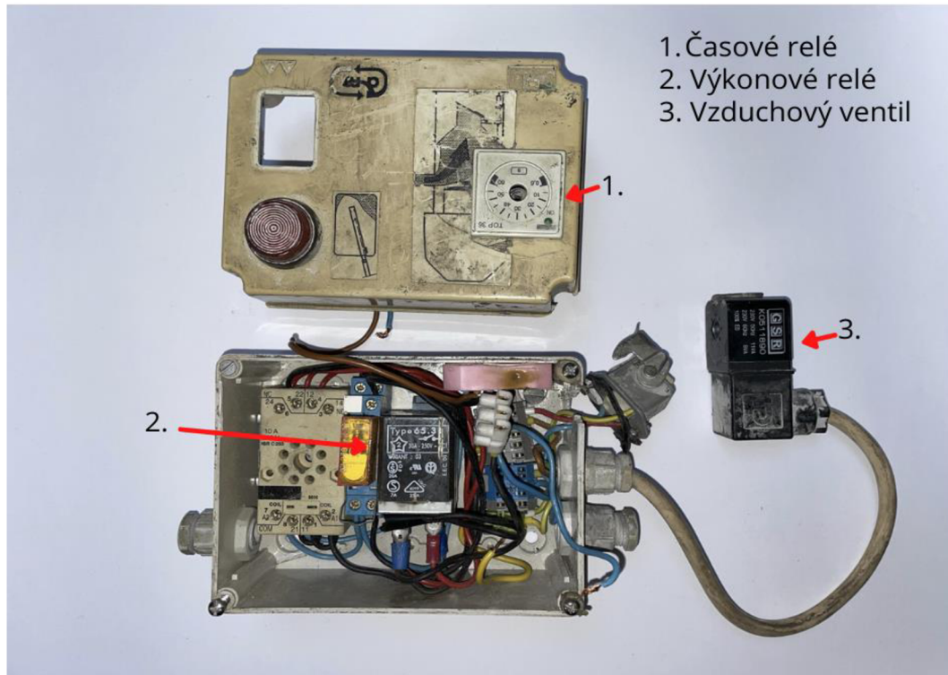
Obrázok 2.3: Pôvodné riešenie riadiaceho systému
