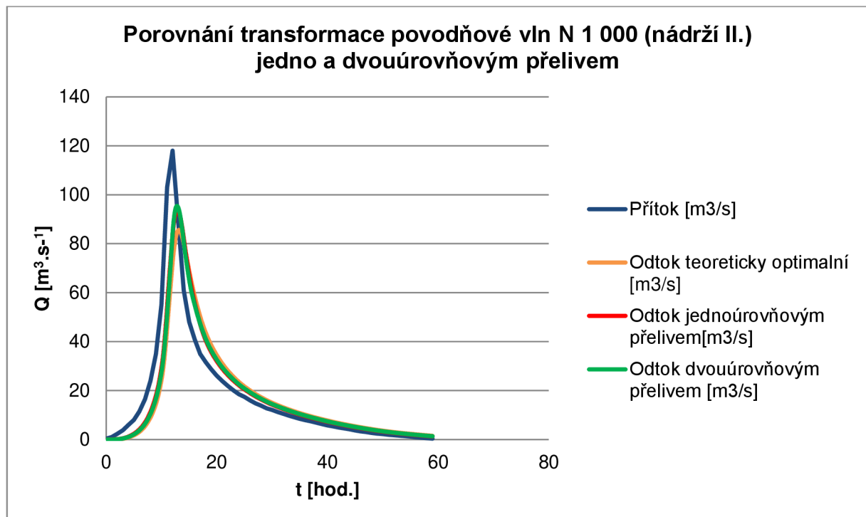
Obr. 68 Porovnání transformace povodňové vln N1 000 (nádrží II.)
