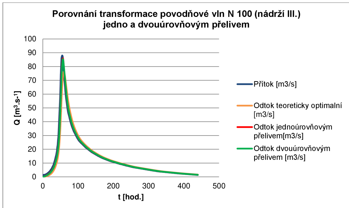
Obr. 75 Porovnání transformace povodňové vln N100 (nádrží III.)
