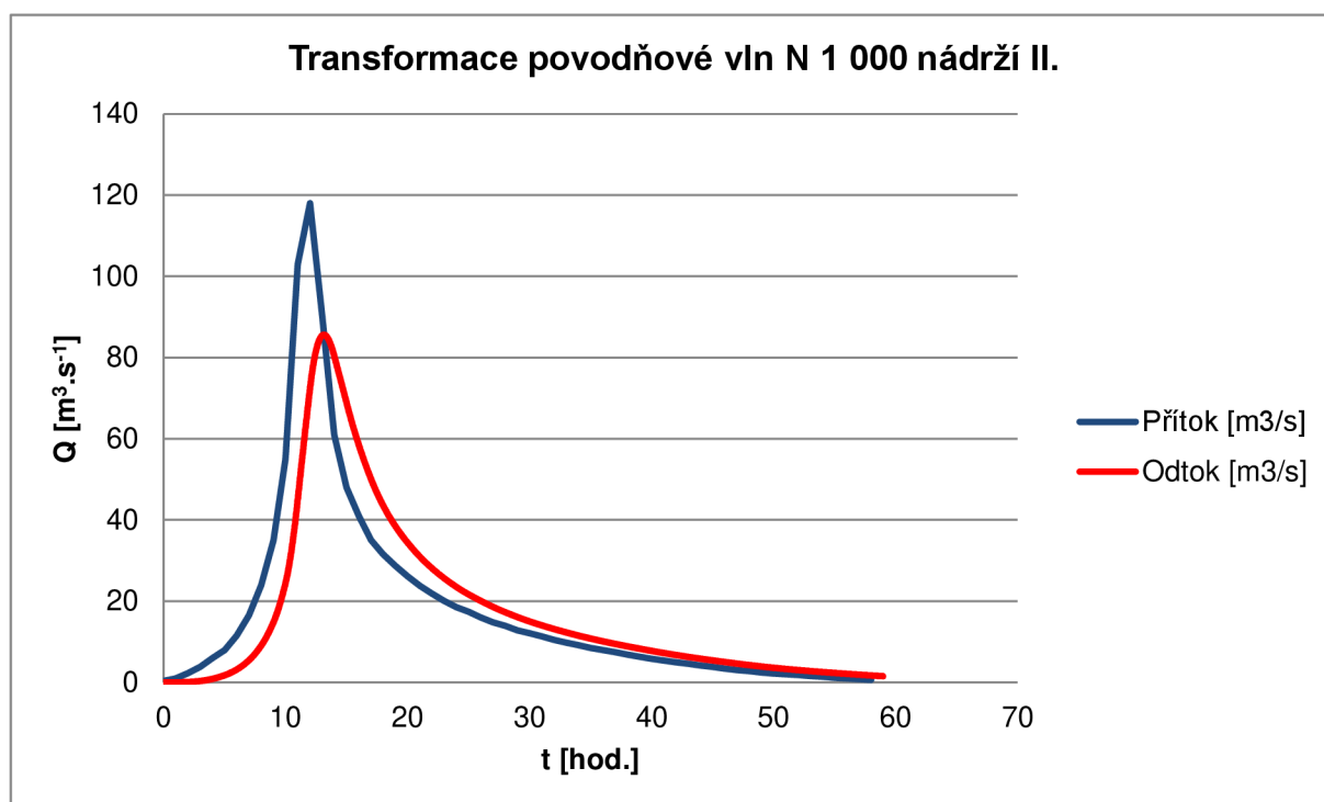
Obr. 27 Transformace povodňové vln N 1 000 nádrží II.
