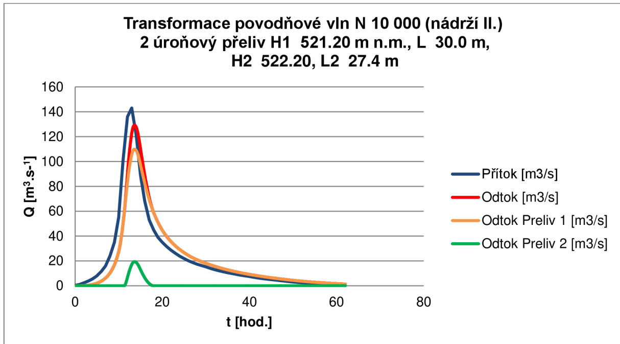
Obr. 51 Transformace povodňové vln N 10 000 (nádrží II.)
