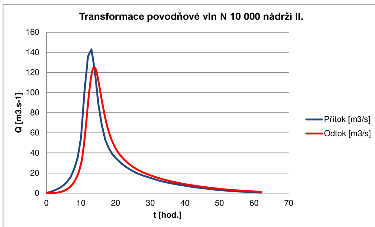
Obr. 26 Transformace povodňové vln N 10 000 nádrží II.
