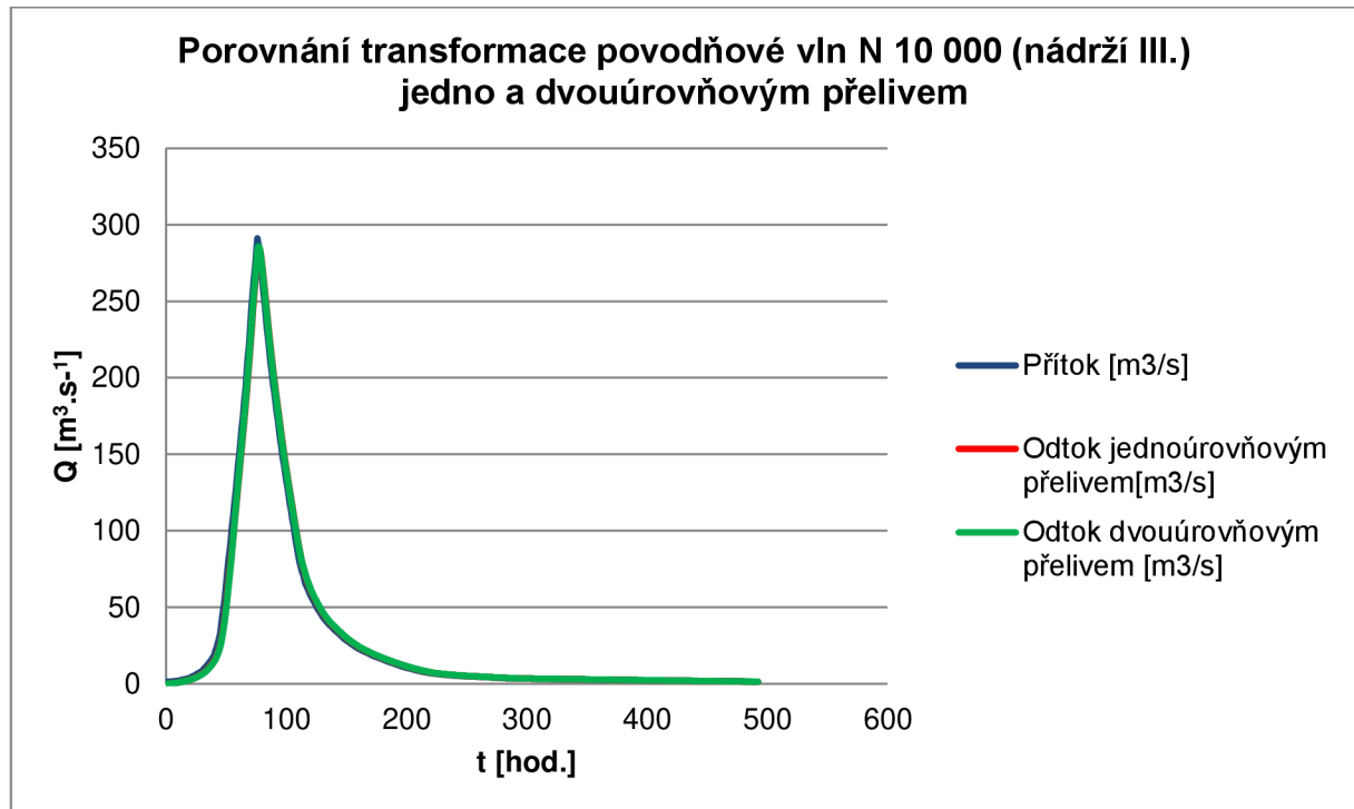
Obr. 72 Porovnání transformace povodňové vln N10 000 (nádrž III.)
