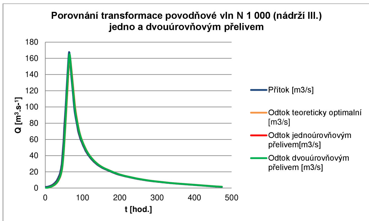
Obr. 73 Porovnání transformace povodňové vln N1 000 (nádrž III.)
