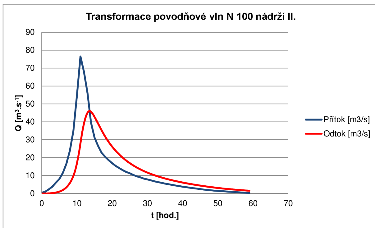
Obr. 28 Transformace povodňové vln N 100 nádrží II.
