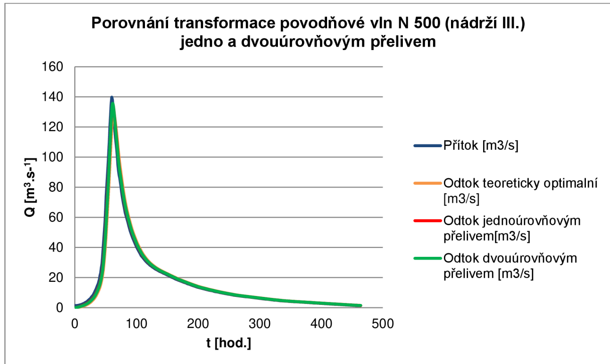
Obr. 74 Porovnání transformace povodňové vln N500 (nádrží III.)
