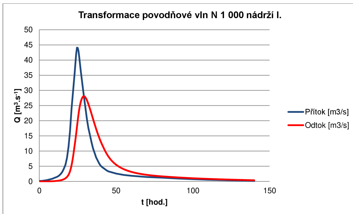
Obr. 22 Transformace povodňové vln N 1 000 nádrží I.
