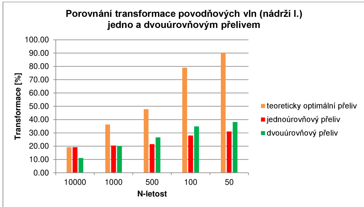
Obr. 60 Porovnání transformace povodňových vln (nádrž I.)
