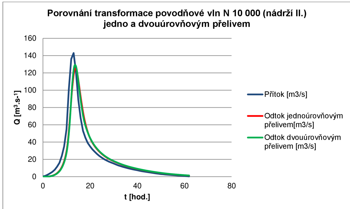
Obr. 67 Porovnání transformace povodňové vln N10 000 (nádrží II.)
