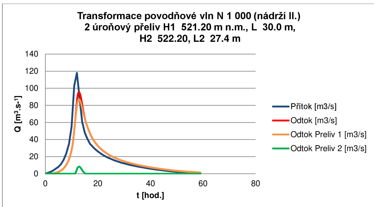
Obr. 52 Transformace povodňové vln N 1 000 (nádrží II.)
