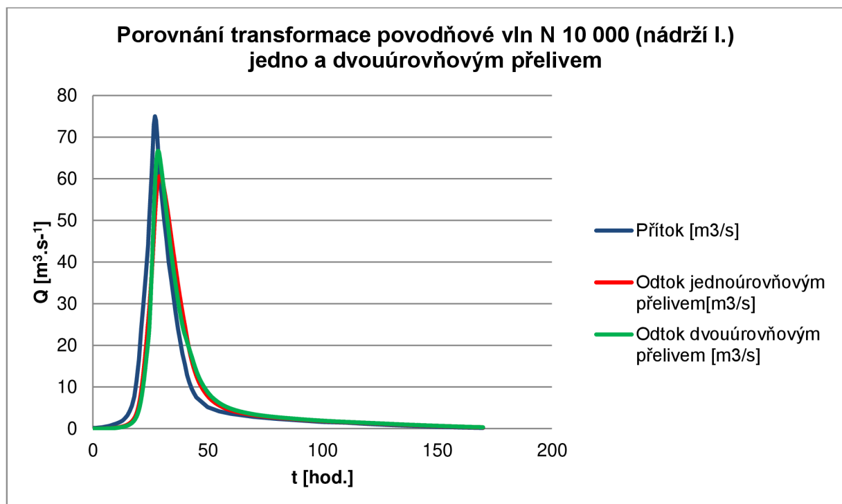
Obr. 61 Porovnání transformace povodňové vln N 10 000 (nádrž I.)
