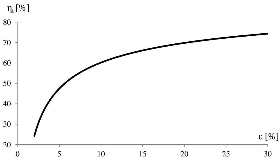
Obr. 5 Graf termické účinnosti Ottova cyklu v závislosti na kompresním poměru
