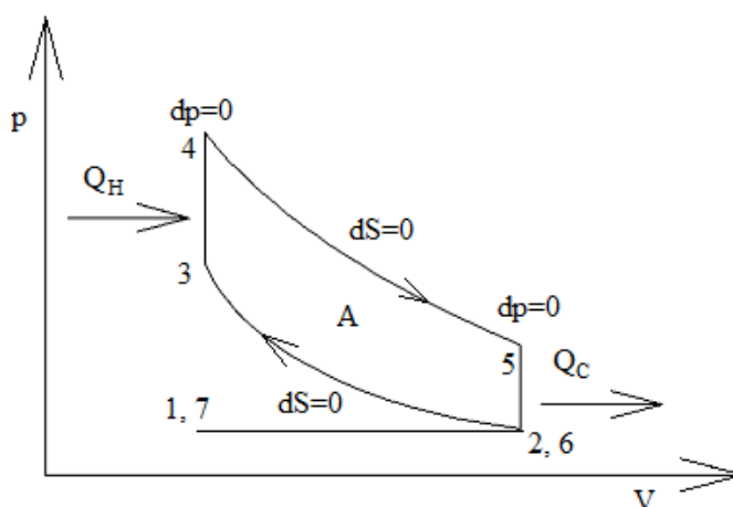
Obr. 4 Znázornění energetické bilance čtyřdobého Ottova cyklu v pV diagramu
