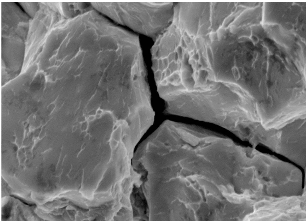
Obr. 10 Trhliny po hranicích zrn u vodíkovou korozí poškozeného materiálu (snímek pořízený elektronovým mikroskopem) [44]
