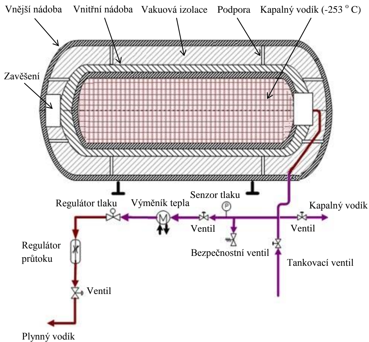
Obr. 16 Schéma kryogenní komory pro uskladnění vodíku v kapalně fázi [75], [76]
