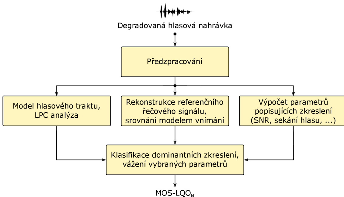
Obr. 1.7: Blokové schéma algoritmu P.563 (3SQM) [ 1 ]
