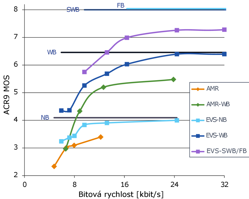
Obr. 3.12: Subjektivní hodnoty MOS čistých hl. vzorků kodeků AMR a EVS [ ]
