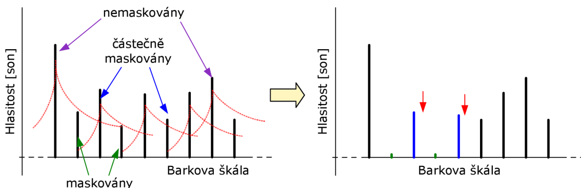
Obr. 1.6: Výpočet modifikovaných kritických pásem algoritmem POLQA [ ]
