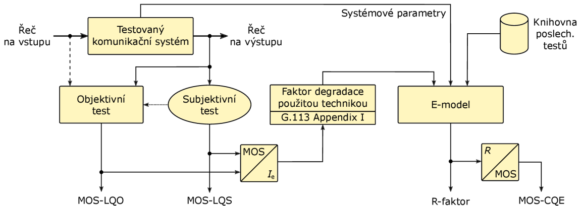
Obr. 2.5: Vztah E-modelu k dalším metodám testování kvality přenosu hlasu [ ]
