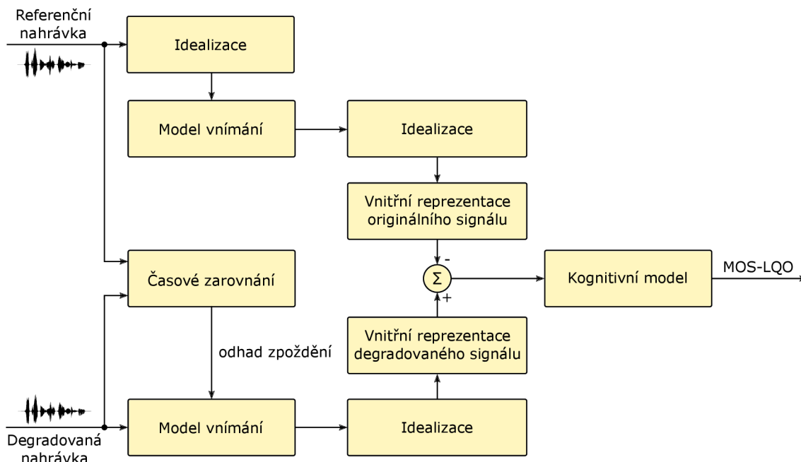
Obr. 1.3: Zjednodušené blokové schéma algoritmu POLQA [ 1 ]
