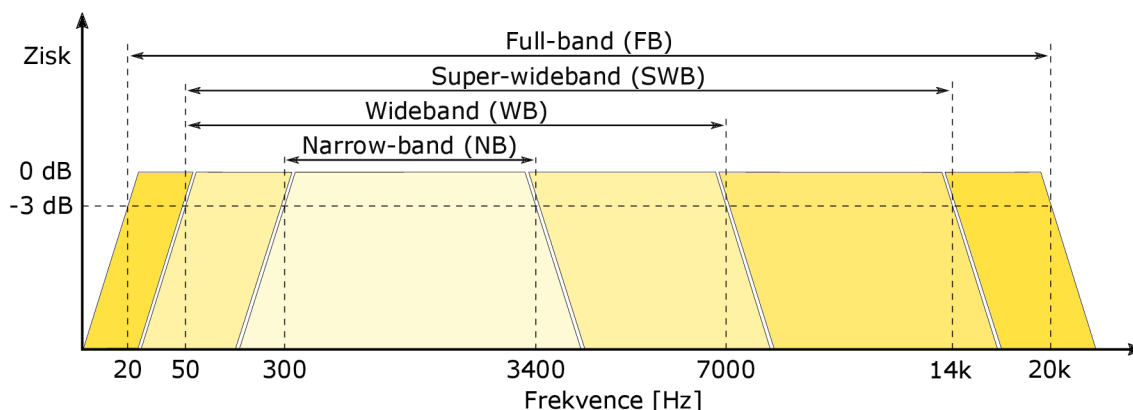
Obr. 3.8: Používané frekvenční šířky pásma hlasových kodeků
