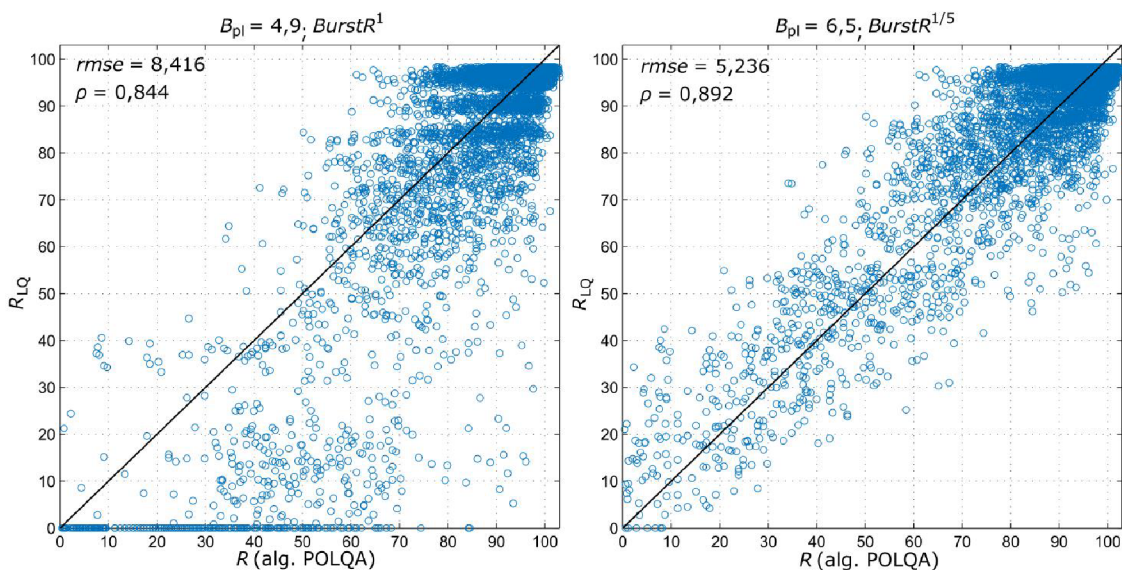
Obr. 4.18: Korelační diagramy R před a po optimalizaci parametrů
