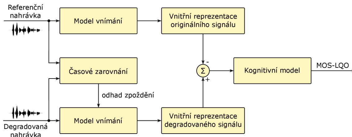
Obr. 1.2: Zjednodušené blokové schéma algoritmu PESQ [ 11 ]
