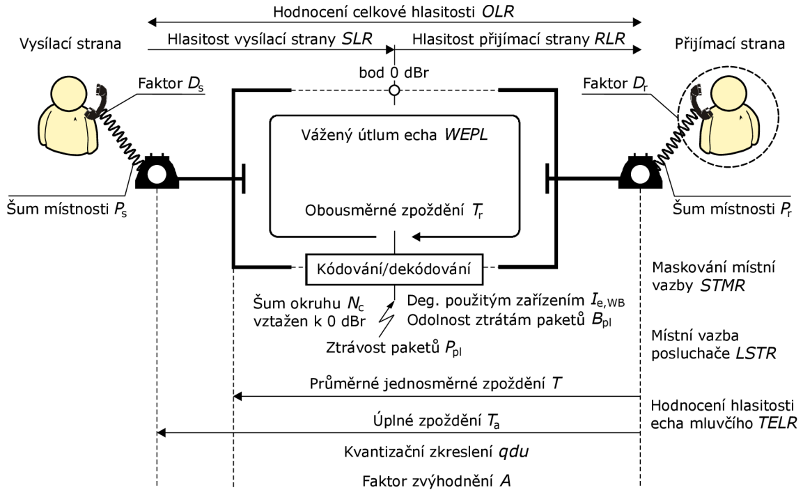
Obr. 2.1: Parametrický popis E-modelu [ 1 ]
