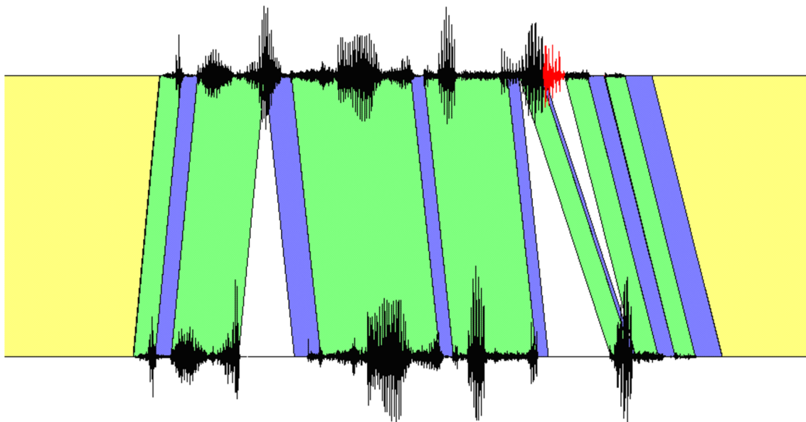
Obr. 1.5: Příklad zarovnání signálů algoritmem POLQA [ 1 ]
