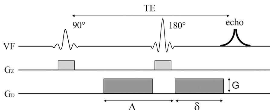
Obr. 1.1: Stejskal-Tannerova sekvence
