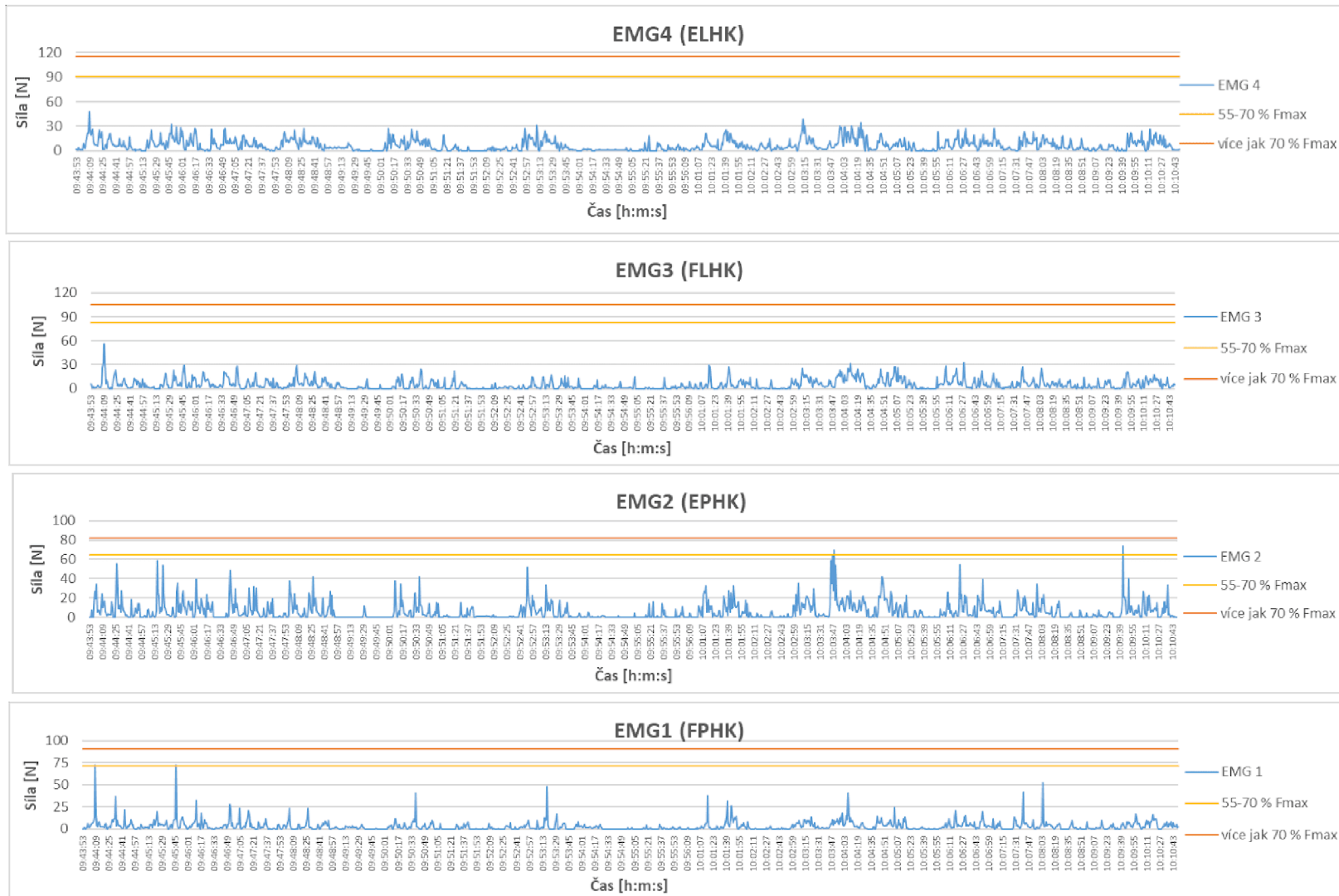
Obrázek č. 29: Graf průběhu svalových sil probanda M1, OP170
