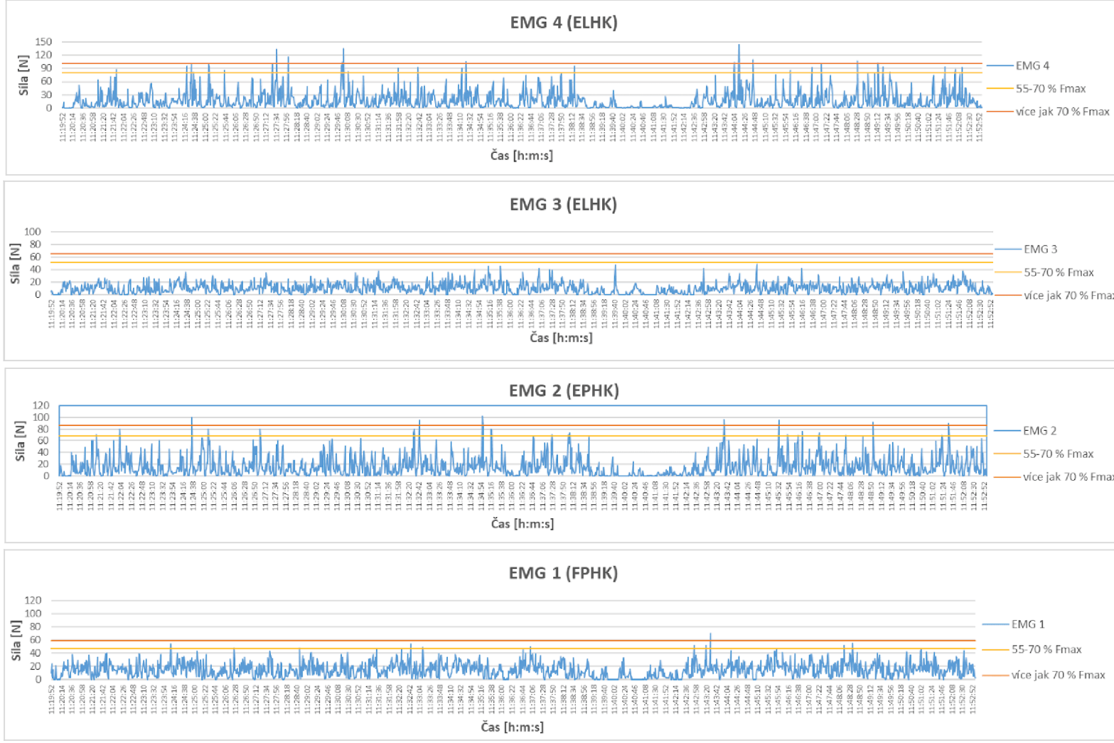
Obrázek č. 31: Graf průběhu svalových sil probanda M2, OP110
