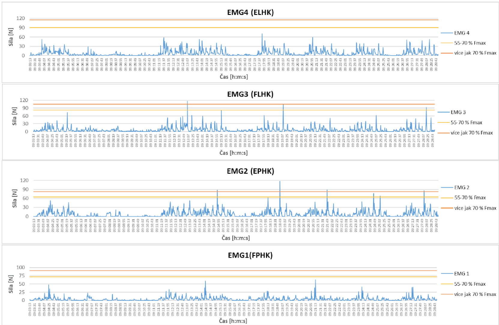
Obrázek č. 28: Grafické zpracování průběhu svalových sil probanda M1, OP160
