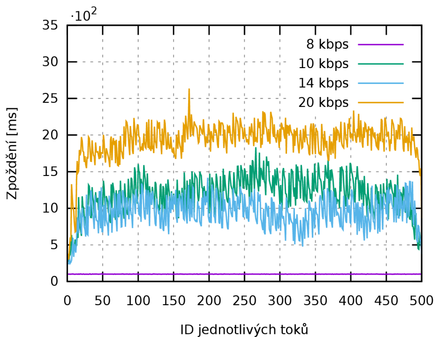
Obr. 6.7: Zpoždění upload - konfigurace LTE Cat-M1.
