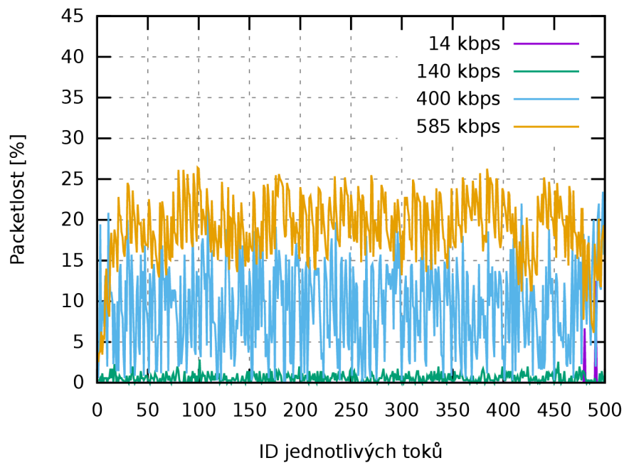
Obr. 6.4: Ztrátovost upload LTE/LTE-A – 500 UE, 1 eNB.
