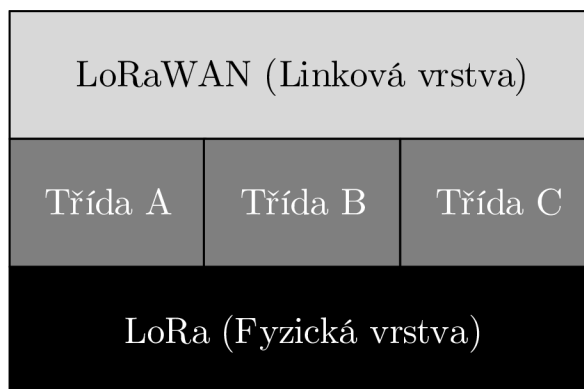
Obr. 3.2: Architektura protokolu LoRaWAN [30].
