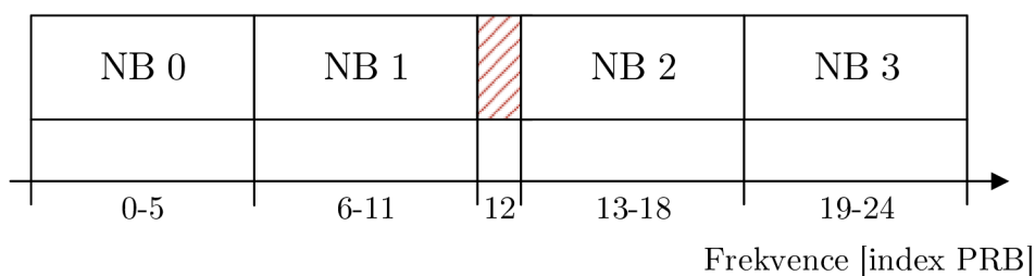
Obr. 2.6: Příklad systému LTE o šířce frekvenčního pásma 5 MHz [1].
