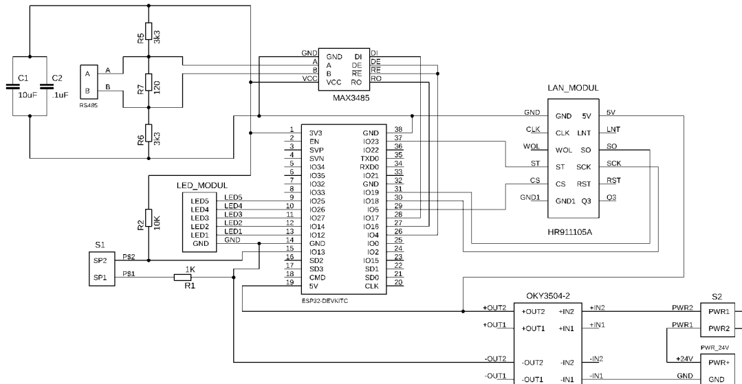
Obr. 6-6 Schéma zapojenia
