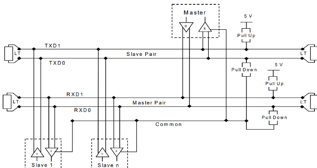
Obr. 1-A Štvorvodičové zapojenie.
