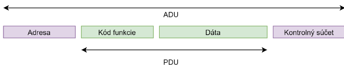
Obr. 2-2 Základná štruktúra MODBUS rámca. [1]
