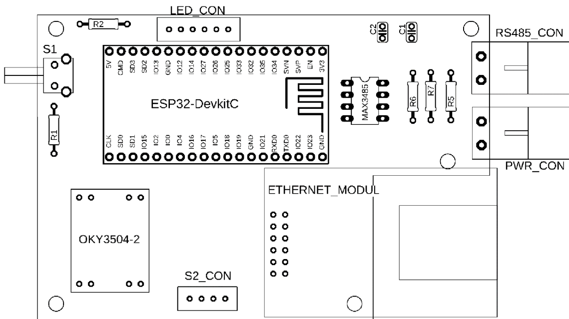
Obr. 6-8 DPS z pohľadu súčiastok
