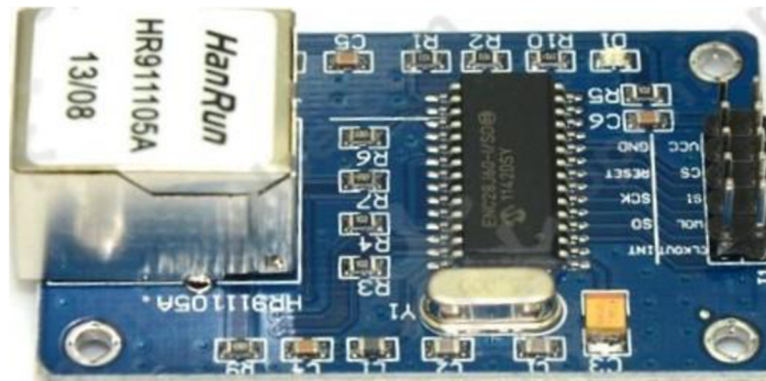
Obr. 6-3 Ethernetový modul s obvodom ENC28J60.
