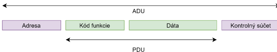
Obr. 3-1 Rámec ADU MODBUS SERIAL LINE. [4]
