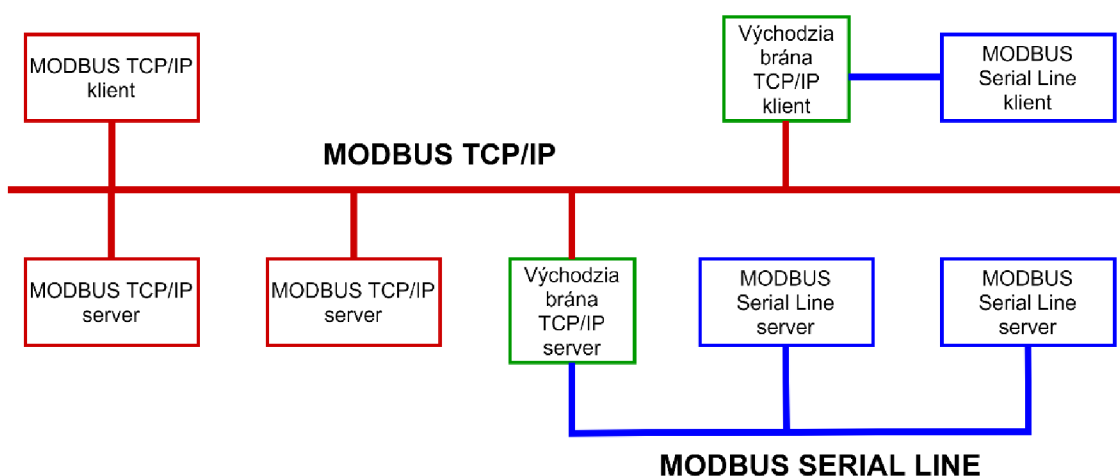
Obr. 4-2 Spôsob pripájania zariadení k MODBUS TCP/IP. [7]
