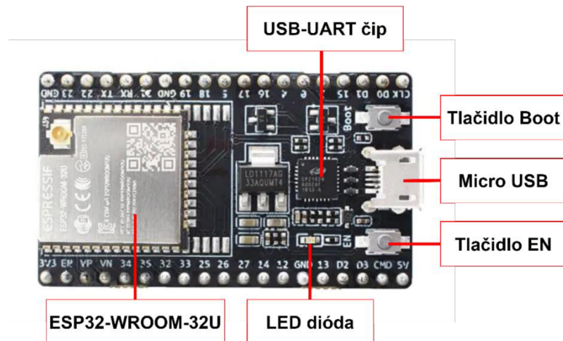
Obr. 5-2 Vývojový kit ESP32-DevKitC-32U
