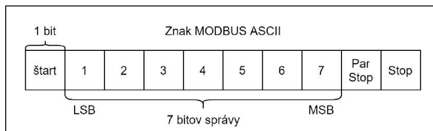
Obr. 3-3 Sekvencia bitov, znaku MODBUS ASCII [4]
