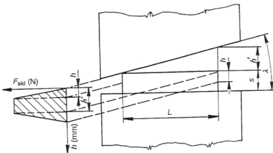
Obr. 10 Stříhání skloněnými břity [19]
