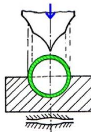
Obr. 23 Princip stříhu trubek [6]
