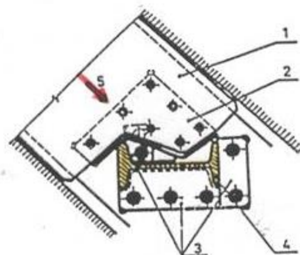
Obr. 22 Nože na stříhání profilů [6]
