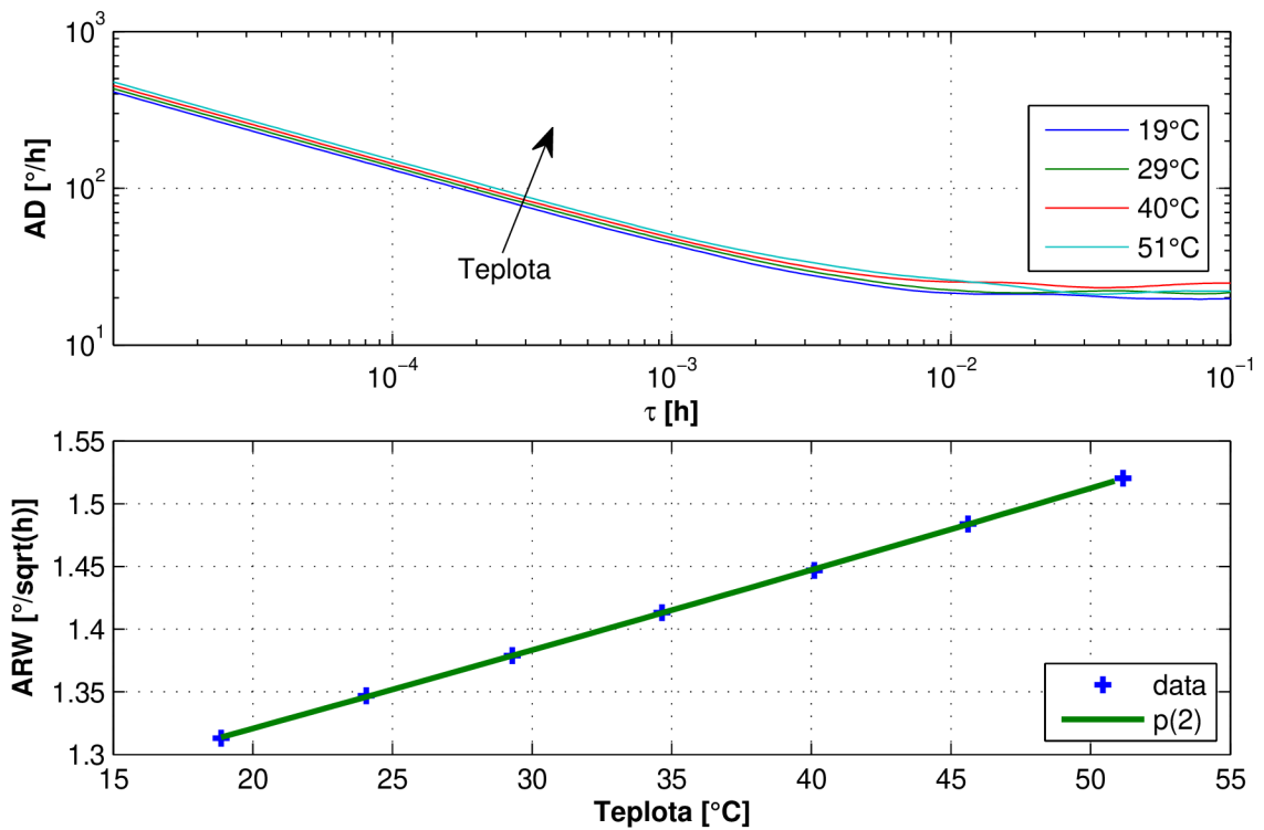
Obr. A.42: Závislost ARW na teplotě (ADXRS642 #1)
