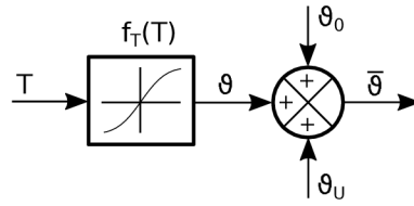
Obr. 6.13: Model teplotního snímače MEMS gyroskopu
