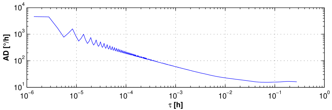
Obr. 5.12: Allanova odchylka - rušení z napájecího zdroje
