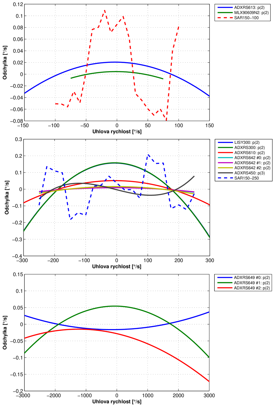
Obr. 6.5: Aproximace chyby linearity MEMS gyroskopů
