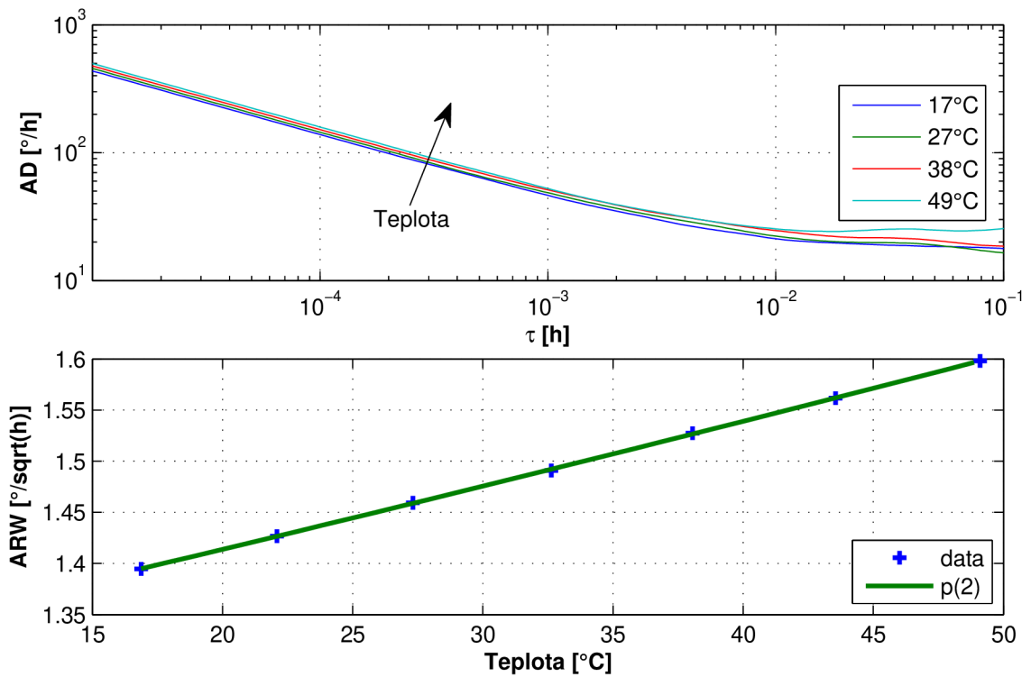
Obr. A.41: Závislost ARW na teplotě (ADXRS642 #0)
