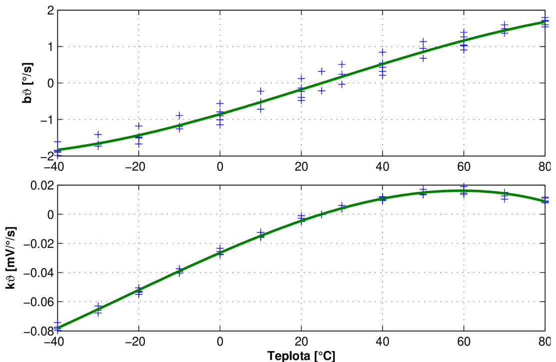
Obr. 6.6: Opakovatelnost parametrů ADXRS610 při cyklování teploty
