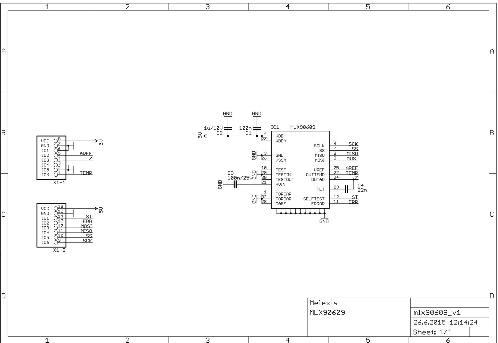
Obr. D.6: Schéma univerzální DPS pro gyroskopy Melexis (MLX90609)
