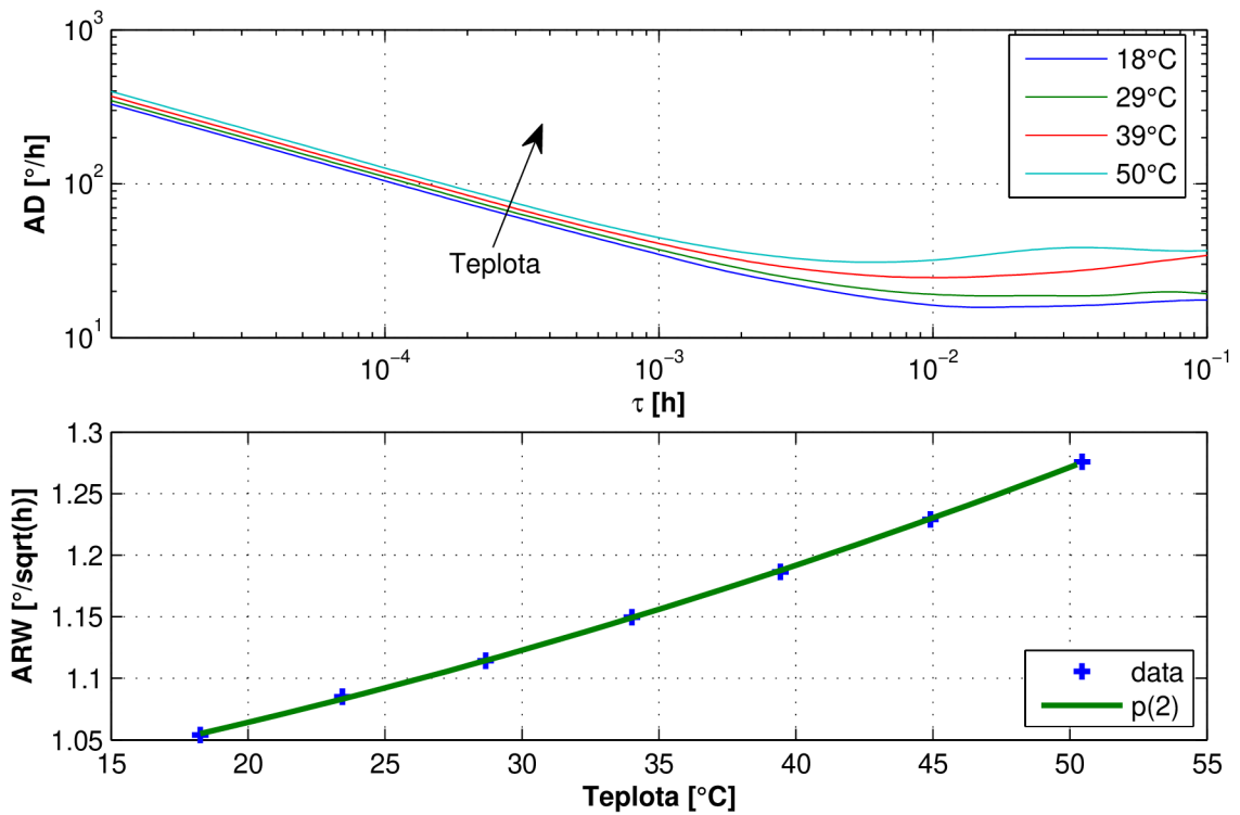
Obr. A.43: Závislost ARW na teplotě (ADXRS642 #2)
