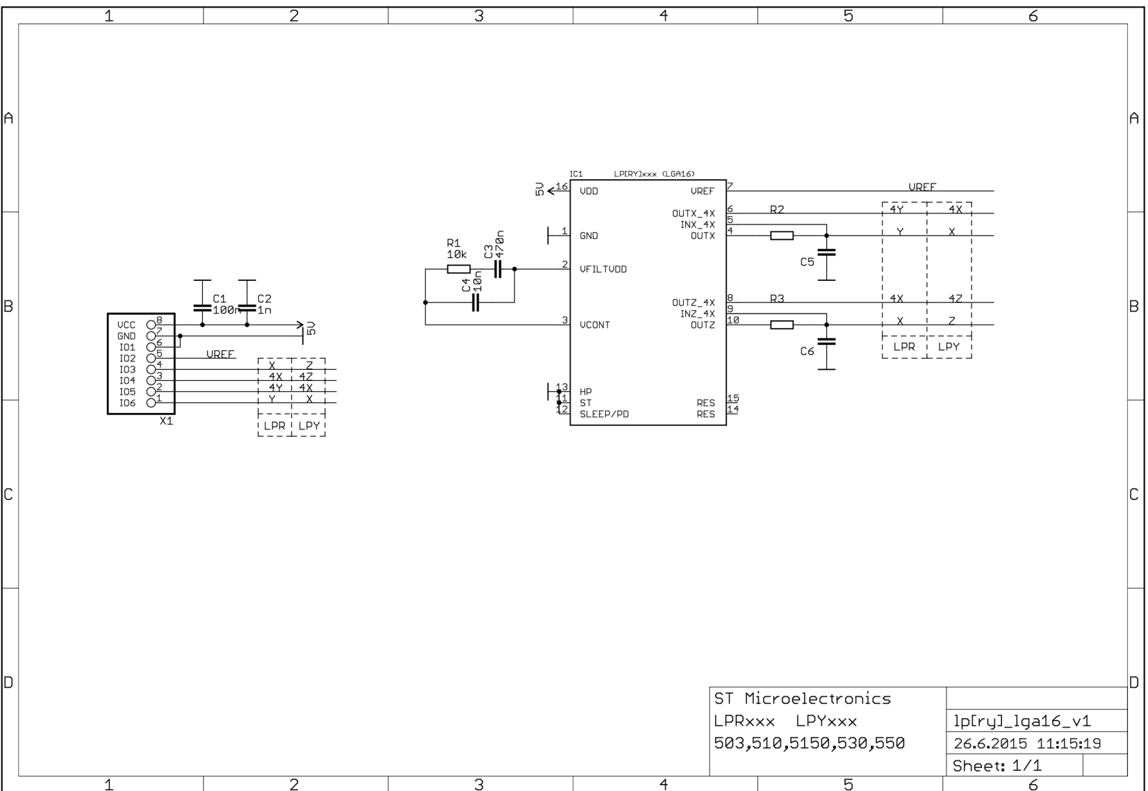
Obr. D.8: Schéma univerzální DPS pro gyroskopy ST Microelectronics (LGA16)
