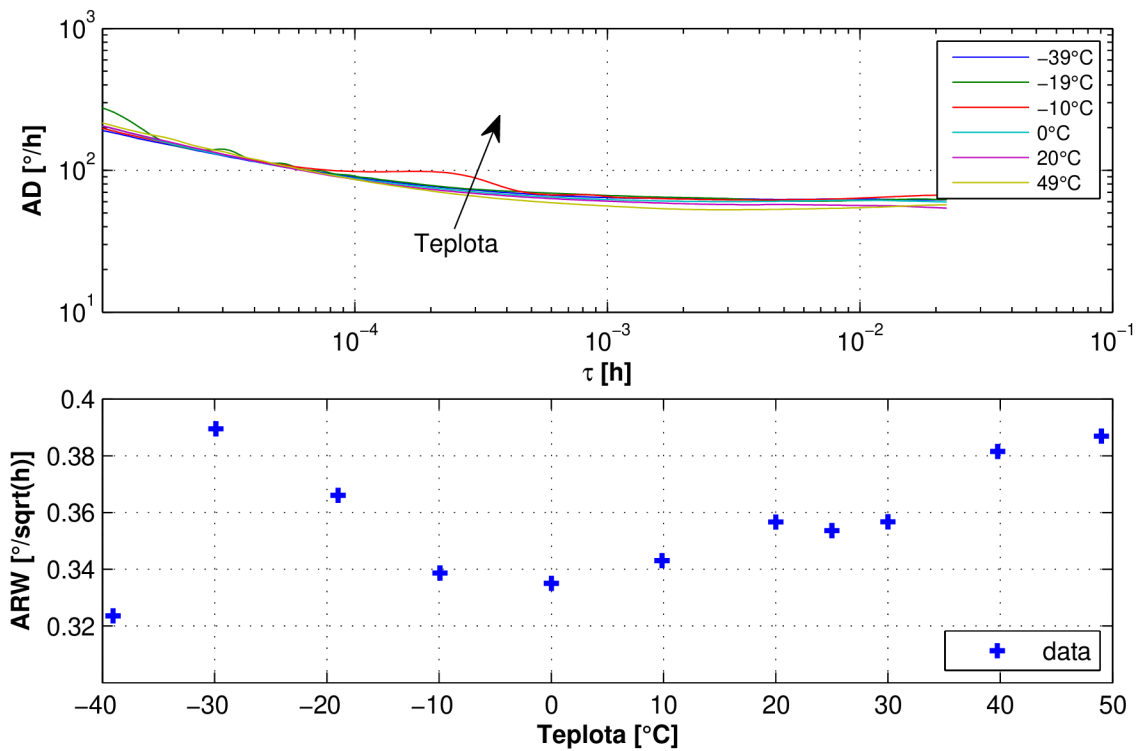
Obr. A.44: Závislost ARW na teplotě (SAR150-100)
