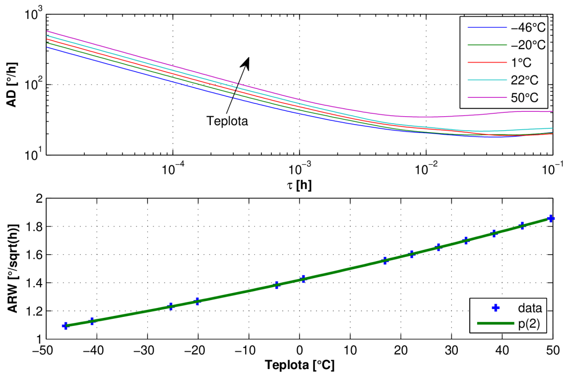
Obr. A.40: Závislost ARW na teplotě (ADXRS613)
