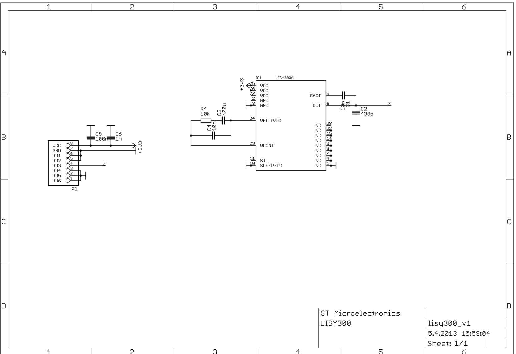
Obr. D.10: Schéma univerzální DPS pro gyroskopy ST Microelectronics (LISY300)
