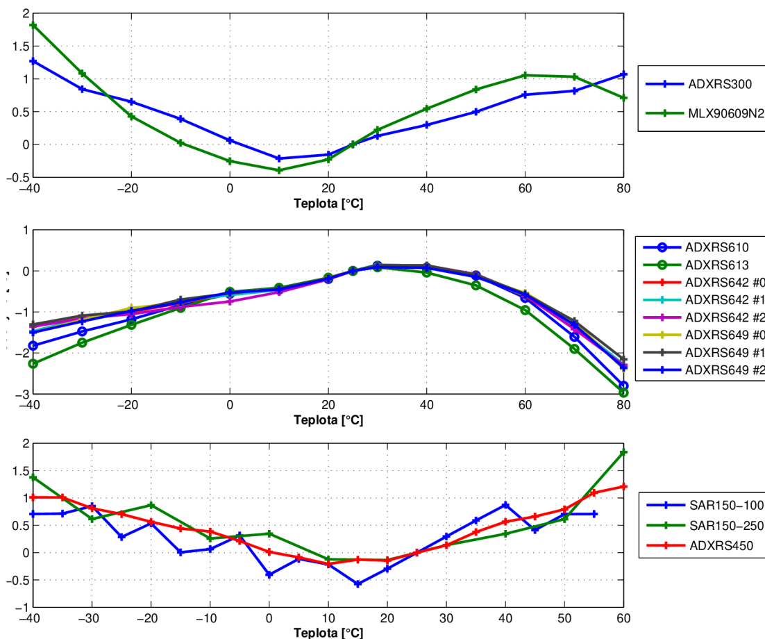
Obr. 6.1: Nelinearita snímače teploty v MEMS gyroskopech
