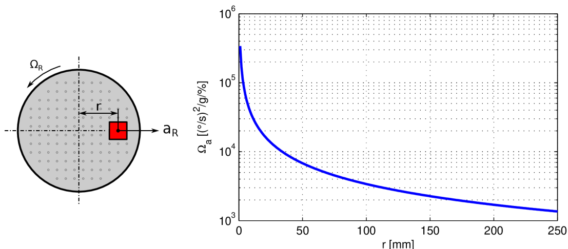
Obr. 5.22: Vliv umístění gyroskopu na RS
