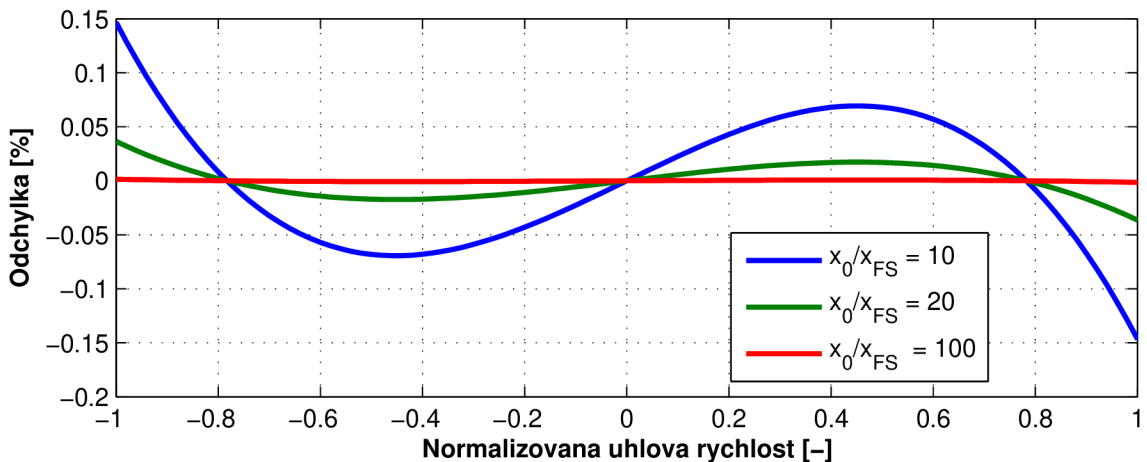
Obr. 6.4: Nelinearita způsobená snímacím kondenzátorem
