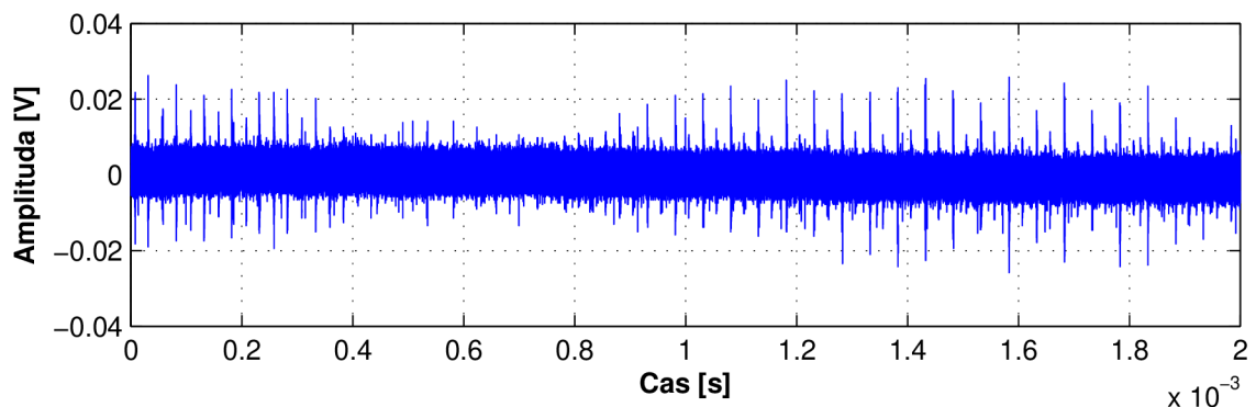
Obr. 5.5: Rušení signálů na rotačním konektoru SDL1401 (jehlové impulzy)
