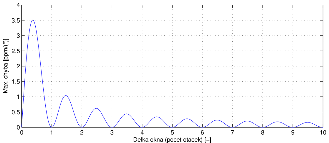
Obr. 5.15: Maximální chyba vlivem kývání osy
