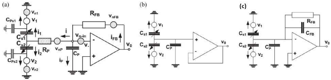
Obr. 2.7: Zesilovače pro kapacitní snímače [33]
