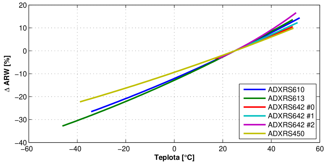
Obr. 6.10: Relativní změna ARW v závislosti na teplotě
