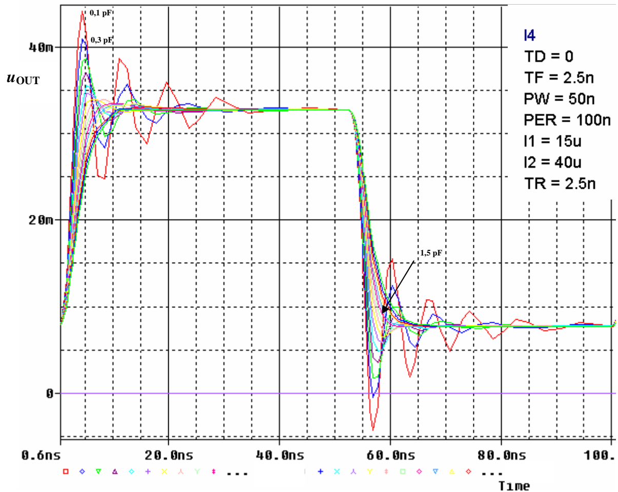
Obr.: 7-12 Oscilace výstupního napětí, vstupní proud s frekvencí 10 MHz
