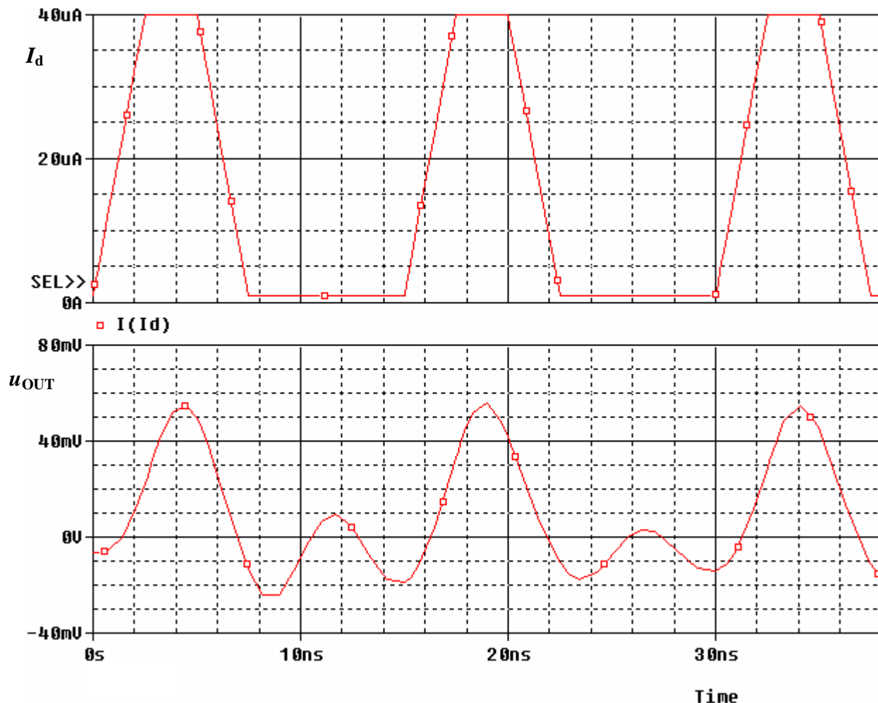
Obr.: 7-11 Průběh proudu I_d a výstupního napětí OZ
