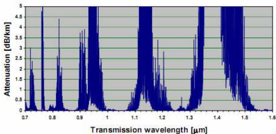
Obr.: 2-2 Závislost útlumu Mieovým rozptylem na vlnové délce, převzato z [9].
