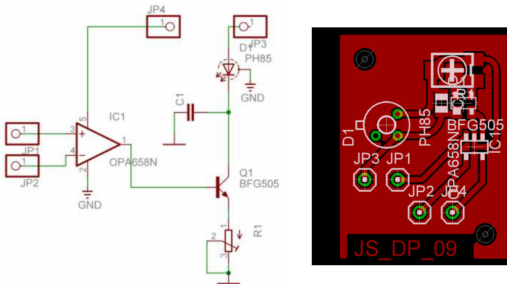
Obr C-1 Schéma zapojení budiče laseru pro praktickou realizaci
