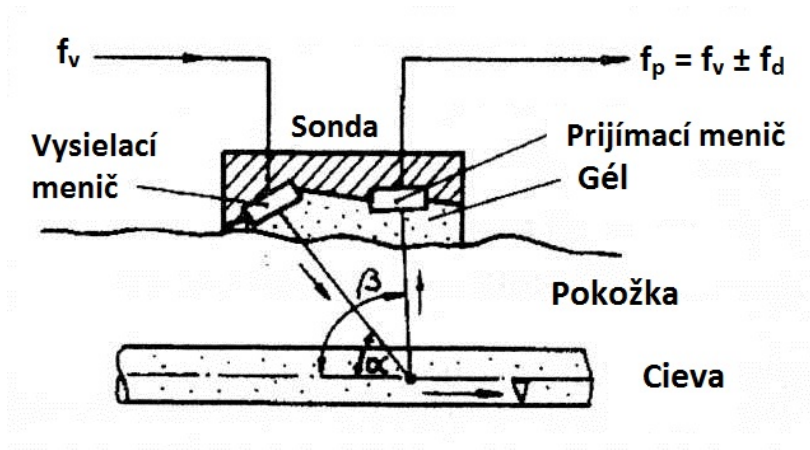
Obr. 8 Dopplerov efekt [17].
