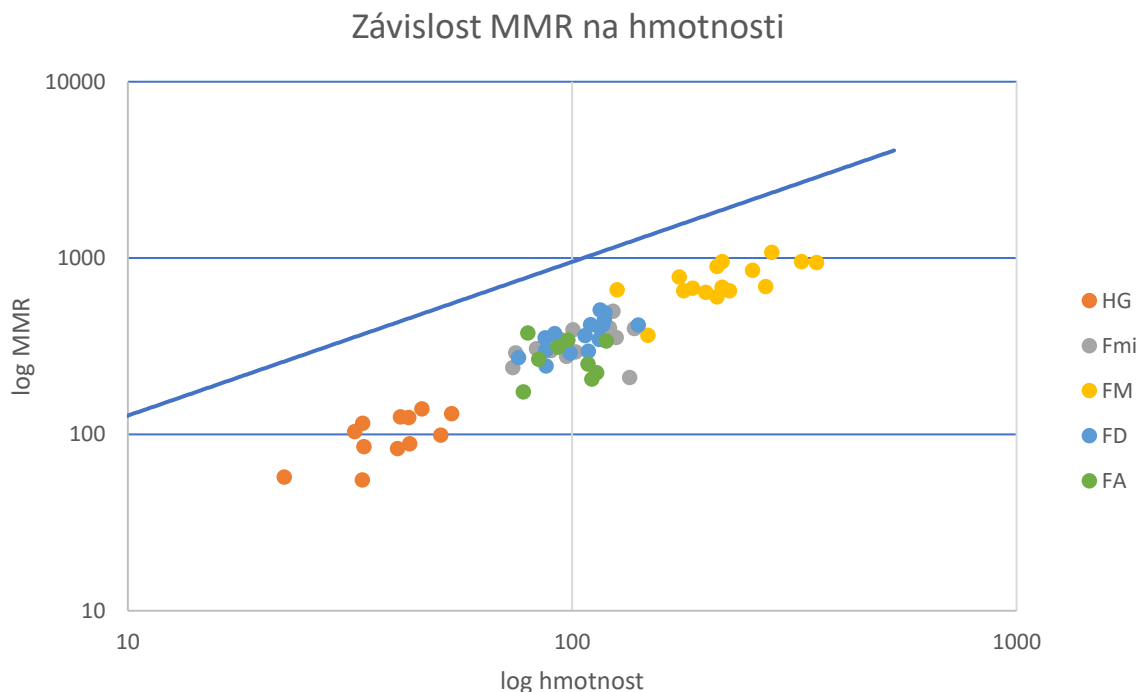
Obr. 5: Ověření alometrické závislosti logaritmičkových hodnot maximálního metabolismu na logaritmičkových hodnotách hmotnosti. Graf je proložen přímkou regrese škálování VO_{2max} ( VO_{2MAX}=118,2 * Mb^{0,872} ; R^2 = 0,9653 ; Weibel et al. 2004). (Fa- Fukomys anelli , Fd- Fukomys darlingi , Fm- Fukomys mechowii , Fmi- Fukomys micklei , Hg- Heterocephalus glaber ; přímká-regresivní přímká).
