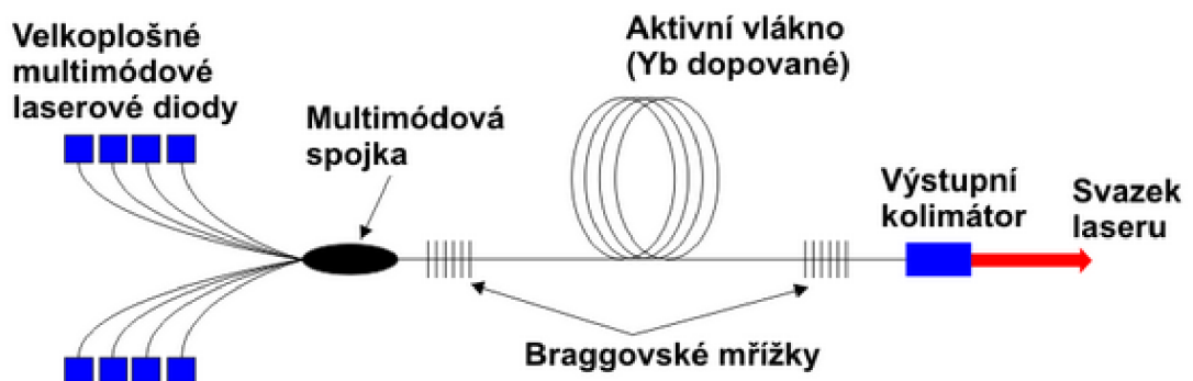
Obr. 11 Princip vláknového laseru [16].
