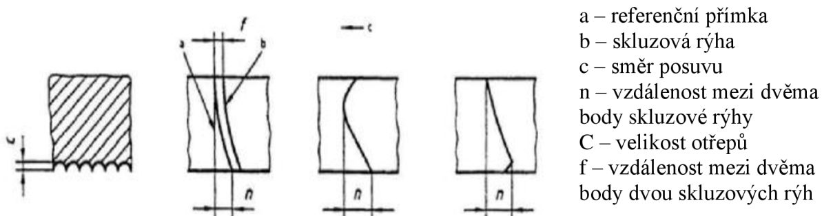
Obr. 27 Skluzová rýha [17].
