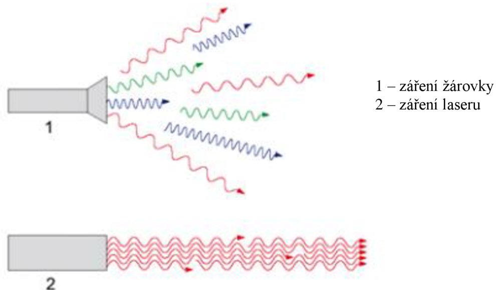
Obr. 6 Typy záření [35].
