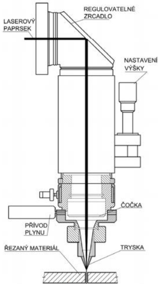
Obr. 22 Řezací hlavice [9].
