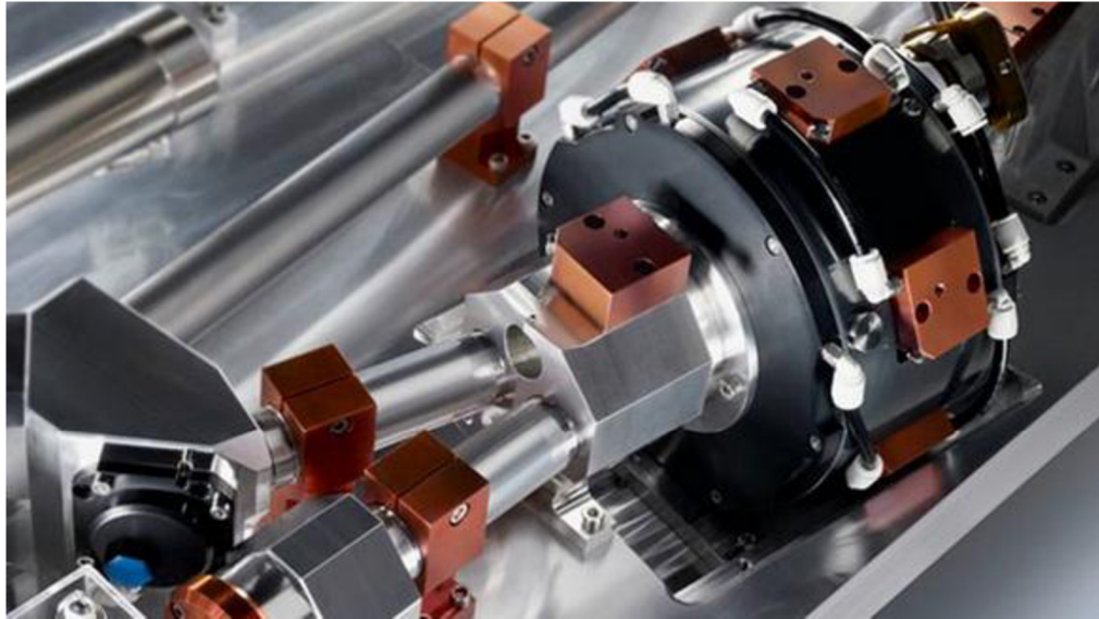
Obr. 10 Diskový laser [16].
