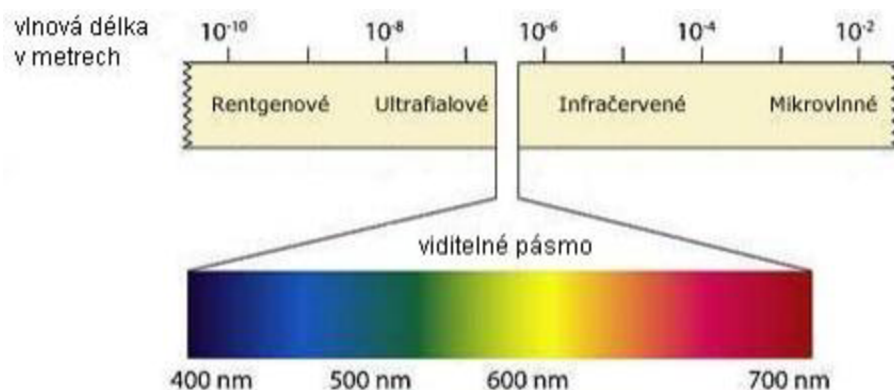
Obr. 7 Světelné spektrum [39].
