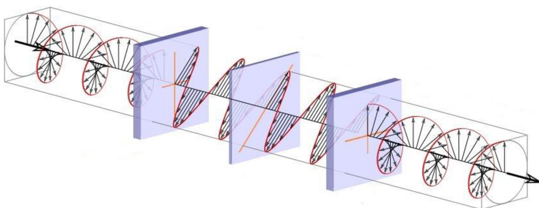
Obr. 8 Polarizace světla [19].
