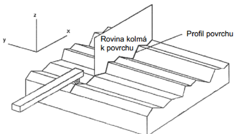
Obr. 29 Profil povrchu [25].
