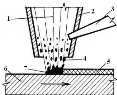
Obr. 21 Princip povlakování [28].
