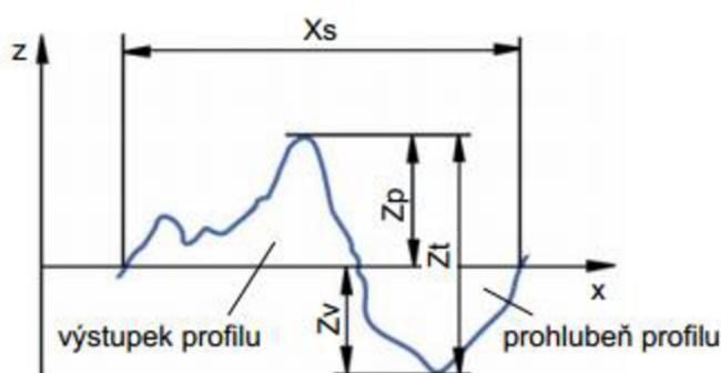
Obr. 30 Prvek profilu [25].
