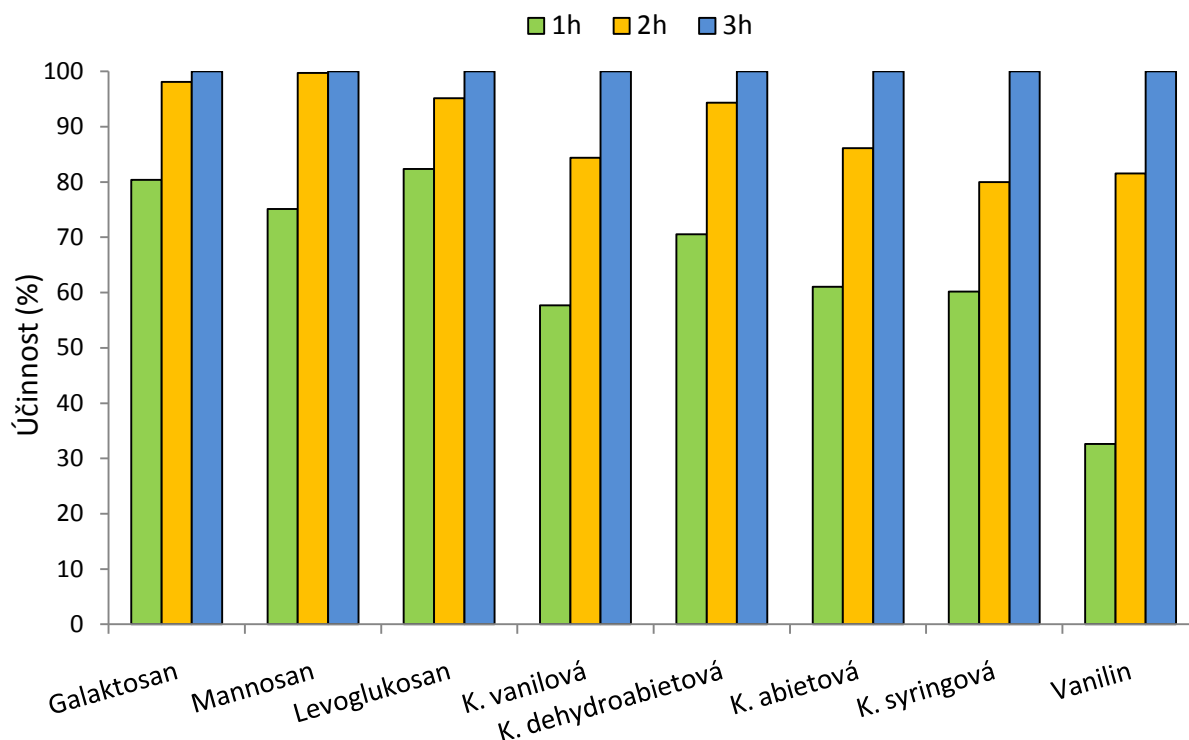
Graf č. 5.7: Závislost účinnosti derivatizace směsí MSTFA na čase derivatizace pro anhydridy monosacharidů a markery spalování dřeva (reálný vzorek)
