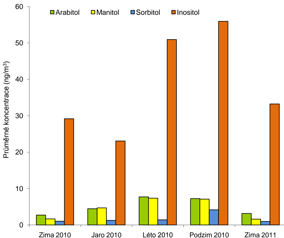
Graf č. 5.27: Průměrné hodnoty koncentrace alditolů v aerosolu PM 2,5
