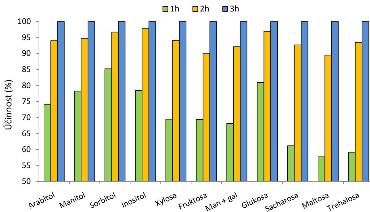
Graf č. 5.7: Závislost účinnosti derivatizace směsí MSTFA na čase derivatizace pro anhydridy monosacharidů a markery spalování dřeva (reálný vzorek)
