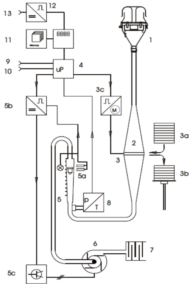
Obr. č. 4.2: Schéma vzorkovače DIGITEL HVS DHA-80. (1) PM separátor, (2) průtoková komora, (3) filtr, (3a) zásobník čistých filtrů, (3b) odběr použitých filtrů, (3c) elektronické zařízení pro automatickou výměnu filtrů, (4) mikroprocesorová kontrola, (5) průtokoměr, (5a) fotosenzor snímající průtok vzduchu, (5b, 5c) kontrolní elektronika, (6) čerpadlo pro nasávání vzduchu, (7) tlumič hluku, (8) měřicí jednotka tlaku a teploty, (9) výstup pro tisk, (10) rozhraní RS232 C, (11) slot pro PC kartu, (12,13) vstup pro senzor rychlosti a směru větru (11, 12, 13) jsou volitelné.
