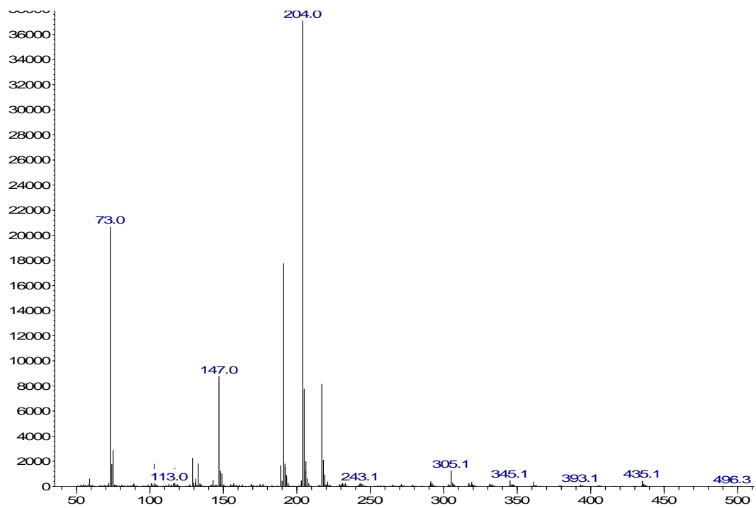
Příloha č. 9.1.3: Hmotnostní spektrum glukosy (monosacharid)
