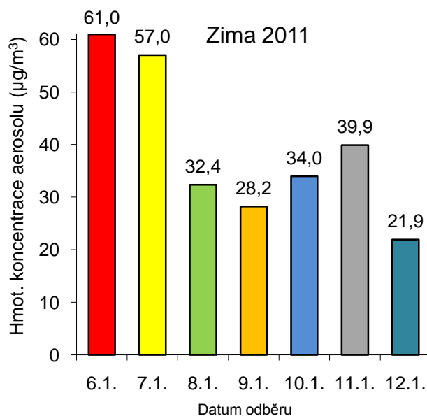
Grafy č. 5.19-5.23: Množství odebraného aerosolu frakce PM 2,5 pro jednotlivá období a dny
