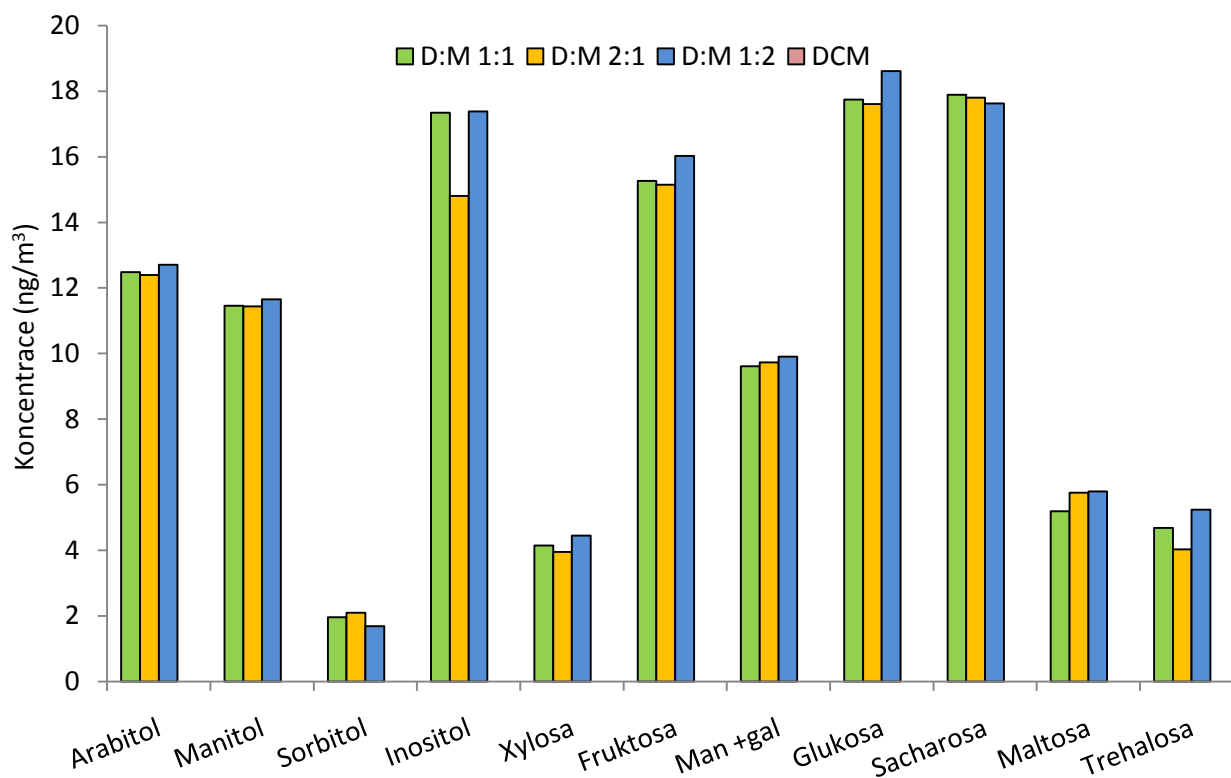
Graf č. 5.18: Porovnání účinnosti rozpouštědel pro sacharidy
