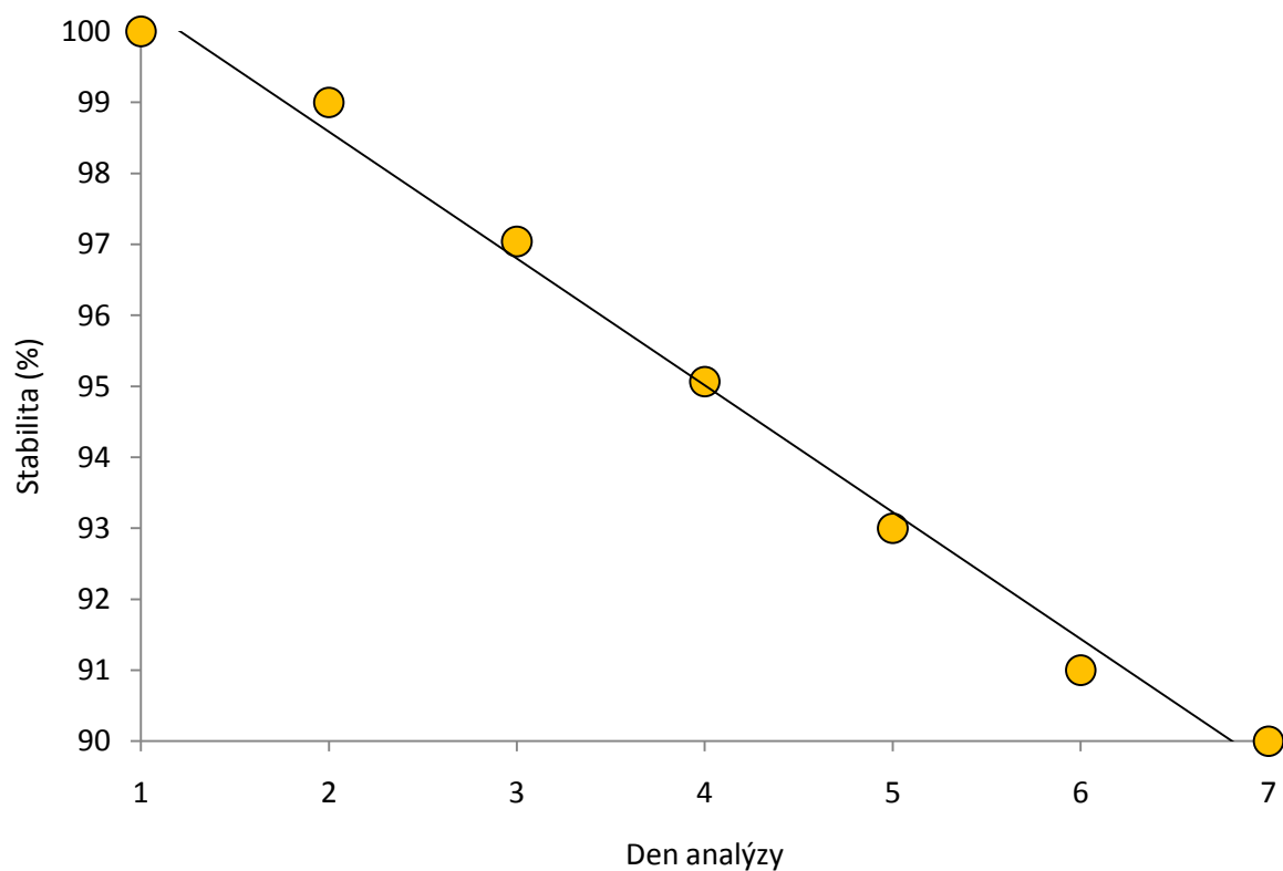
Graf č. 5.16: Zobrazení stability levoglukosanu po derivatizaci směsí MSTFA+1 % TMCS
