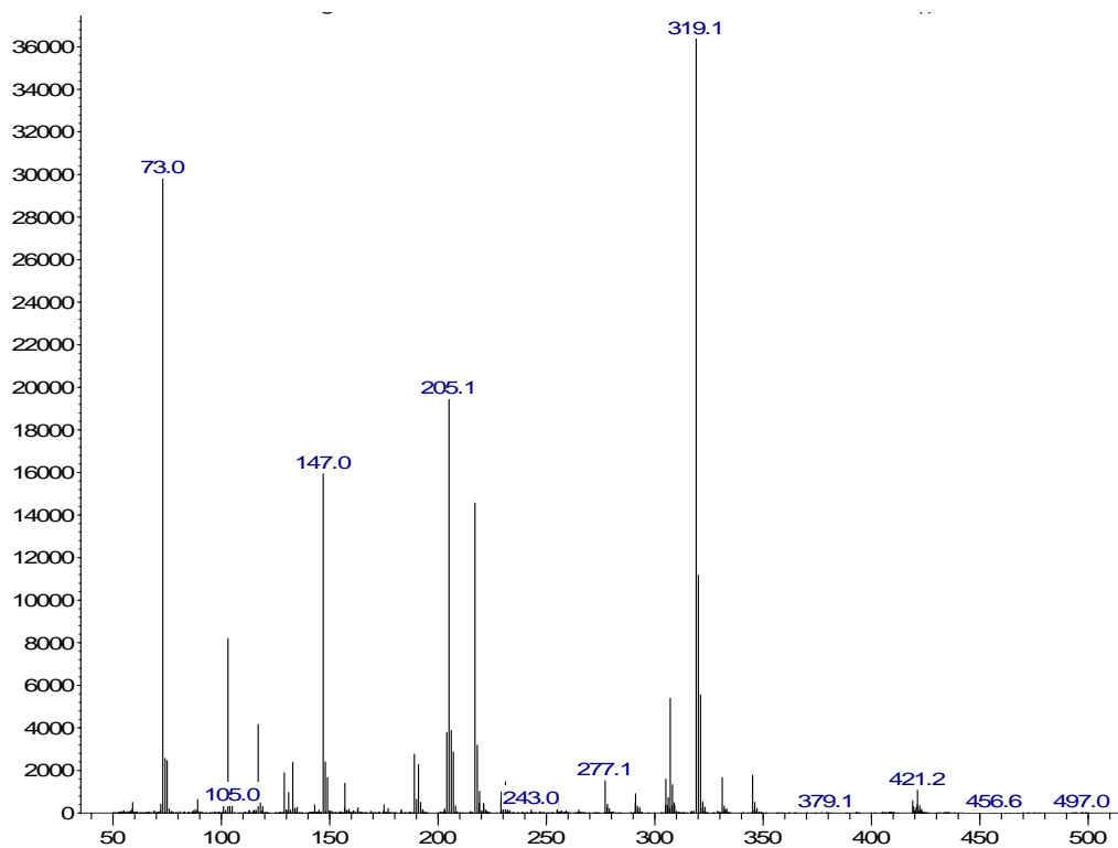
Příloha č. 9.1.4: Hmotnostní spektrum manitolu (alditol)
