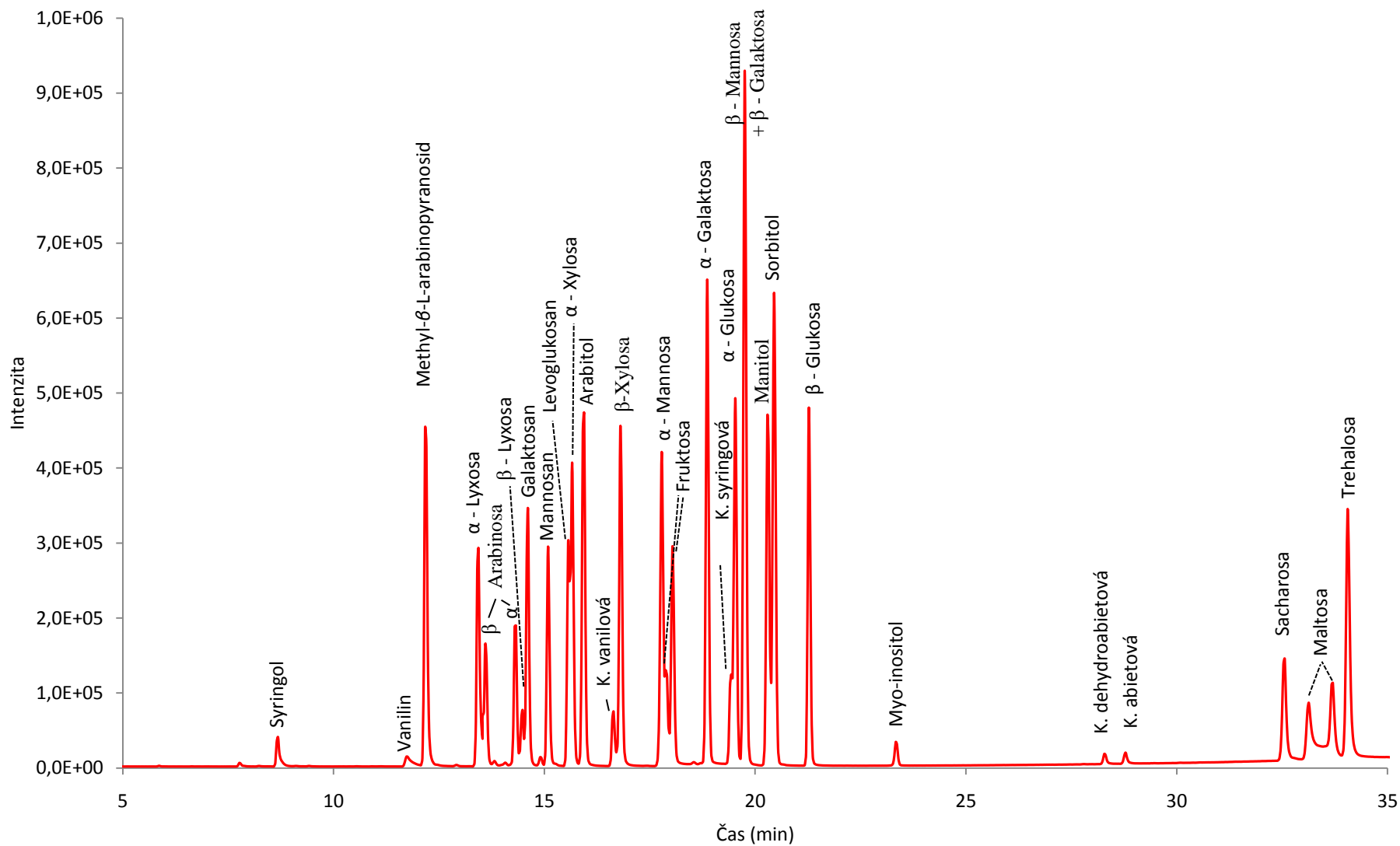
Příloha č. 9.2.1: Chromatogram směsi standardů o koncentraci 5 \mu g/ml
