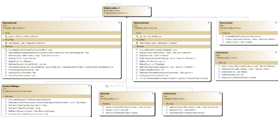
Obrázek 13: Diagram tříd služeb entit vyděděných z EntityServiceBase
