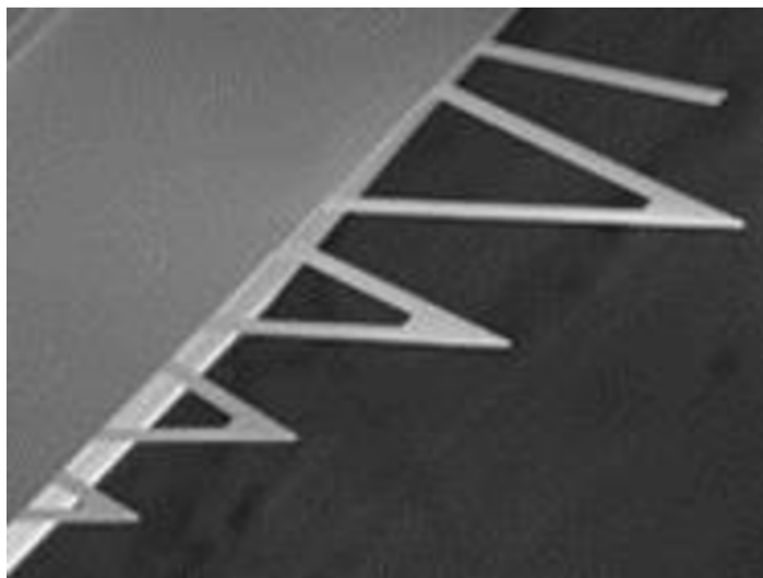
Obrázek 12: čip MLCT na jehož konci je 5 nosníků s hroty
