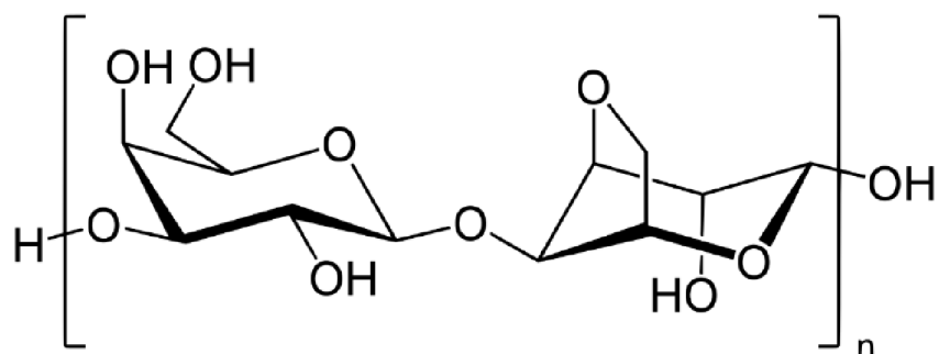
Obrázek 1: Struktura agarózy [21]
