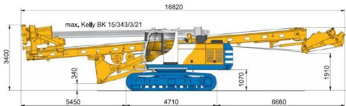
Obr. 6.5 Vrtná souprava BAUER BG 15 H (transportní rozměry) [28]
