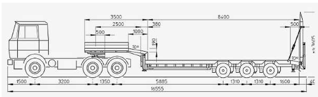
Obr. 6. 9Plošinový podvalník GOLDHOFER STN-L3 BAU [34]
