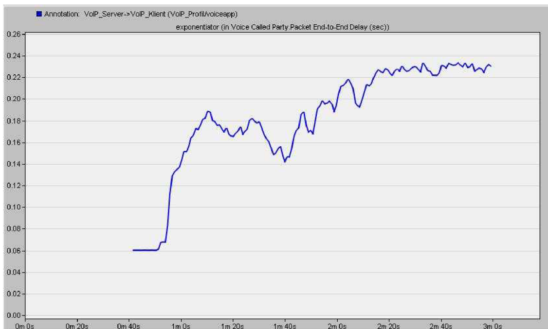
Obr. 21 Statistika zpoždění
