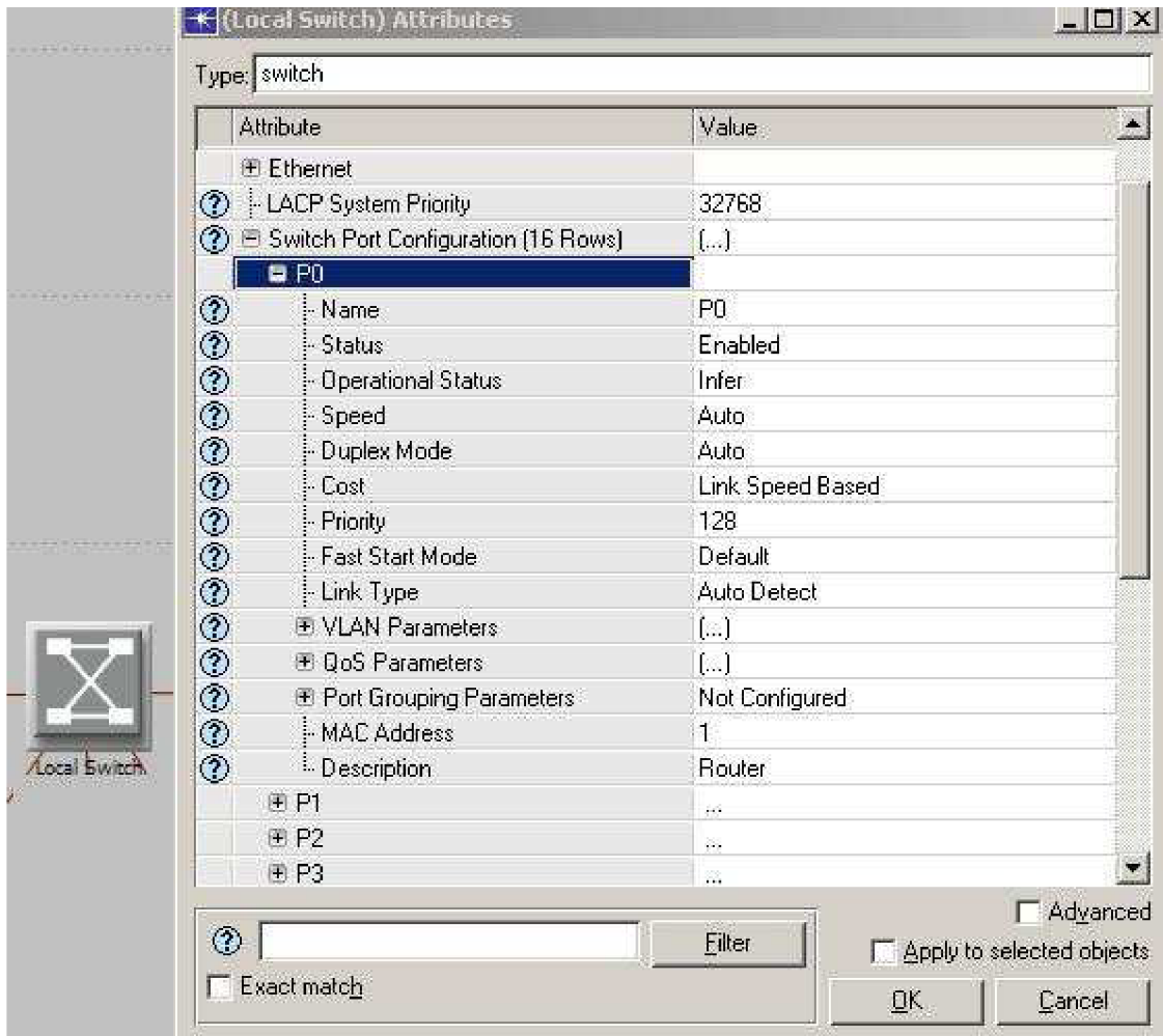
Obr. 14 Nastavení přepínače
