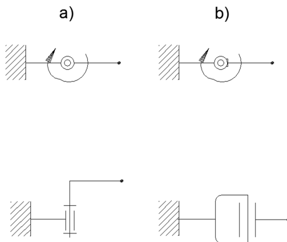
obr. 3 Klouby (rotační KD s ramenem "r") v narysu a půdorysu a) bez omezeného úhlu otáčení, b) s omezeným otáčením [2].
