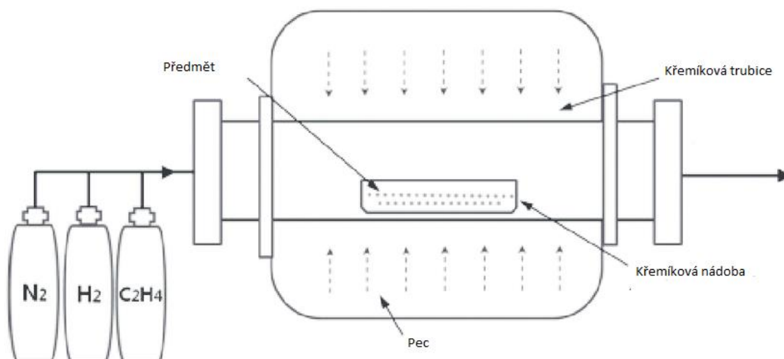
Obr. 2 Schéma povlakování CVD metodou [15].
