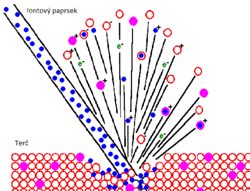
Obr. 9 Schéma vystřelování molekul z terče pomocí iontového paprsku [22].
