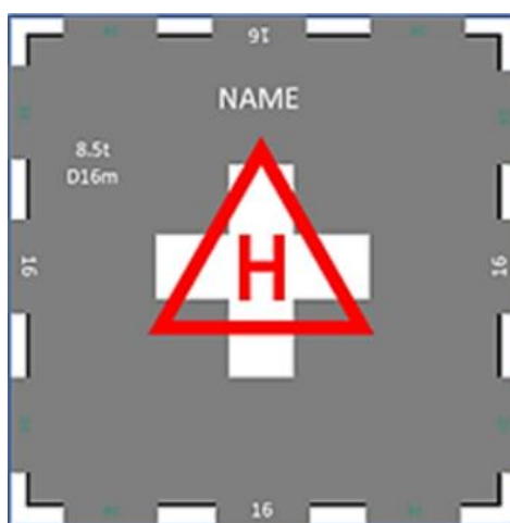
Obr. 9 Poznávací značení heliportu HEMS s TLOF a FATO a značení zaměřovacího bodu. 64
