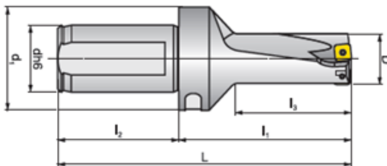
Obr. 14 Vrták 802D-25-50-S32 [18].
