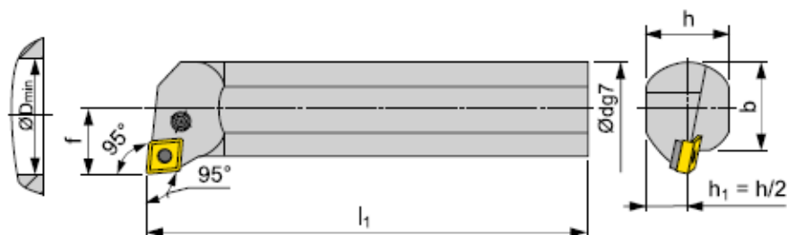
Obr. 12 Nůž A16M-PCLNR 09 [12].
