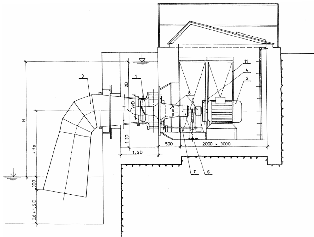
Obr. 7.8-2 Nárýs MVE doporučované firmou ČKD Blansko
