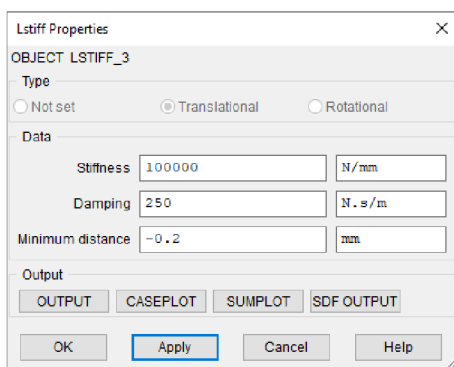
Obr. 5.23: Definice kontaktu vačky a zdvihátka
