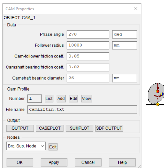
Obr. 5.21: Definice vačky
