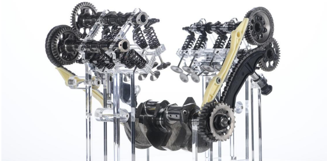
Obr. 2.18: Motor V4 Granturismo [35]
