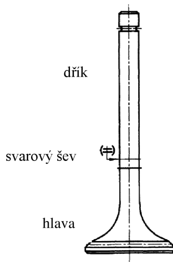
Obr. 2.9: Bimetalový ventil [4]
