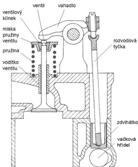
Obr. 2.3: Rozvod OHV [26]
