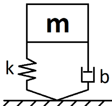
Obr. 5.3: Schéma dynamického modelu s 1° volnosti
