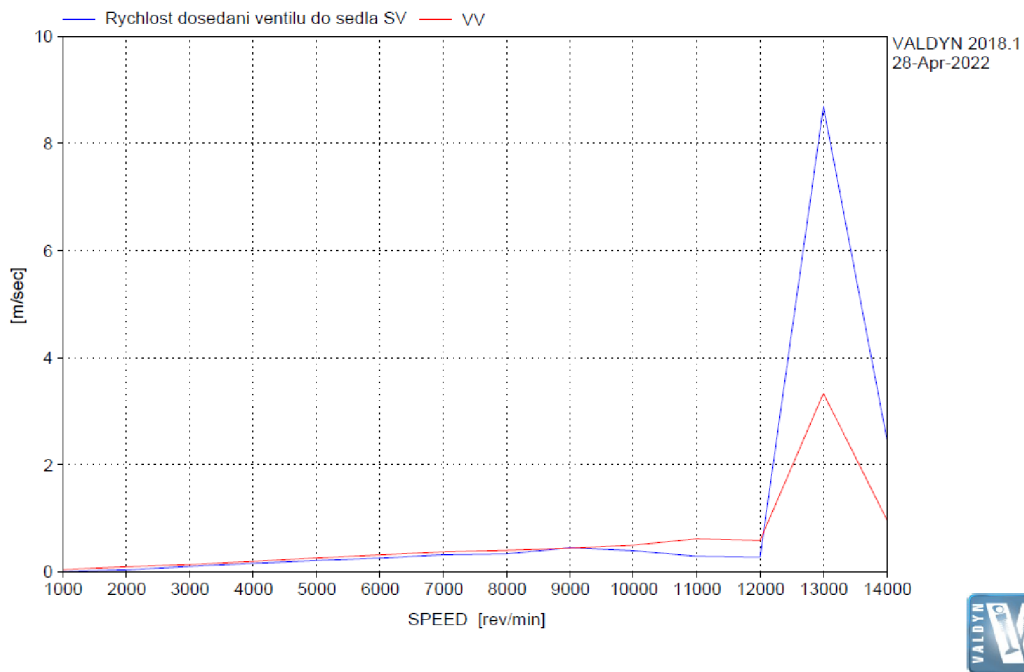
Graf 28: Rychlost dosedání ventilu do sedla
