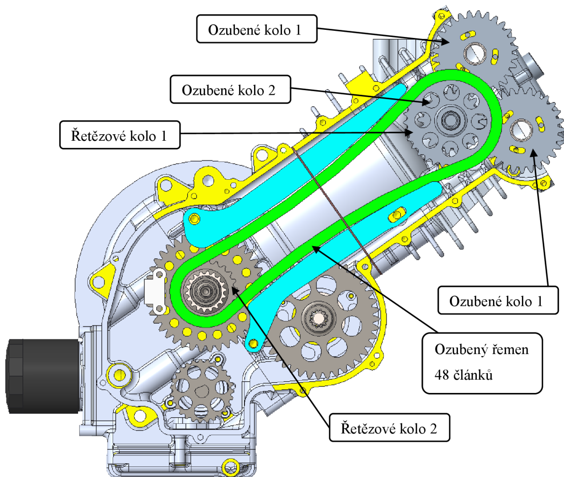
Obr. 4.3: Rozvod motoru
