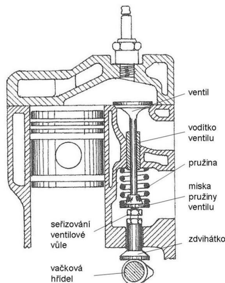
Obr. 2.2: Rozvod SV [25]
