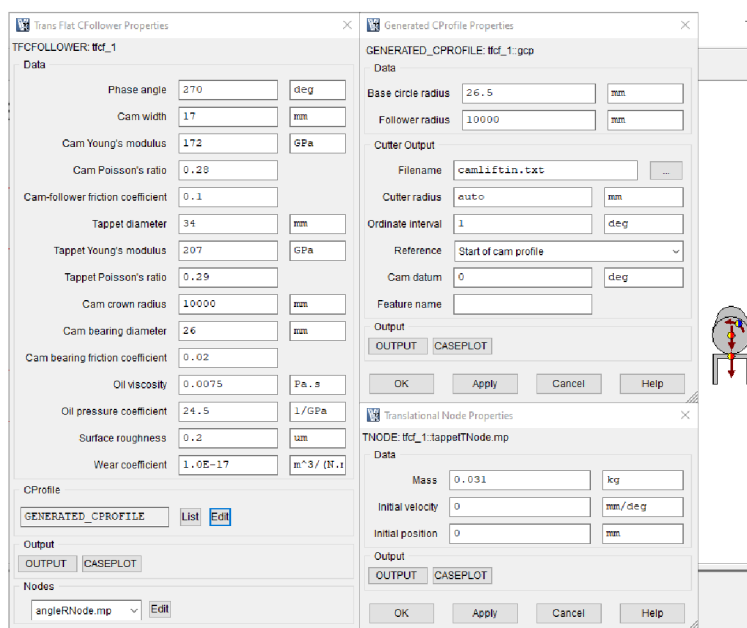
Obr. 5.11: Definice vačky s hříčkovým zdvihátkem
