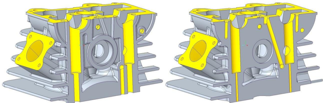
Obr. 4.5: Řez přívodním mazacím kanálkem
