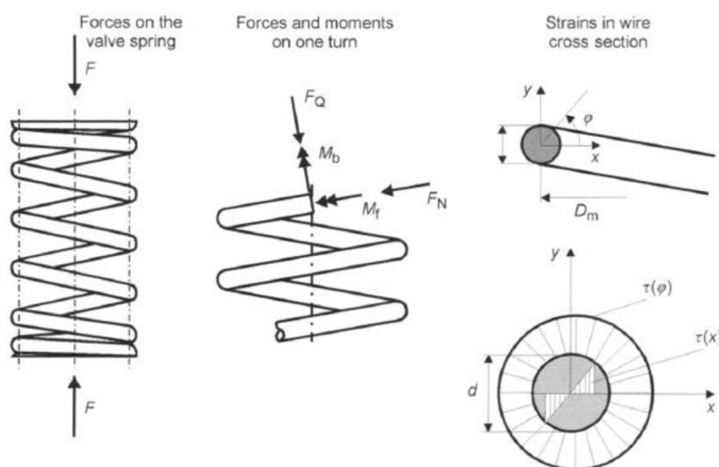
Obr. 2.15: Namáhání pružiny [4]
