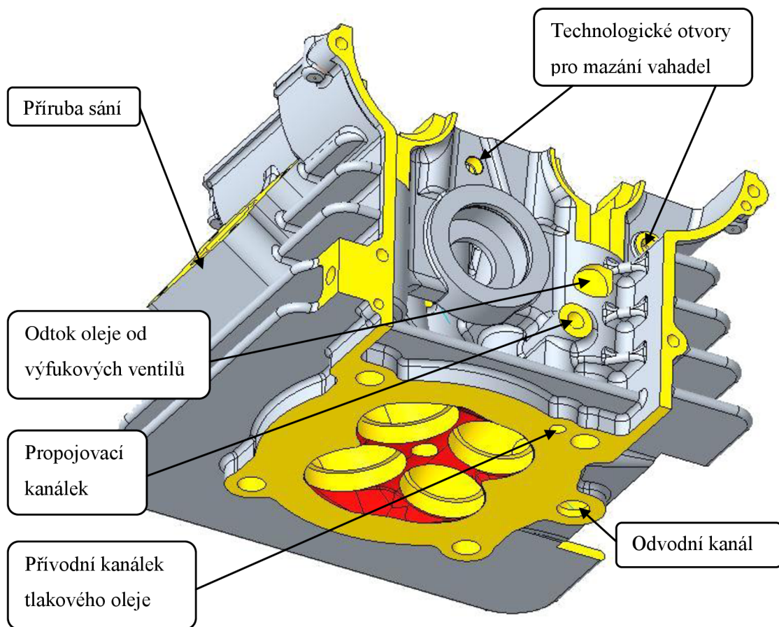
Obr. 4.4: Přívod oleje
