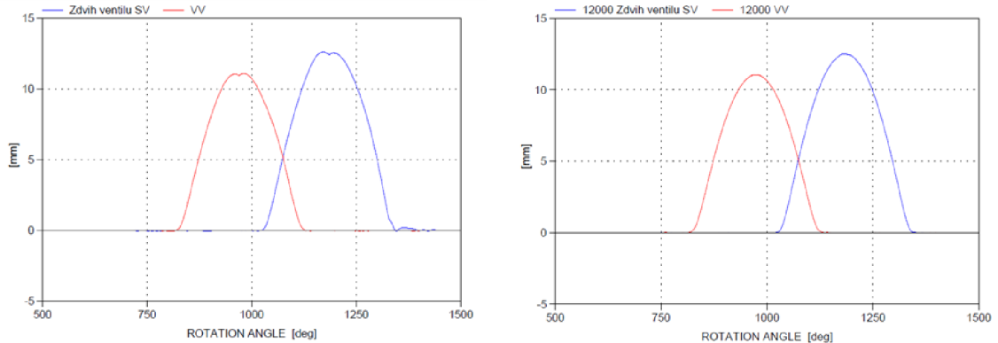
Graf 35: Porovnání zdvihu ventilu pro 12000 ot.min -1
