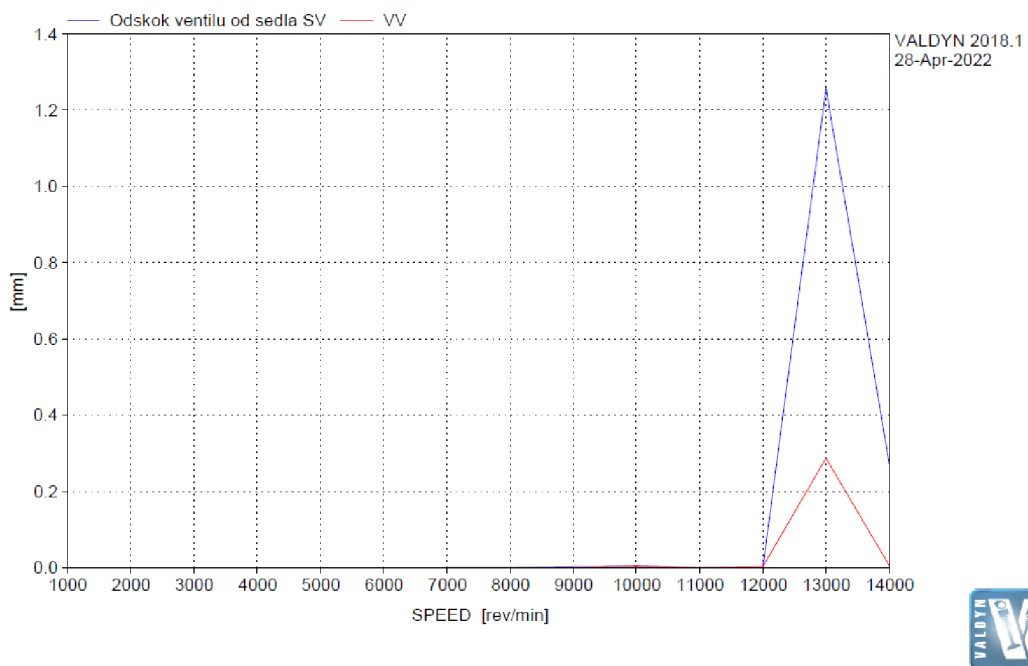
Graf 29: Odskok ventilu ze sedla
