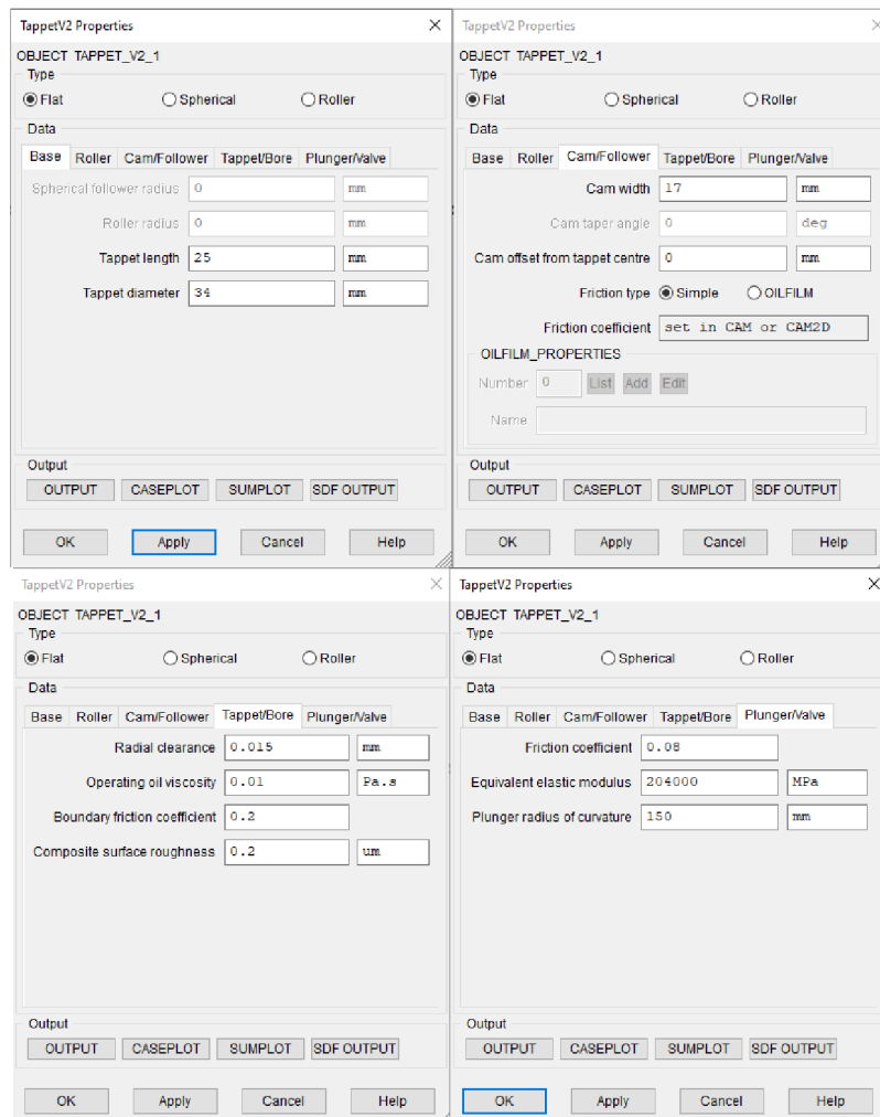
Obr. 5.25: Definice hříčkového zdvihátka
