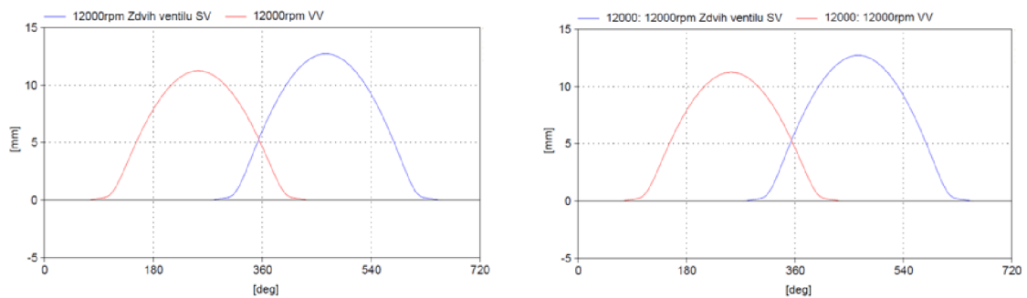
Graf 31: Porovnání zdvihu ventilu pro 12000 ot.min -1
