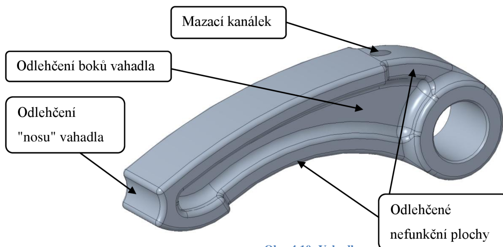
Obr. 4.10: Vahadlo
