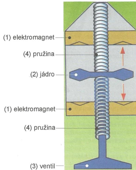
Obr. 3.3: Schéma systému EVA [6]
