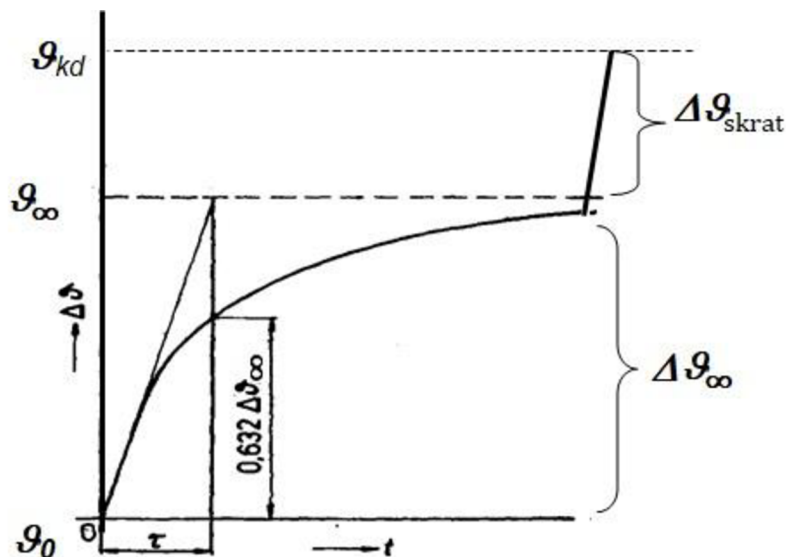
Obrázok 6 - Priebeh najnepriaznivejšieho oteplenia prístroja (pôsobením skratu) [6]
