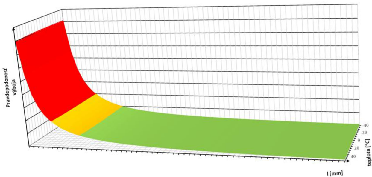
Obrázok 11 - Pravdepodobnosť medzifázového výboja v závislosti na vzdialenosti a okolitej teplote
