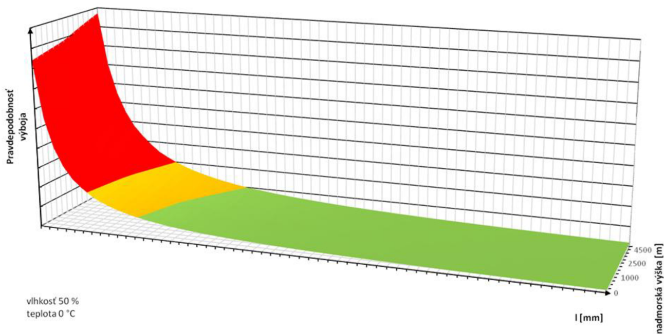
Obrázok 12 - Pravdepodobnosť medzfázového výboja v závislosti na vzdialenosti a nadmorskej výške
