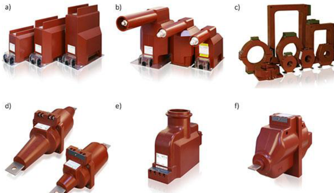
Obrázok 1 - Prístrojové transformátory z ponuky firmy ABB [2] a) prúdový TPU b) napätový TJP c) prúdový káblový vnútorný d) typ TTR e) typ PR 25 f) typ TSR
