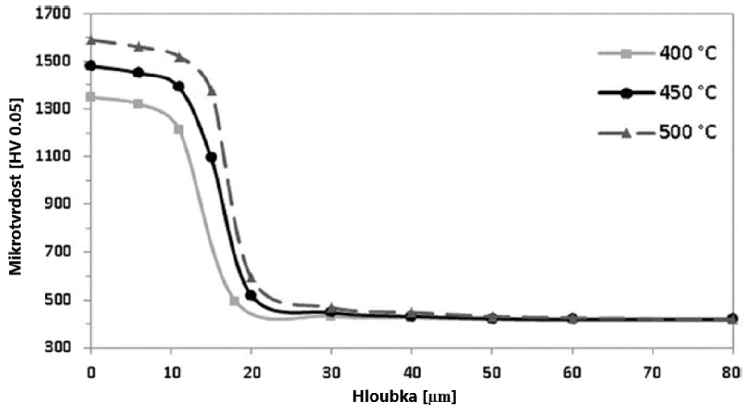
Obr. 11 Mikrotvrdomost povrchu Inconelu 718 plazmově nitridovaném při různých teplotách po dobu 6 hodin [34]
