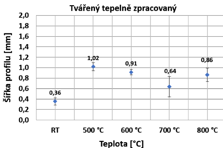
Obr. 41 Šířka profilu pro tvářený tepelně zpracovaný materiál
