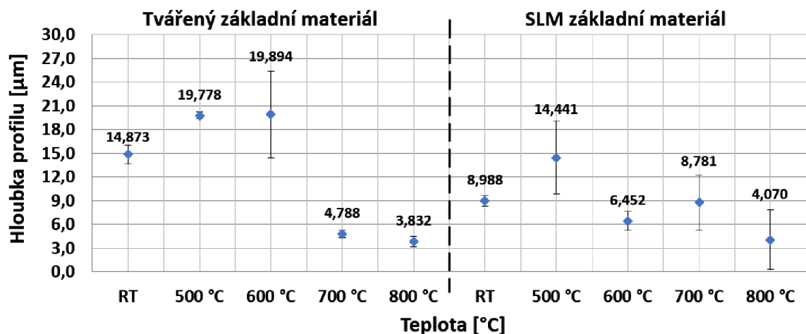
Obr. 36 Hloubka profilu pro tvářený základní materiál a SLM základní materiál
