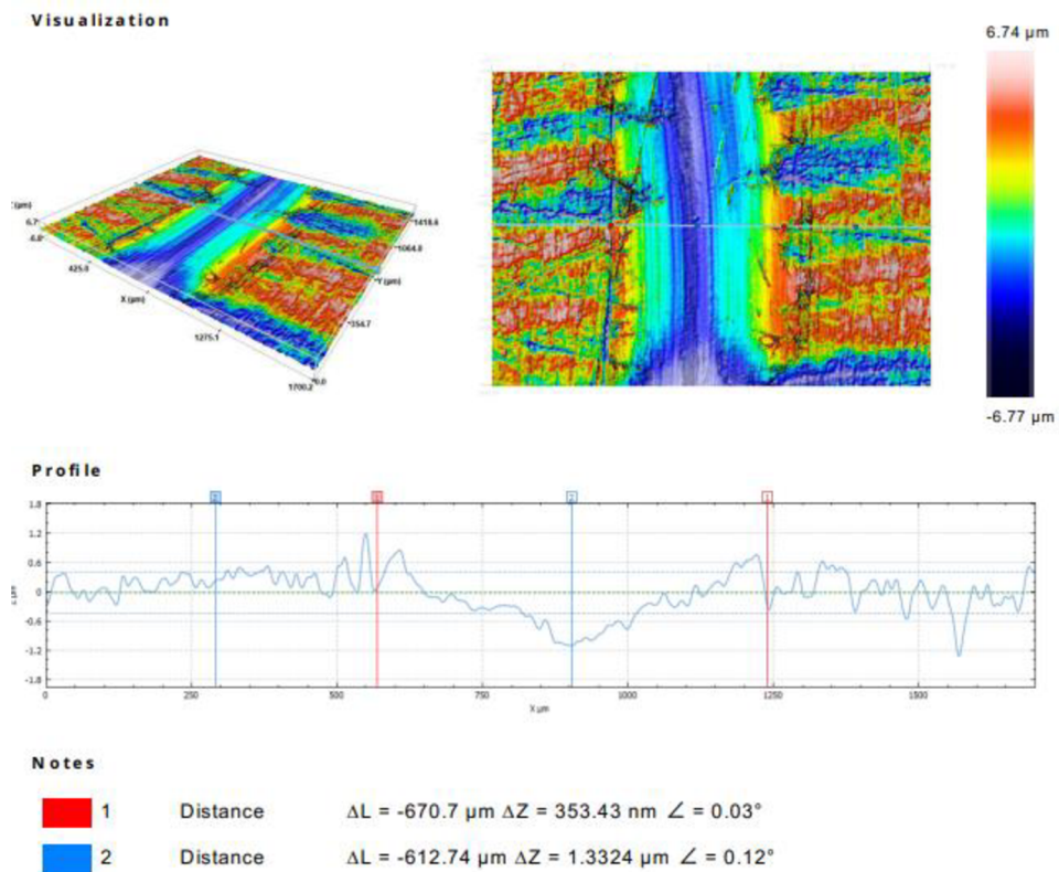
Obr. 35 Opatřebenění zkušebního vzorku – SLM základní materiál + plazmová nitridace při teplotě RT
