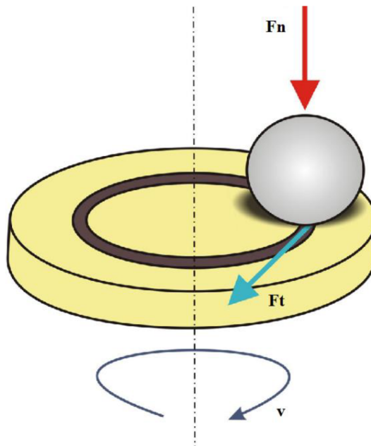
Obr. 17 - Princip tribologické metody Ball-on-Disc [44]
