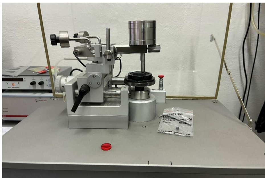
Obr. 22 Tribometr pro suché a kapalně prostředí
