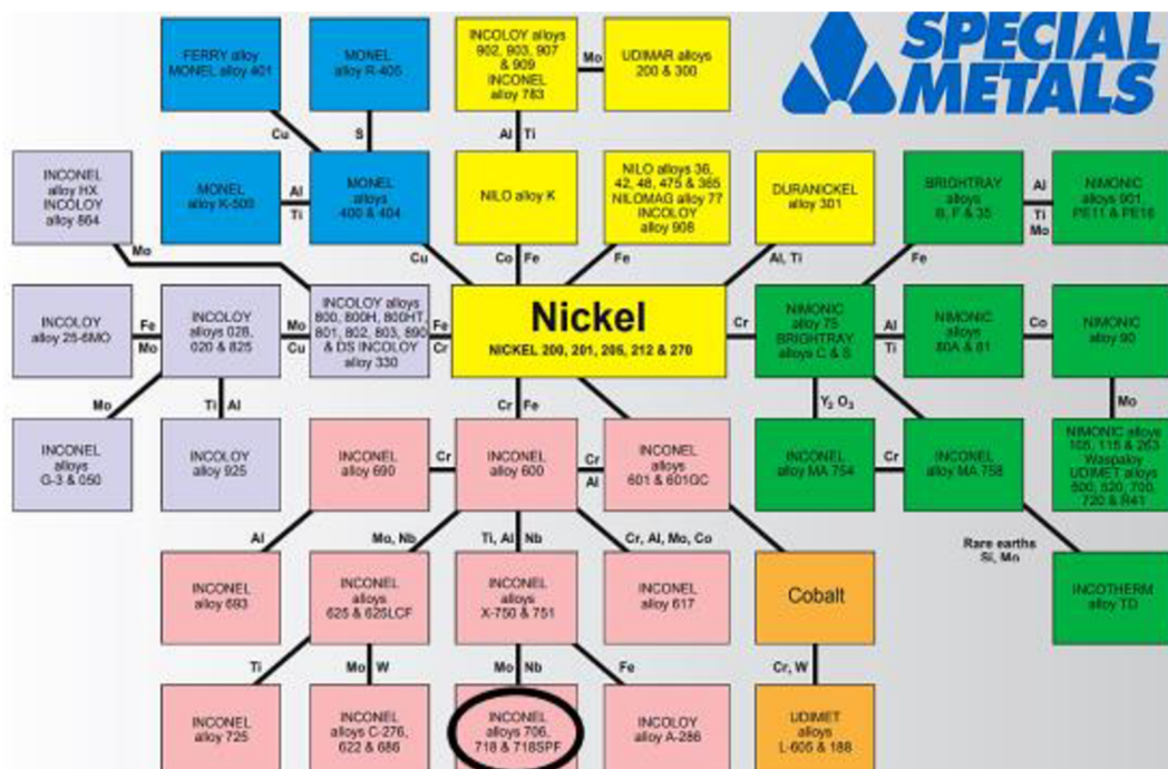
Obr. 1 - Grafický přehled niklových slitin [4]
