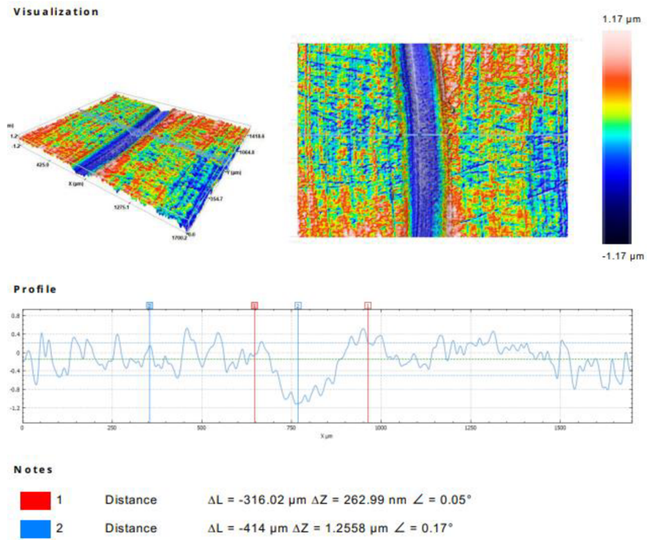
Obr. 34 Opatřebenění zkušebního vzorku – tvářený základní materiál + plazmová nitridace při teplotě RT
