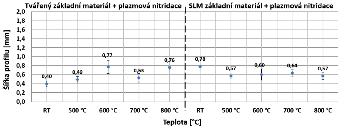
Obr. 42 Šířka profilu pro tvářený a SLM základní materiál s nitridací
