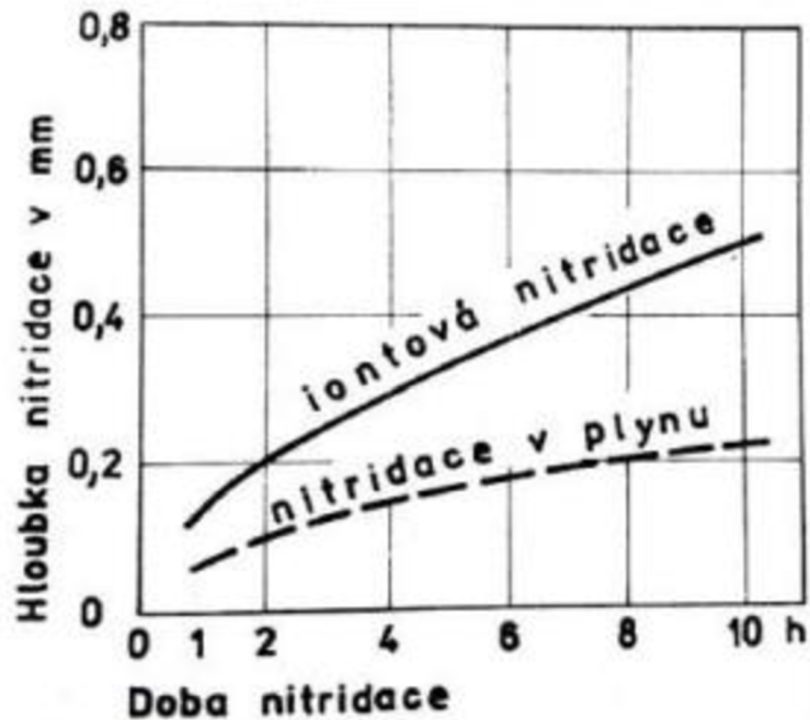
Obr. 10 Porovnání tloušťky nitridované vrstvy za čas pro plazmovou nitridaci a nitridaci v plynu [26]
