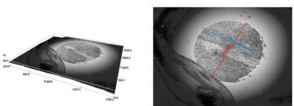
Obr. 44 Opotřebení kuličky vzniklé při teplotě RT pro tvářený základní materiál s nitridací
