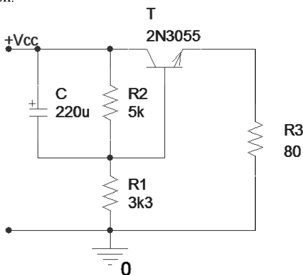
Obr. 7.7 Regulace otáček ventilátoru
