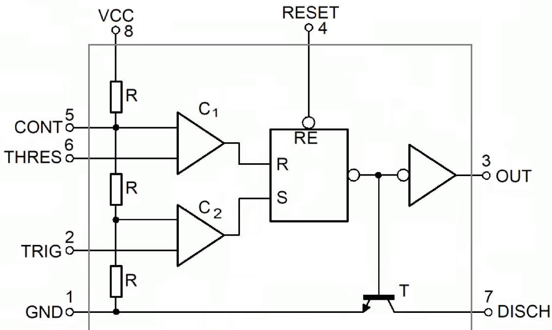
Obr. 6.2 Vnitřní zapojení 555
