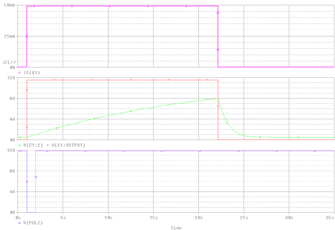
Obr. 7.6 Analýza časovače
