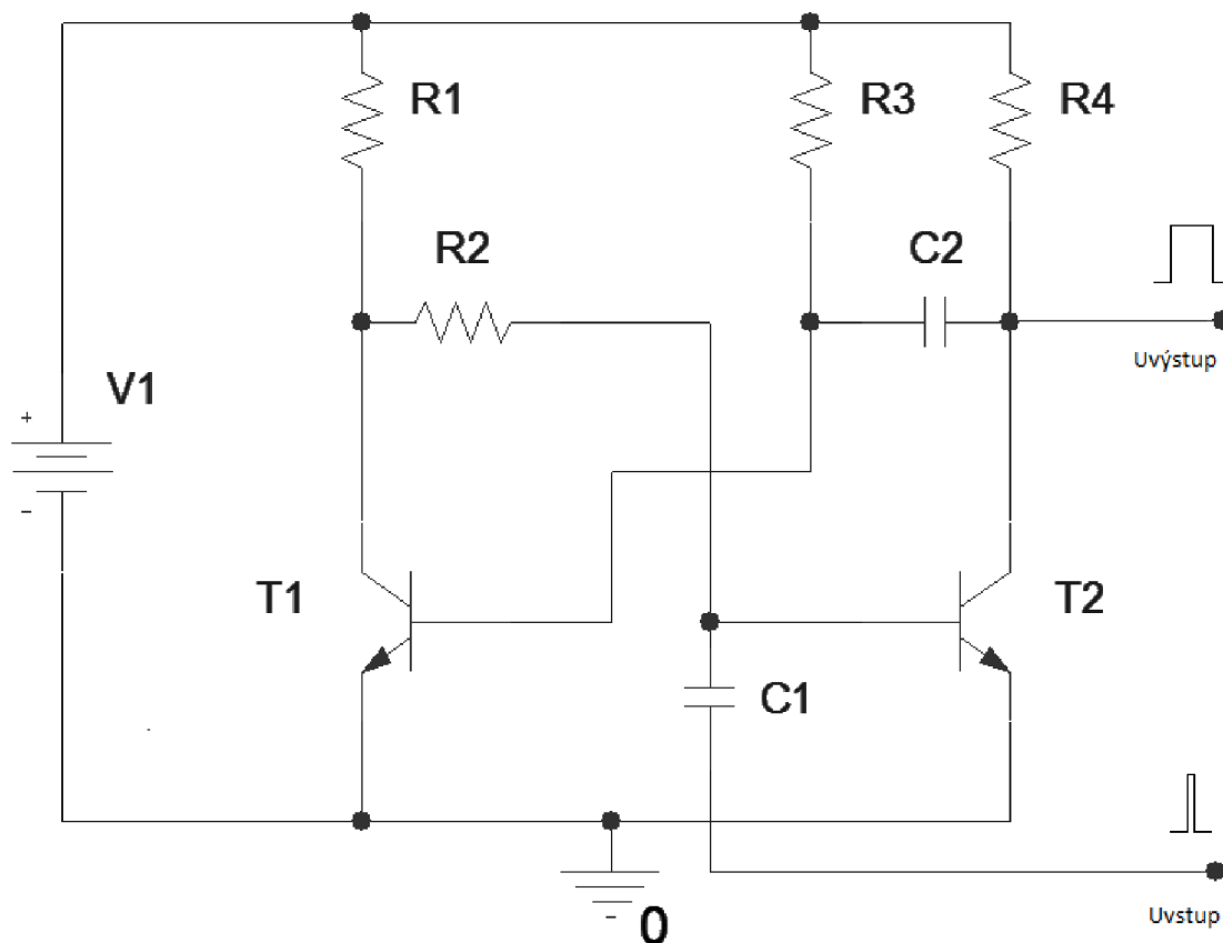
Obr. 7.2 Monostabilní klopný obvod
