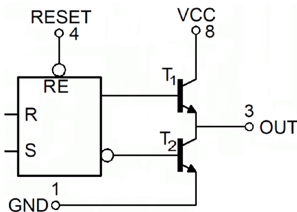
Obr. 6.3 Nahrazení výkonového členu tranzistory
