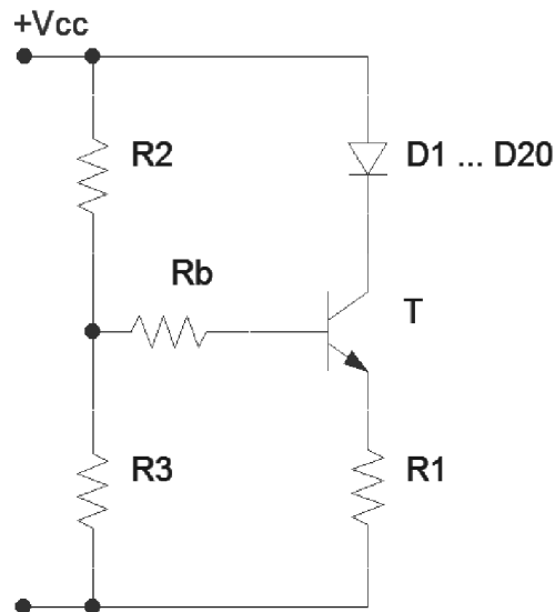
Obr. 7.9 Regulace pomocí děliče a tranzistoru
