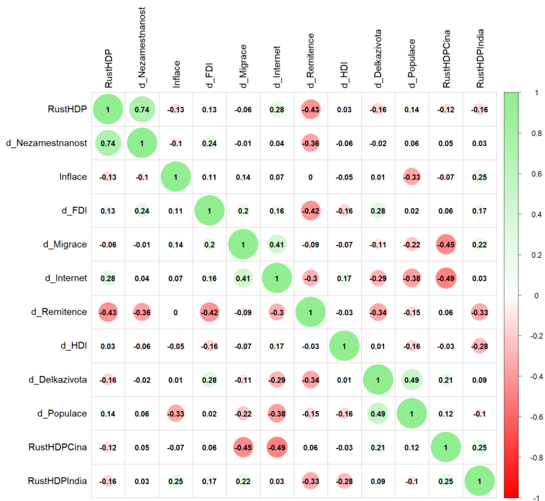
Obrázek 7: Korelační matice
