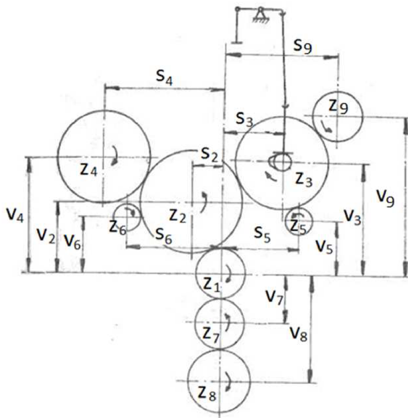
Obr. 14 Schéma rozložení kol rozvodu traktorového motoru [6]
