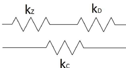
Obr. 40 Model tuhostí záběru, disku a celkové tuhosti
