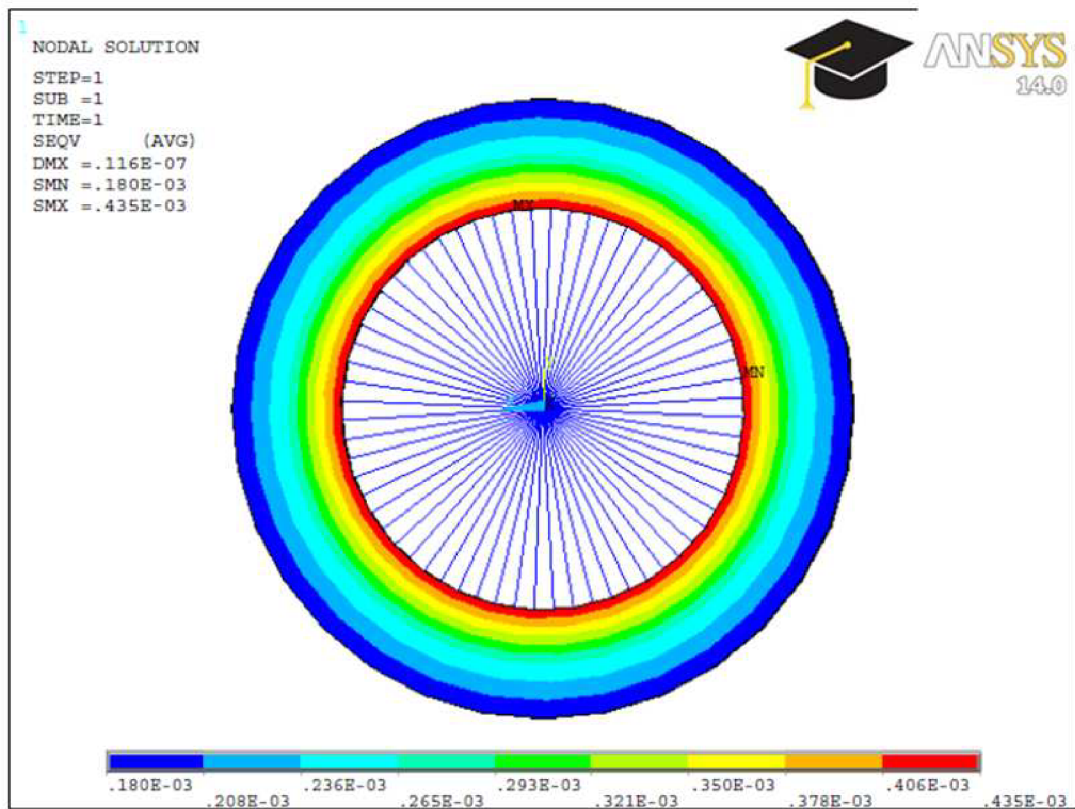
Obr. 38 Konturové znázornění natočení
