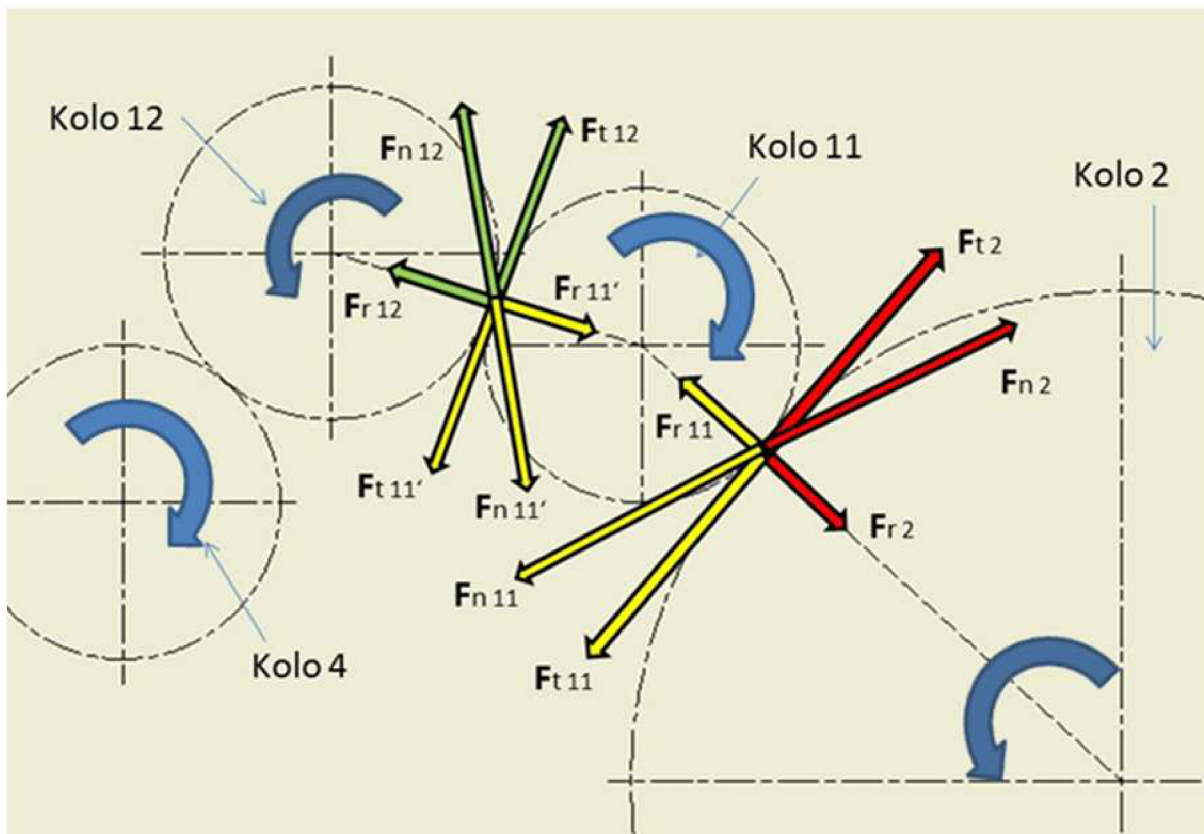
Obr. 42 Síly působící na ozubené kolo 11 z varianty B
