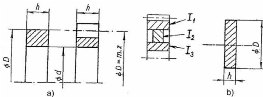
Obr. 41 Průřezy a) prstenec b) kotouč [20]
