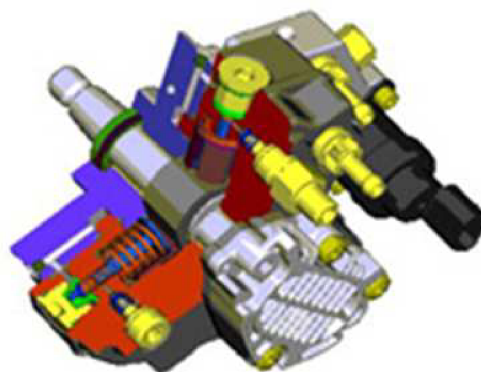
Obr. 6 Řez čerpadlem CP3 BOSCH [12]
