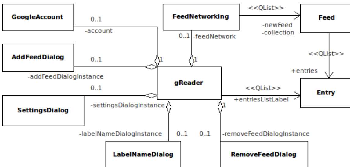
Obrázek 5.1: UML diagram aplikace gReader
