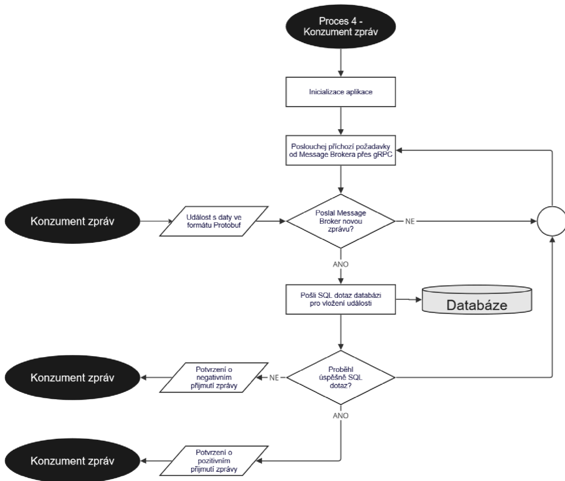
Obrázek 4.8 Proces konzumenta zpráv
