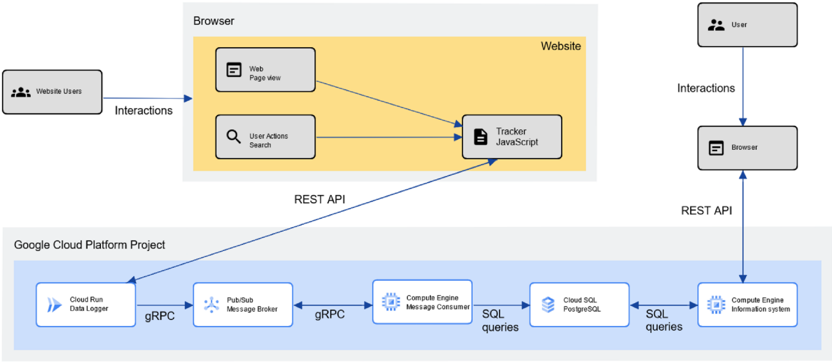
Obrázek 4.13 Blokové schéma systému
