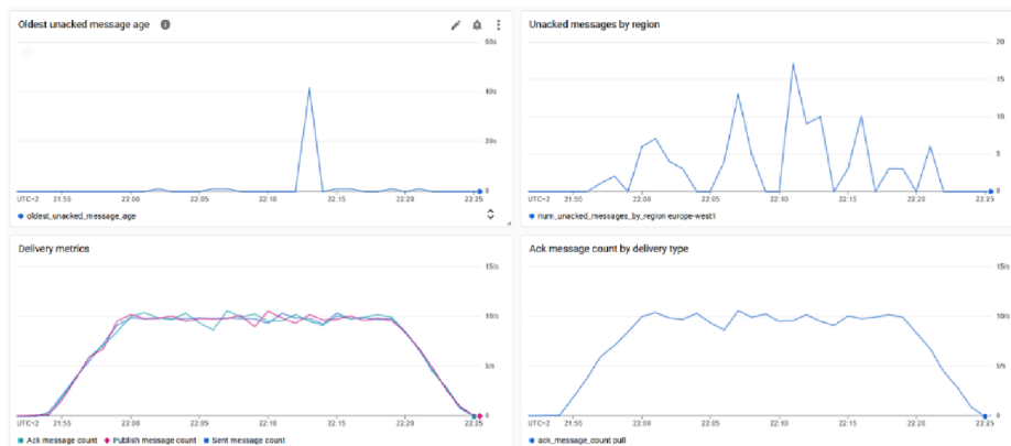
Obrázek 6.3 Testovací scénář 1 – výsledky z pohledu message brokera
