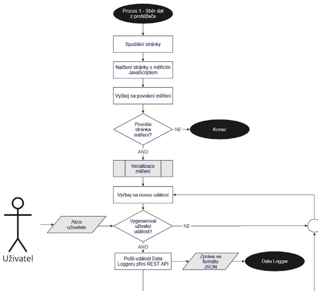
Obrázek 4.1 Proces sběru dat z prohlížeče
