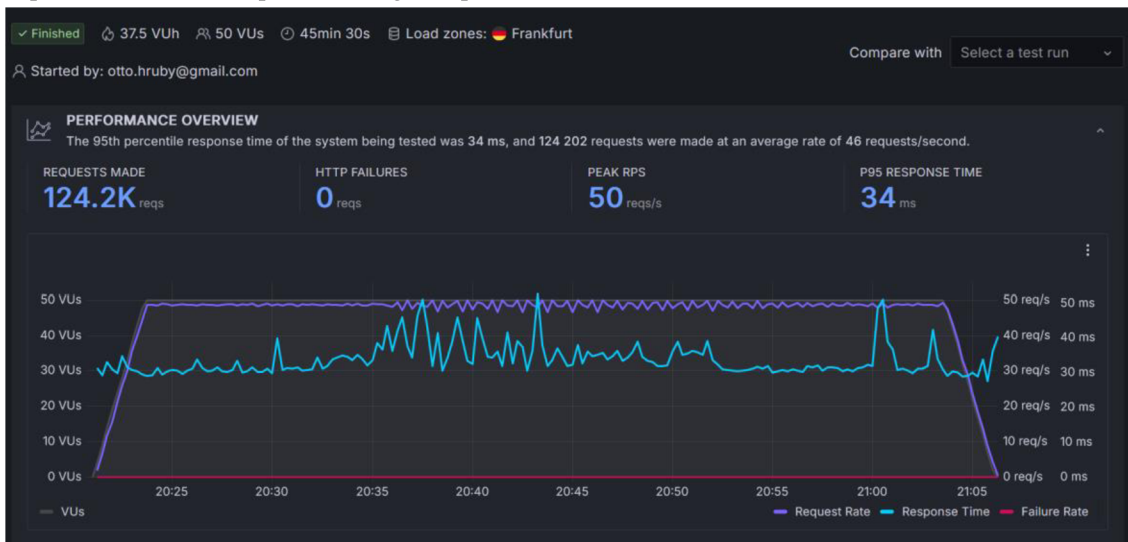
Obrázek 6.5 Testovací scénář 2 – výsledky z pohledu virtuálních uživatelů
