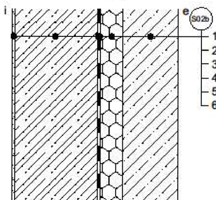
Obrázek 25. Schéma skladby konstrukce S02b
