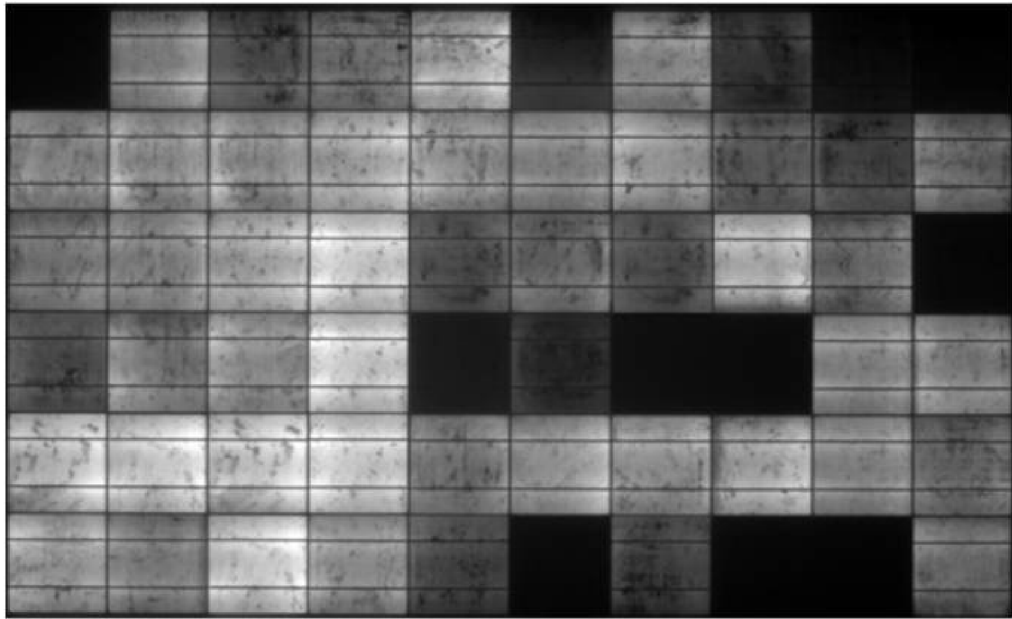
Obrázek 15. Elektroluminiscence [23]
