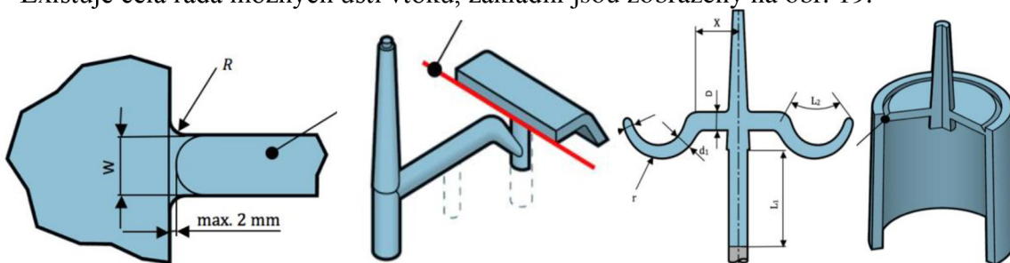
Obr. 19 Základní typy ústí vtoků [18]
