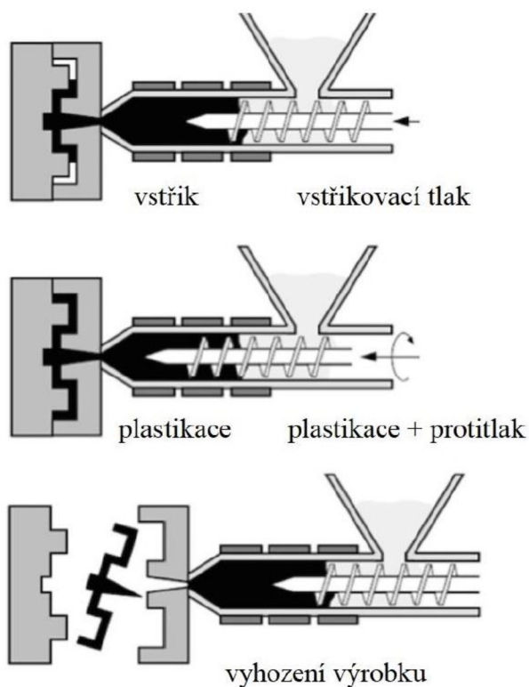
Obr. 7 Postup při vstříkování plastů [9]
