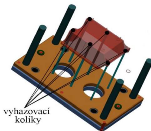
Obr. 24 Vyhození pomocí kolíků [18]
