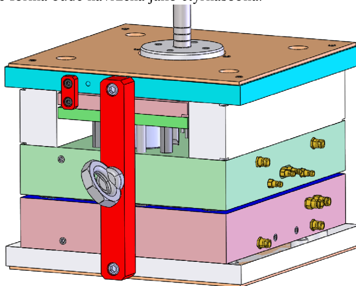
Obr. 33 Vstřikovací nástroj
