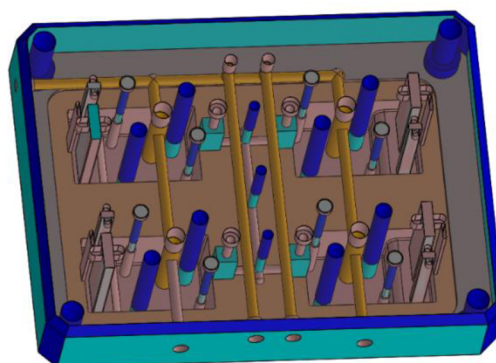
Obr. 38 Tvárnice
