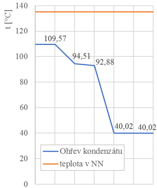
Obr. 4.8 Nizkotlaká regenerace tepla, minimální průtok páry, topný režim ( Q_{TV} = 4,5 \text{ MW} )
