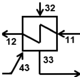
Obr. 1.6 Bilance NTO 1
