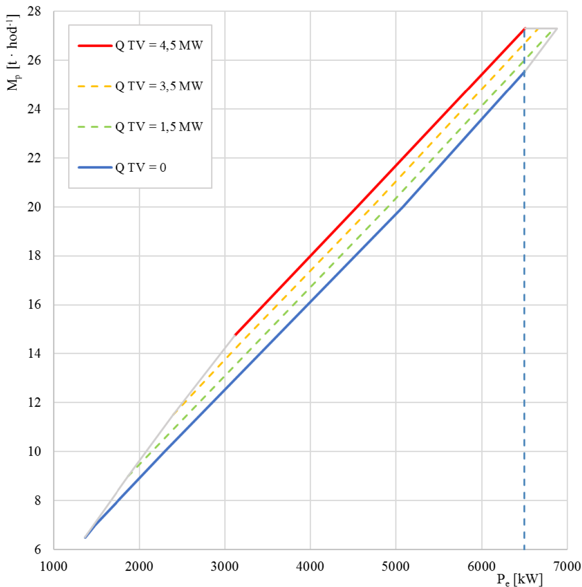
Obr. 4.14 Spotřební diagram, zimní režim provozu topného výměníku
