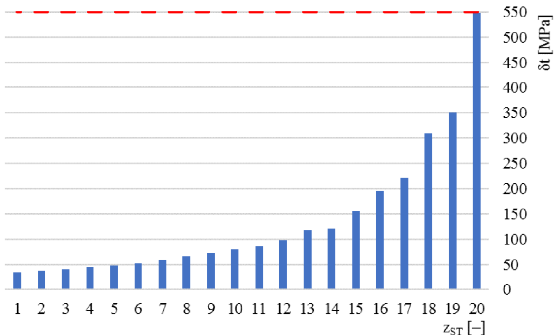
Obr. 3.1 Namáhání oběžných lopatek v tahu
