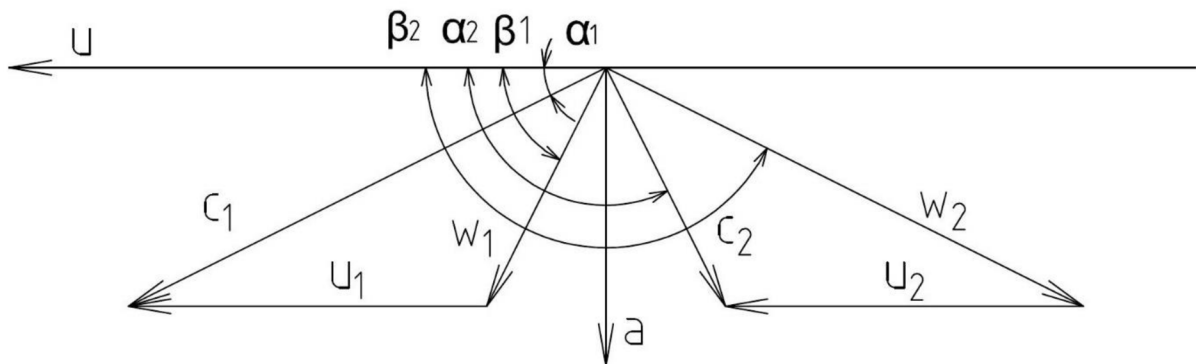
Obr. 2.3 Rychlostní trojúhelníky – značení
