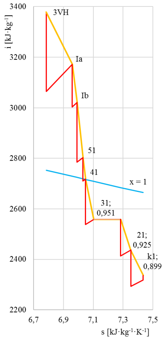
Obr. 4.2 i-s diagram expanze páry v turbíně, jmenovitý výkon, topný režim ( Q_{TV} = 4,5 \text{ MW} , 90/70 \text{ }^\circ\text{C} )
