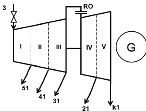
Obr. 1.3 Bilance turbíny
