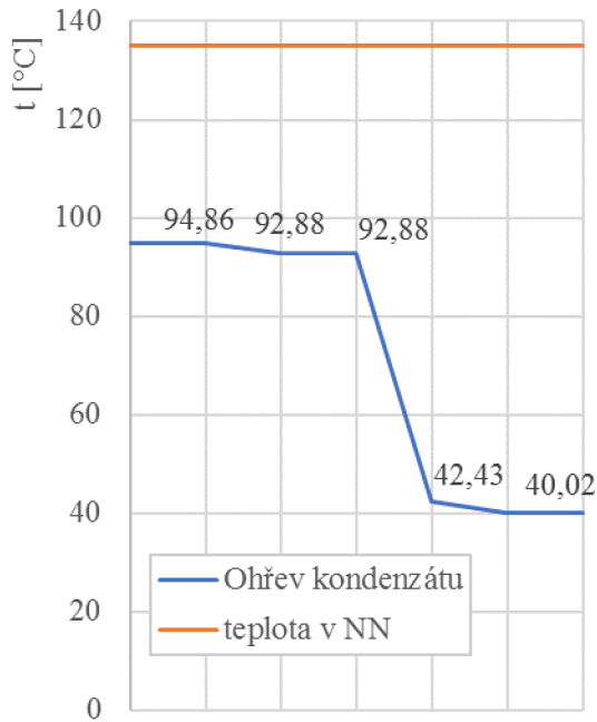
Obr. 4.7 Nizkotlaká regenerace tepla, minimální průtok páry, kondenzační režim
