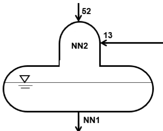
Obr. 1.9 Bilance napájecí nádrže
