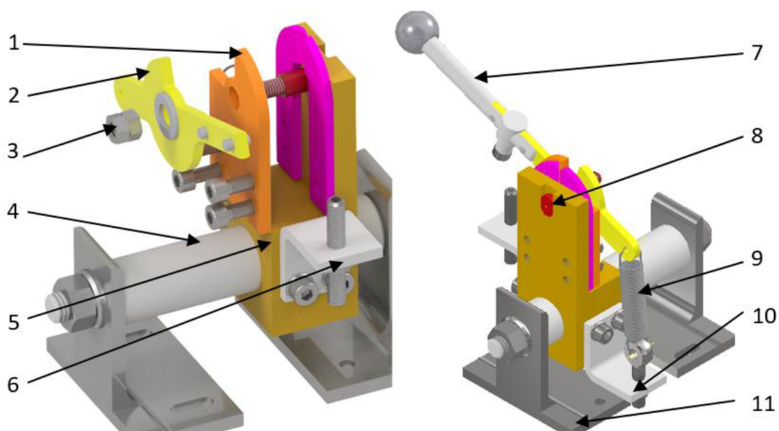
Obr. 5-6 Náhled mechanismu pro zastřížení a nařezání s označením důležitých součástí
