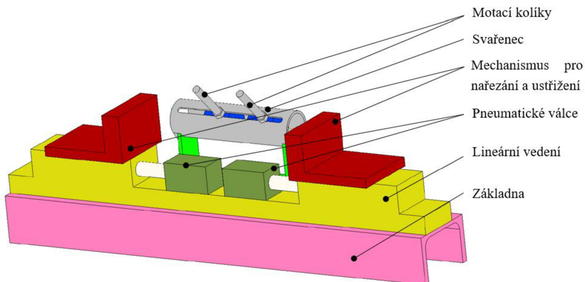
Obr. 4-2 Náhled druhé koncepční varianty s popisem využitých součástí
