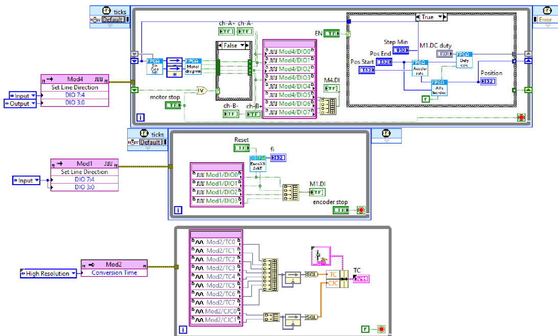
Obrázek 2.8: LabVIEW kód běžící na FPGA čipu
