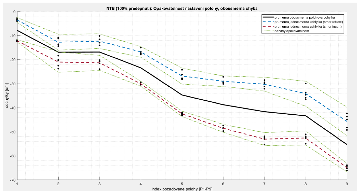
Obrázek 2.19: Výsledek měření matice typu NTB pro úroveň předeprnutí 100 %
