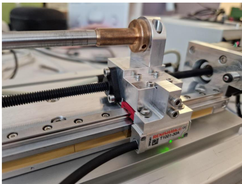
Obrázek 2.3: Uchytení enkodéru a pravítka na skutečném zařízení v laboratoři
