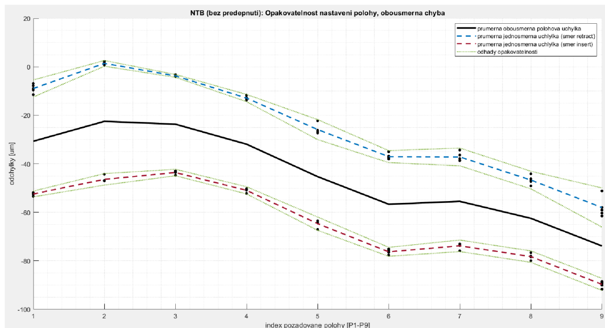
Obrázek 2.15: Výsledek měření matice typu NTB pro úroveň předeprnutí 0 %
