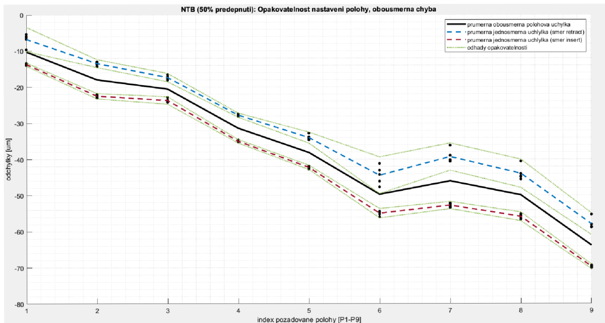
Obrázek 2.17: Výsledek měření matice typu NTB pro úroveň předepnutí 50 %
