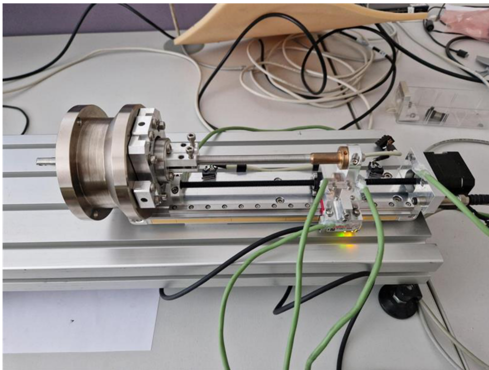
Obrázek 2.5: Retract kompletně osazený měřicími prvky. Zelené kabely jsou termočládky T1-T5
