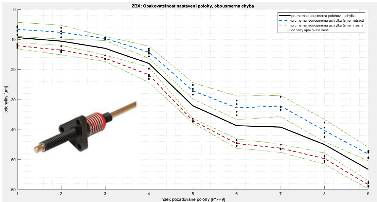
Obrázek 2.13: Výsledek měření matice typu ZBX
