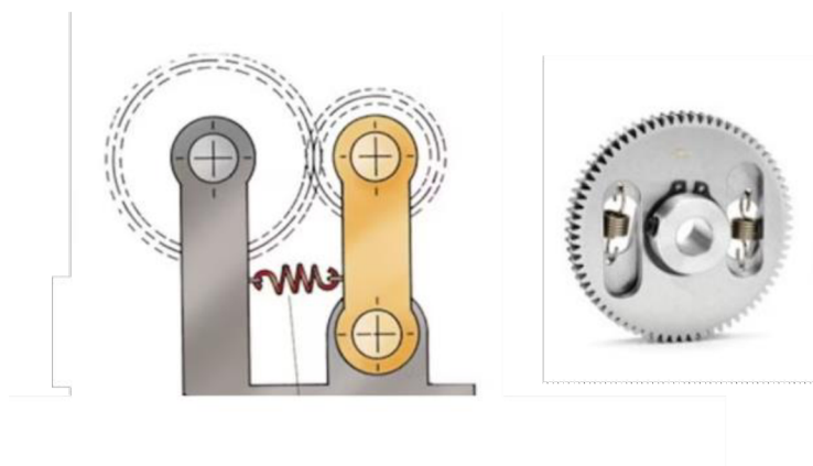
Obrázek 1.9: Možnosti předeptnutí ozubených kol [7], [8]
