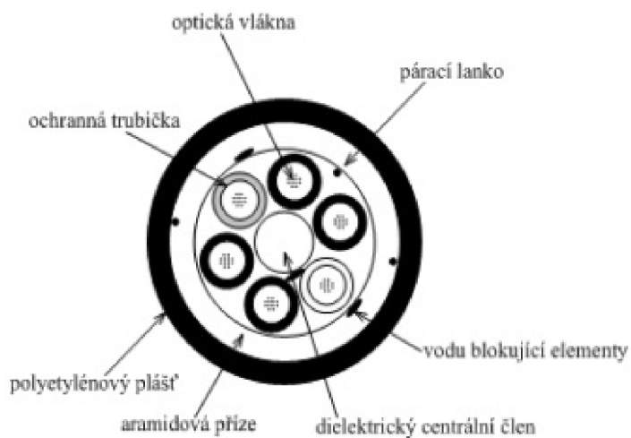
Obr. 2.8: Kabel OPTION1 [5].
