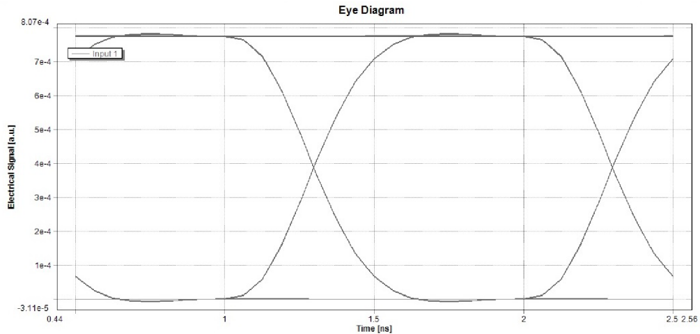
Obr. 7.4: Diagram oka rozhodnutí pro trasu 8 km
