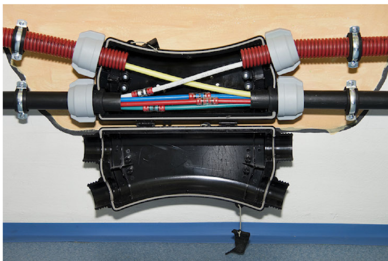
Obr. 3.2: Chráníčka spojek
