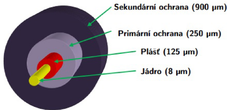
Obr. 2.6: Řez kabelem. [1].
