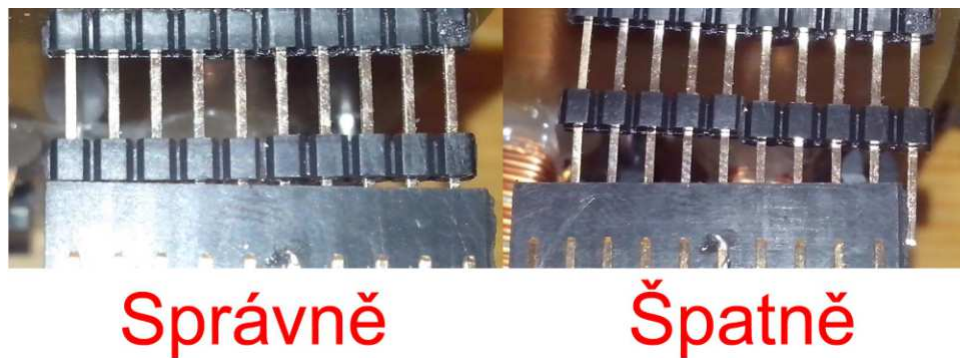
Obr. 1.15: Propojení modulů
