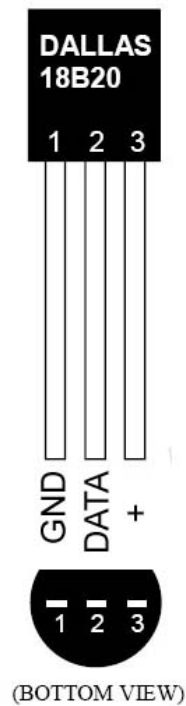
Obr. 1.13: Rozložení vývodů u čidla
