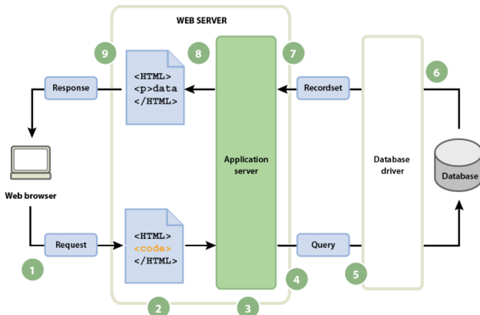
Obrázek 3 – Přístupování k databázi [8]
