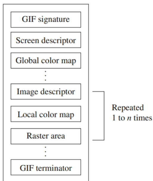
Obrázek 7 – Formát GIF87a [15]
