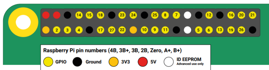
Obrázek 11 – Význam jednotlivých GPIO pinů [17]
