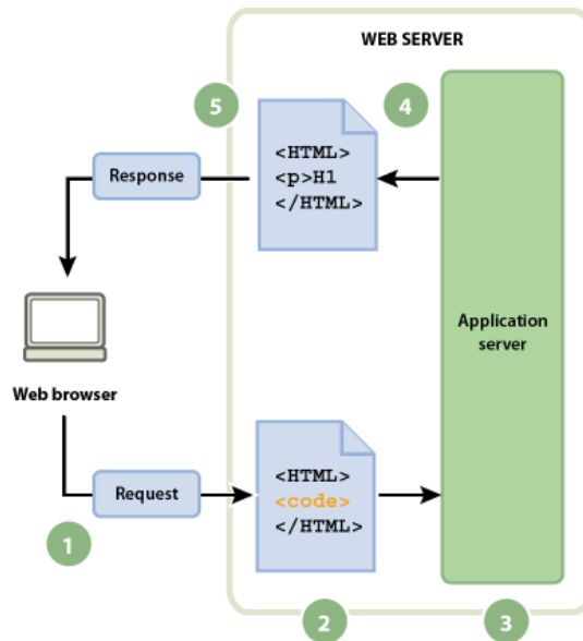
Obrázek 2 – Zpracování dynamických stránek [8]
