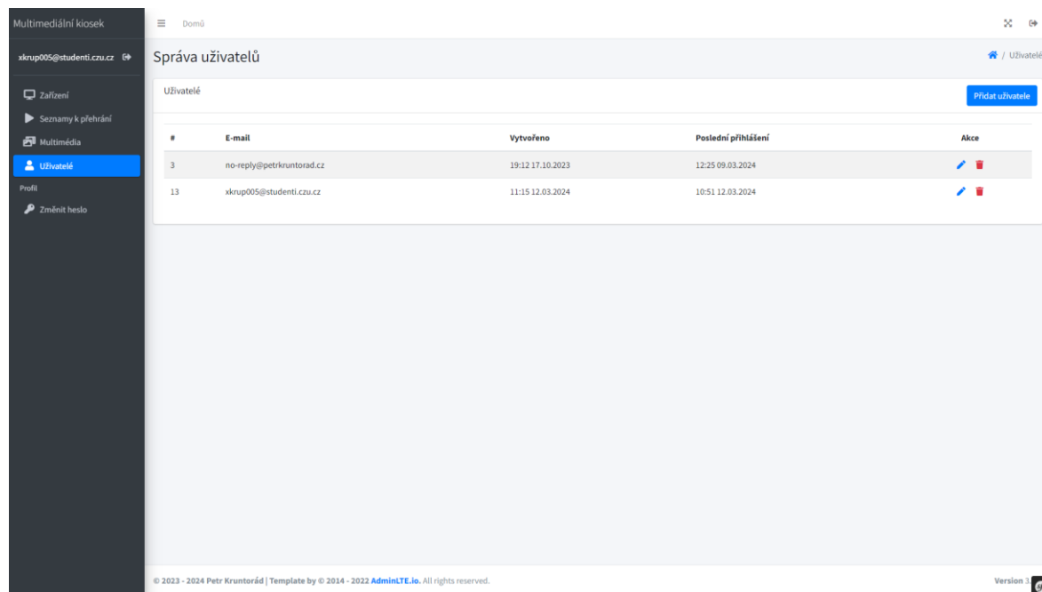
Obrázek 30 – Stránka uživatelé
