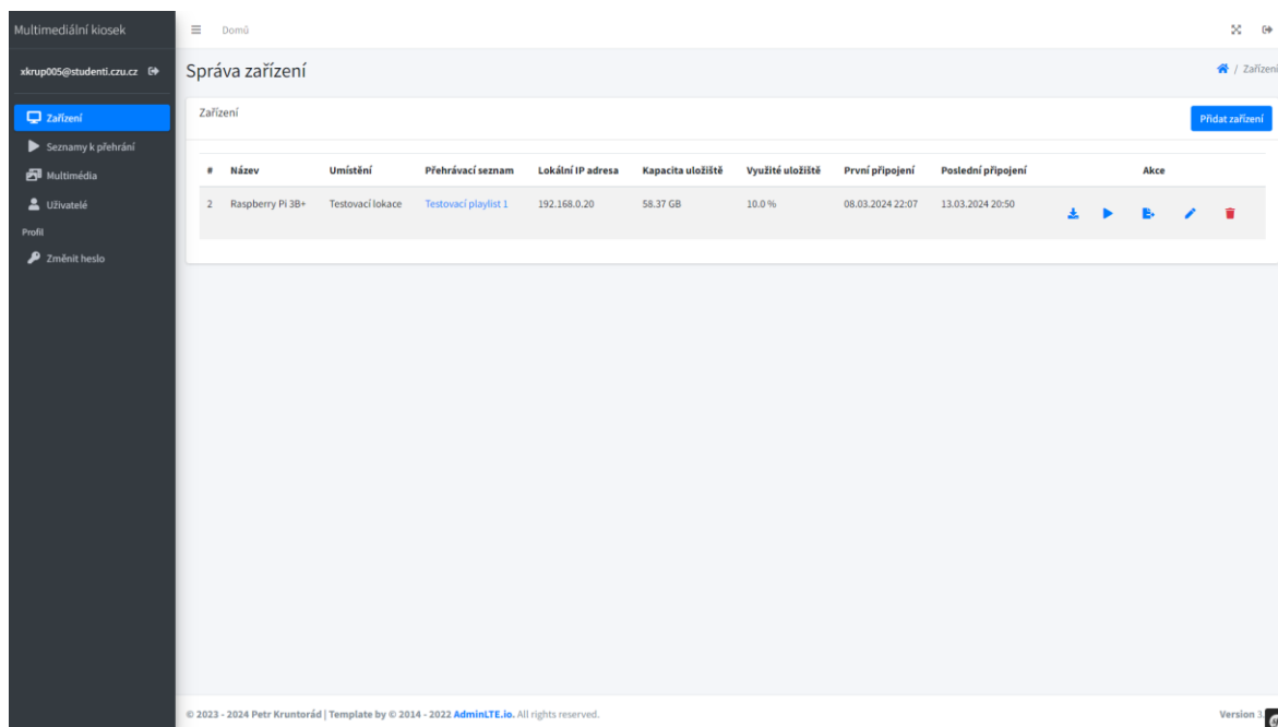
Obrázek 25 – Stránka zařízení
