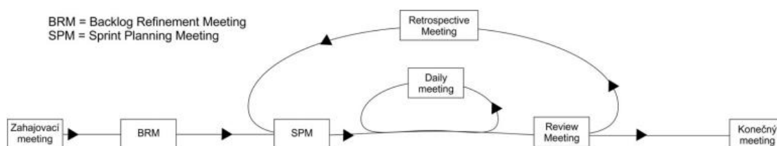
Obrázek 6 – Průběh vývojového cyklu řízeného metodikou SCRUM [10]
