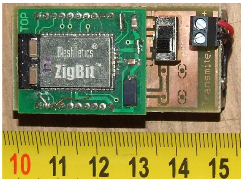
Obr. 8.11: Horní pohled na vysílač
