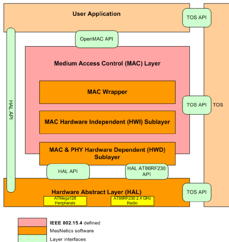
Obr. 7.1: Architektura OpenMAC Layer
