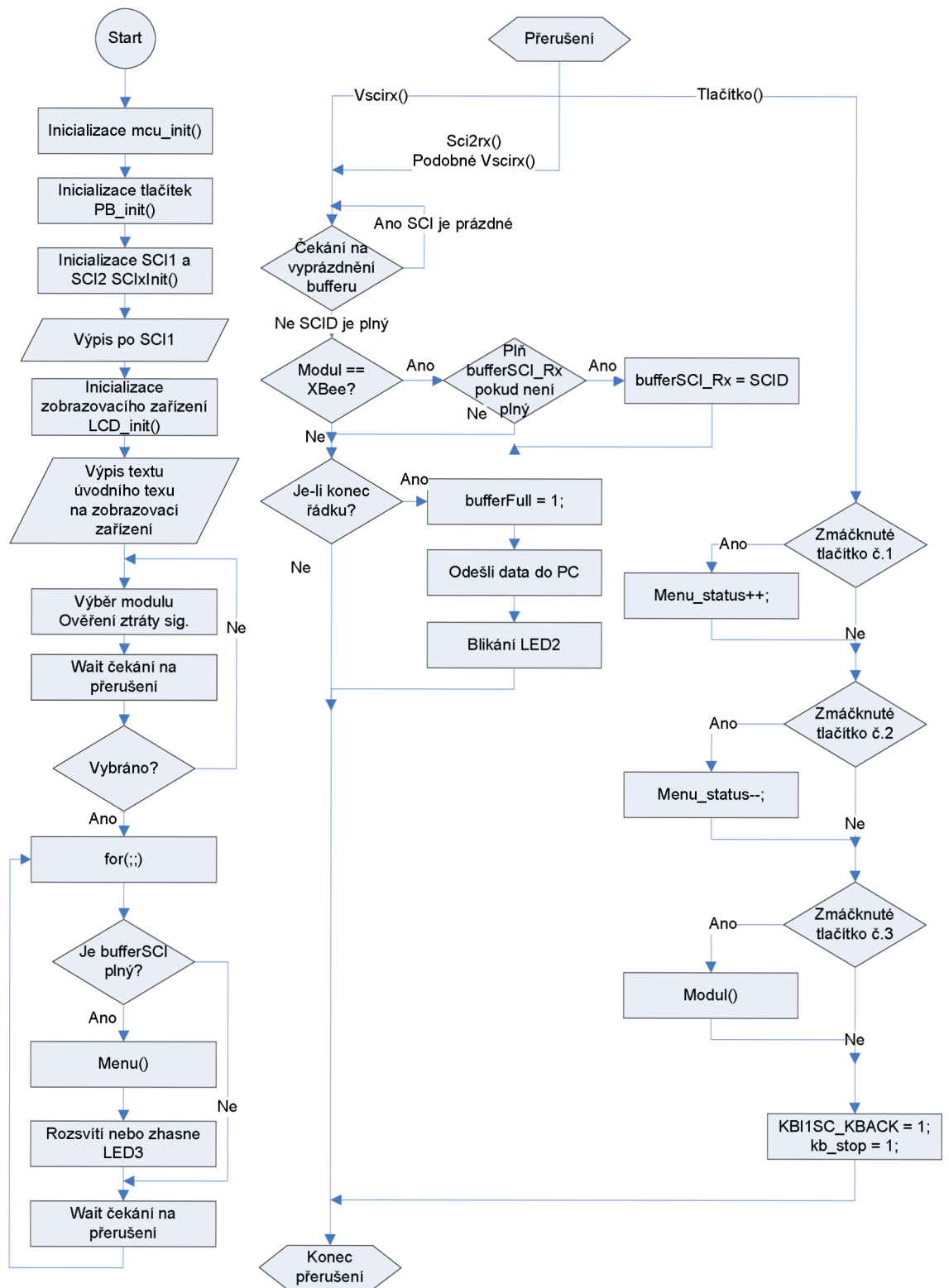
Obr. Příloha B: Vývojový diagram programu nahraného v řídicím procesoru MC9S08GB60
