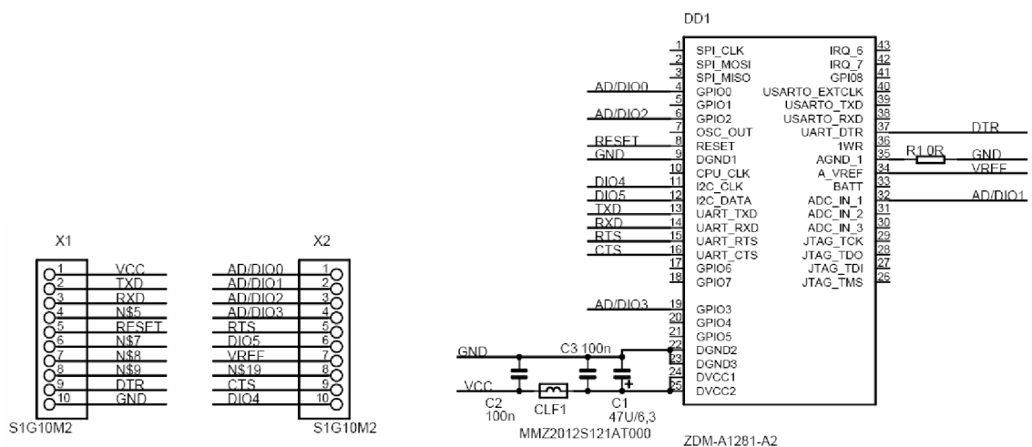
Obr. 2.3: a) Rozmístění vývodů na redukci ZigBit XBee b) Schéma připojení ZigBit k pinům
