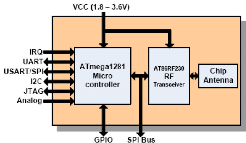
Obr. 2.1: ZDM-A1281-A2 Blokový Diagram
