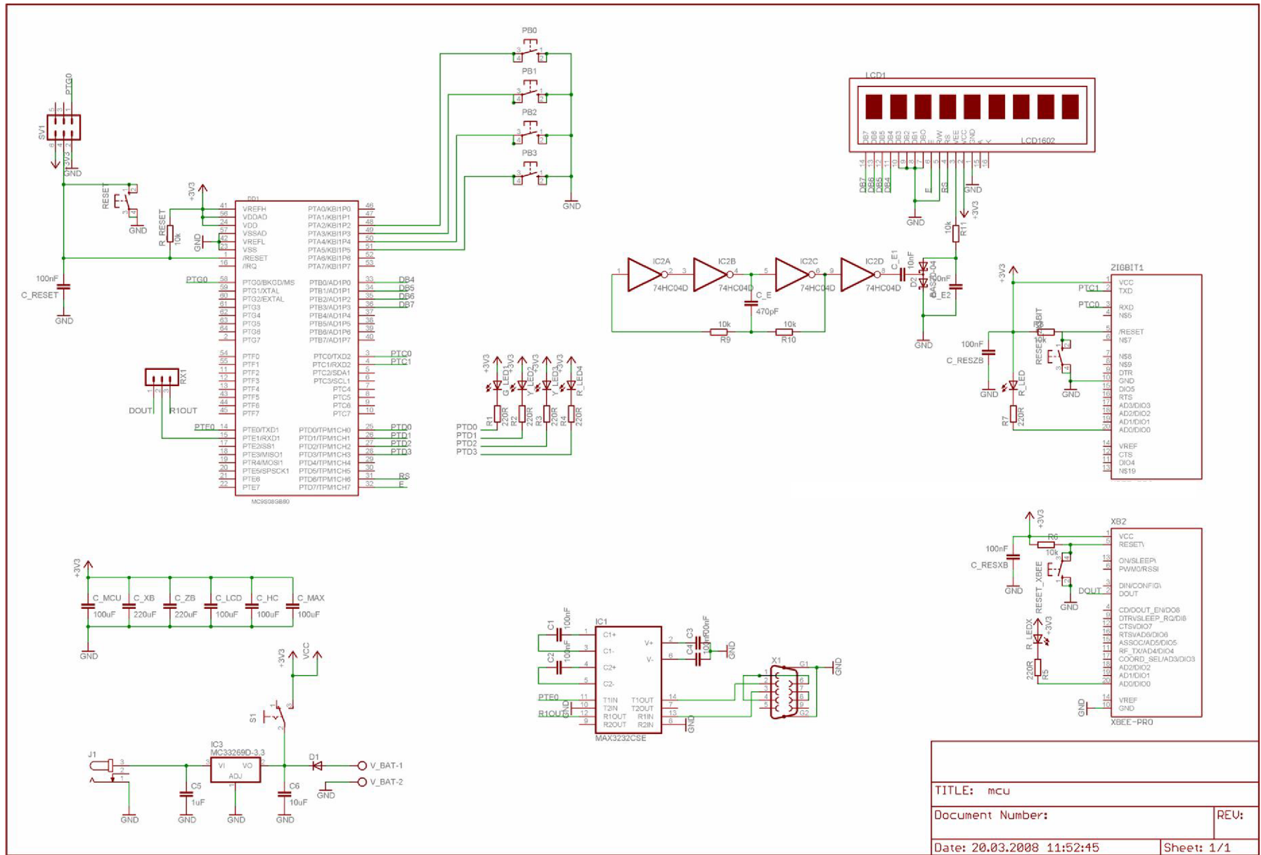
Obr. 8.4: Schéma zapojení přijímače zařízení
