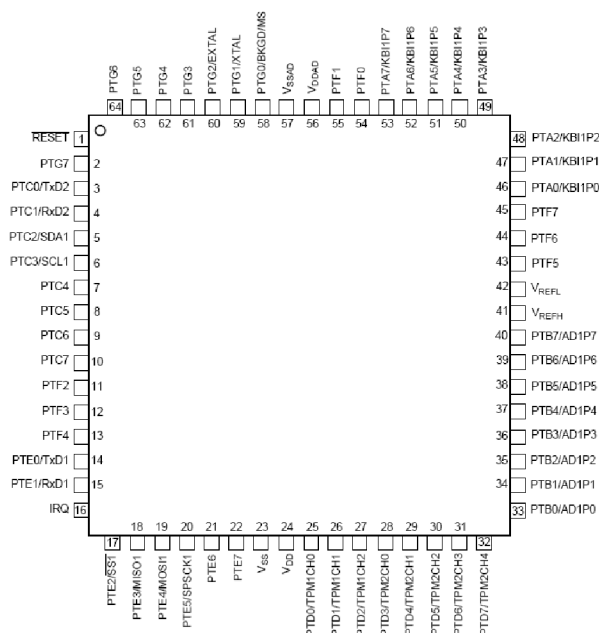
Obr. 4.1: Rozmístění vývodů
