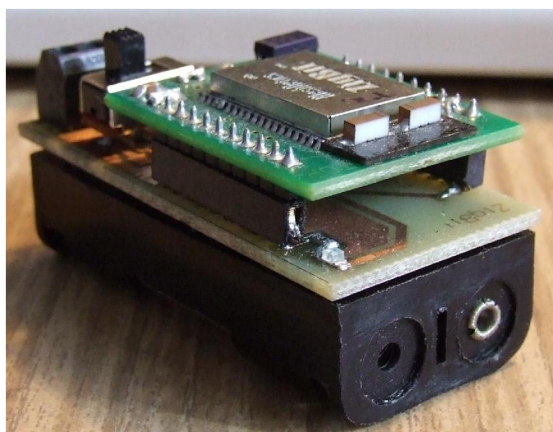
Obr. 8.9: Vysílací zařízení
