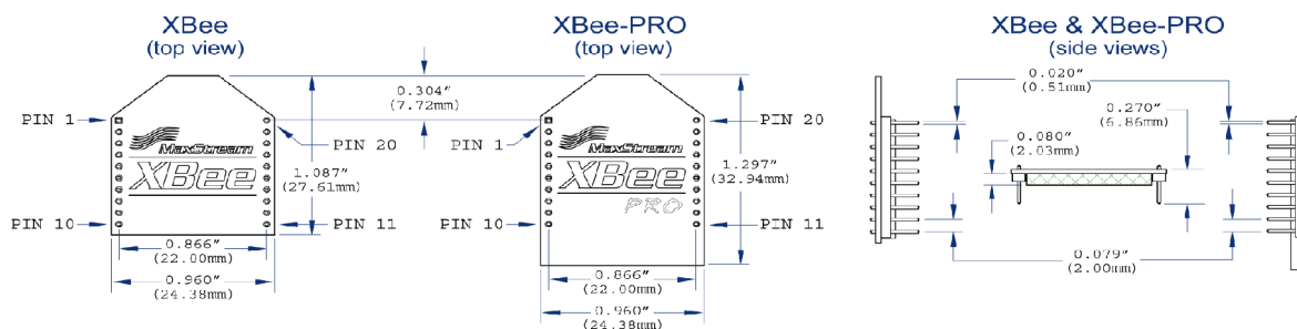
Obr. 3.1: Rozměry a popis Xbee/XBee-PRO
