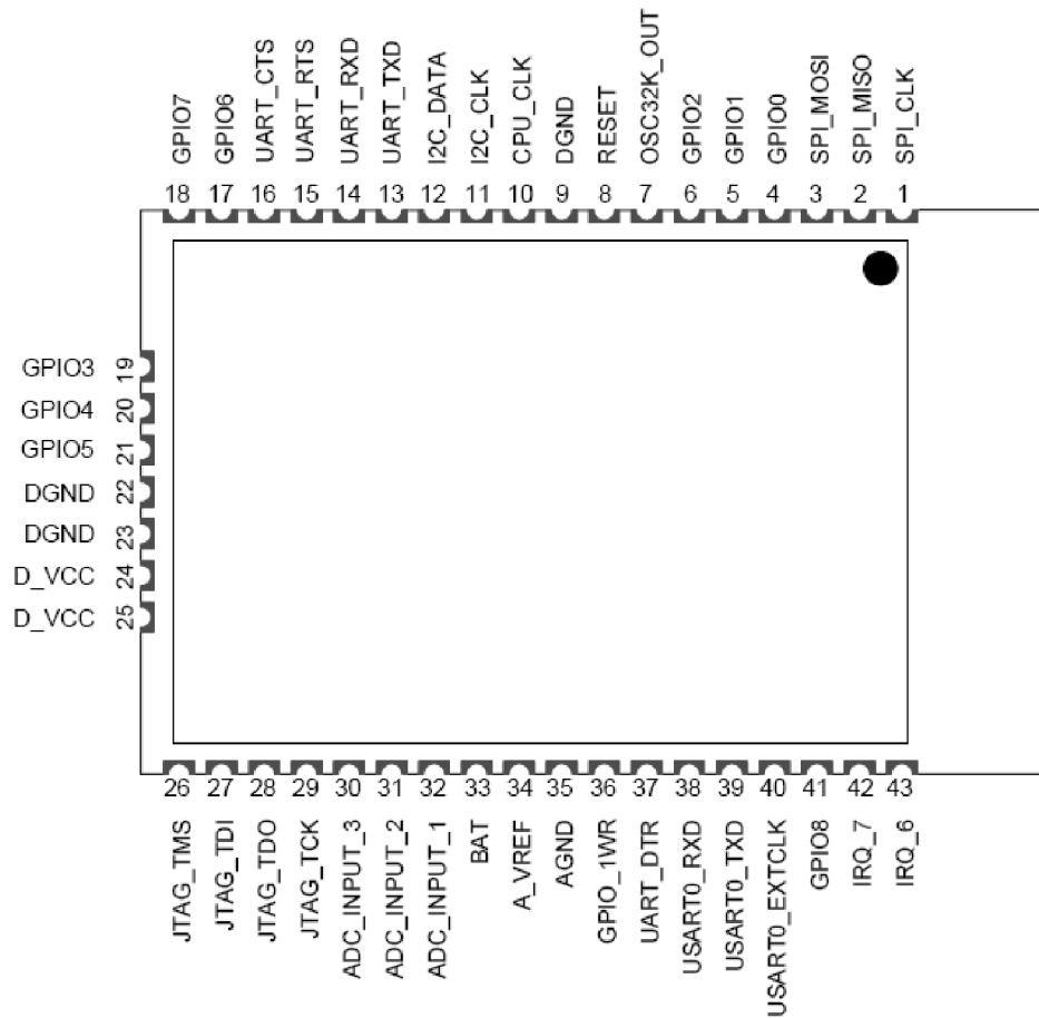
Obr. 2.2: Popis pinů ZigBit (SMD)
