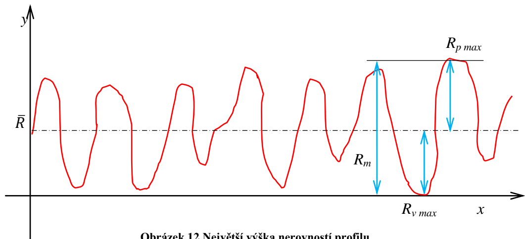
Obrázek 12 Největší výška nerovností profilu.
