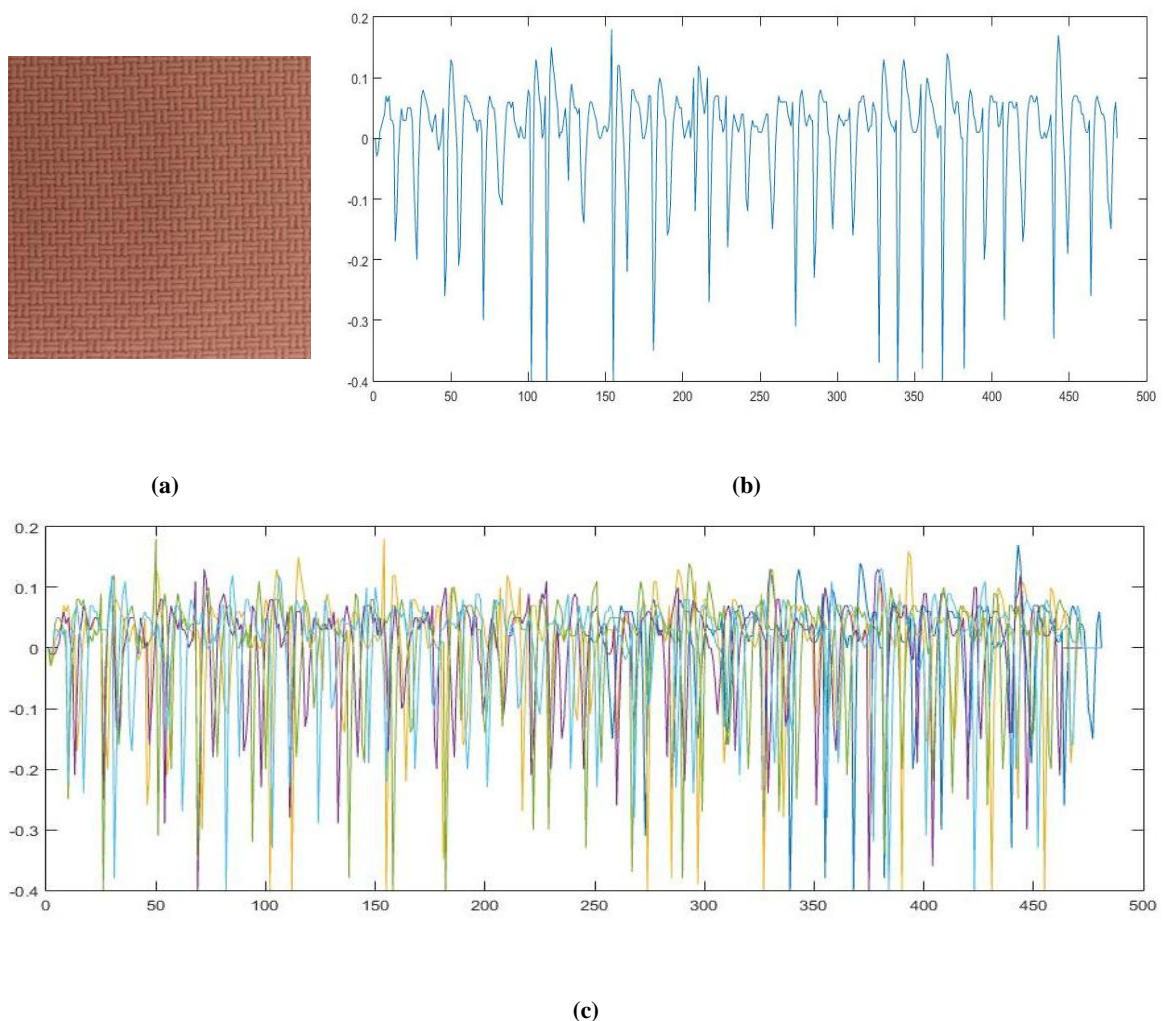
Obrázek 27 (a) obrázek vzorku 1, (b) jeden profil měřený přístrojem KES, (c) 6 naměřených profilů naměřených přístrojem KES
