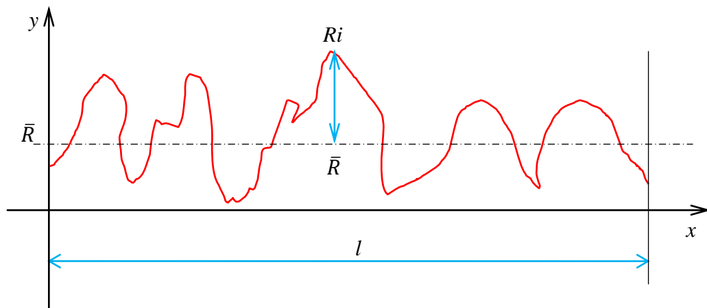
Obrázek 10 Střední aritmetická odchylka profilu.
