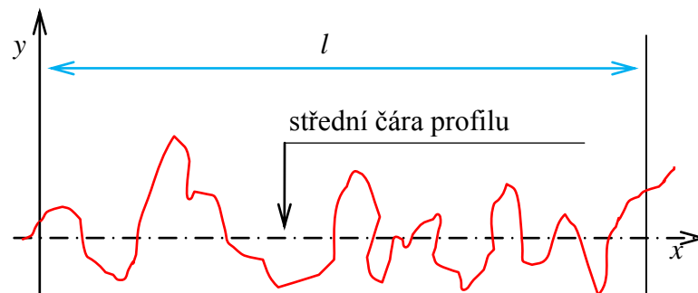
Obrázek 3 Střední čára profilu.
