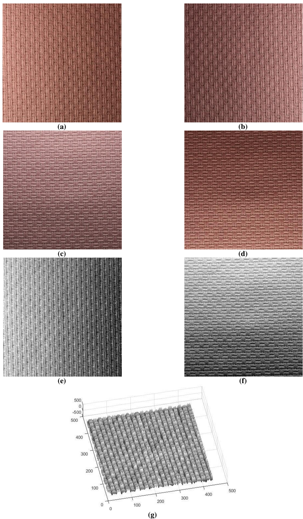
Obrázek 22 (a) levé, (b) pravé, (c) horní, (d) spodní nasvícení vzorku 12, (e) gradientní obraz nasvícený zleva odečtený od obrazu nasvíceného zprava, (f) gradientní obraz nasvícený ze shora odečtený od obrazu nasvíceného zdola, (g) rekonstruovaný 3D povrch vzorku.
