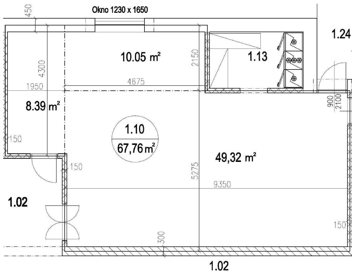
Obr. 2.2 Výpočet podlahové plochy kuchyně
