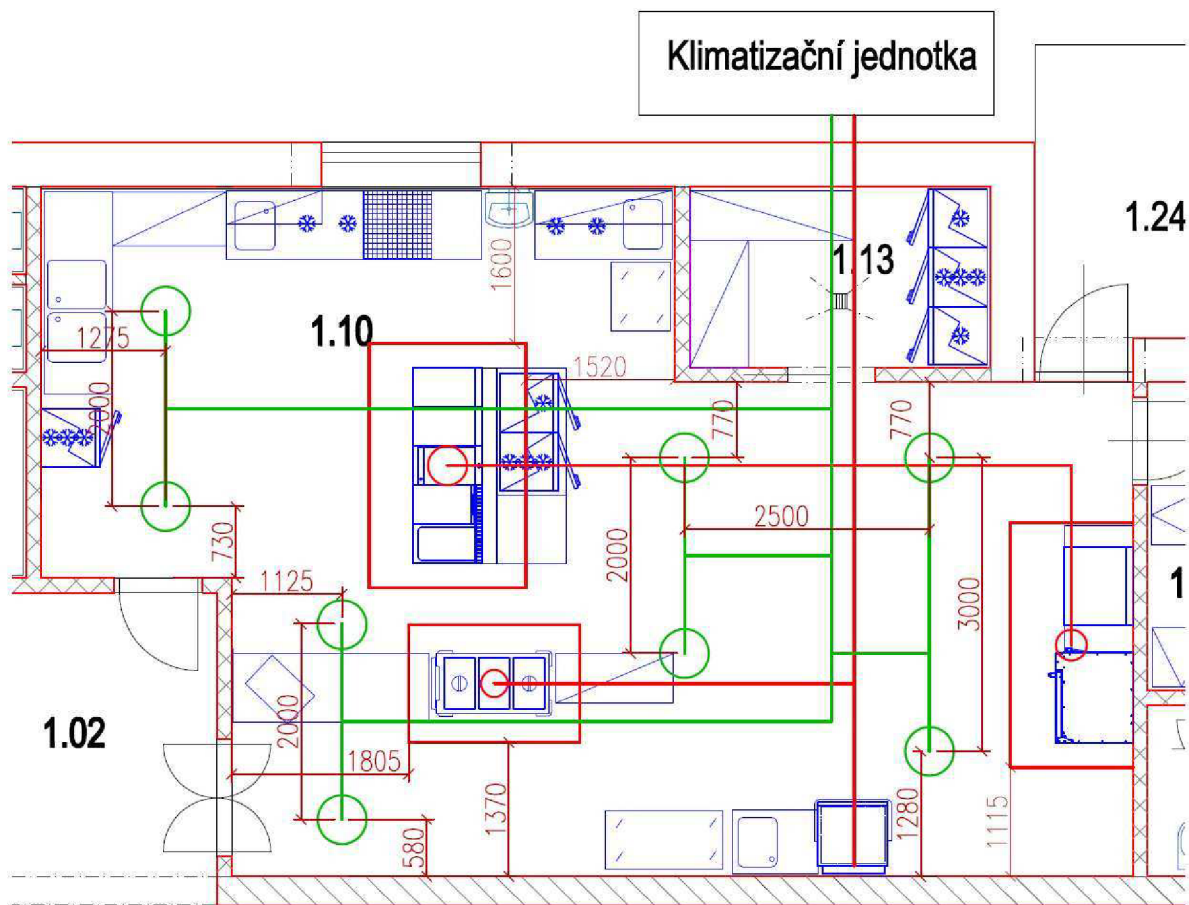
Obr. 6.6 Návrh umístění příváděcích a odváděcích prvků v kuchyni
