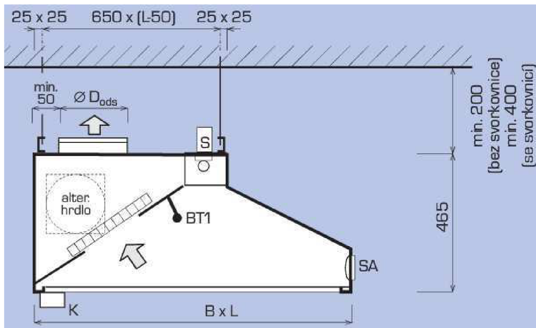
Obr. 6.1 Kuchyňská digestoř Standard-S [9]
