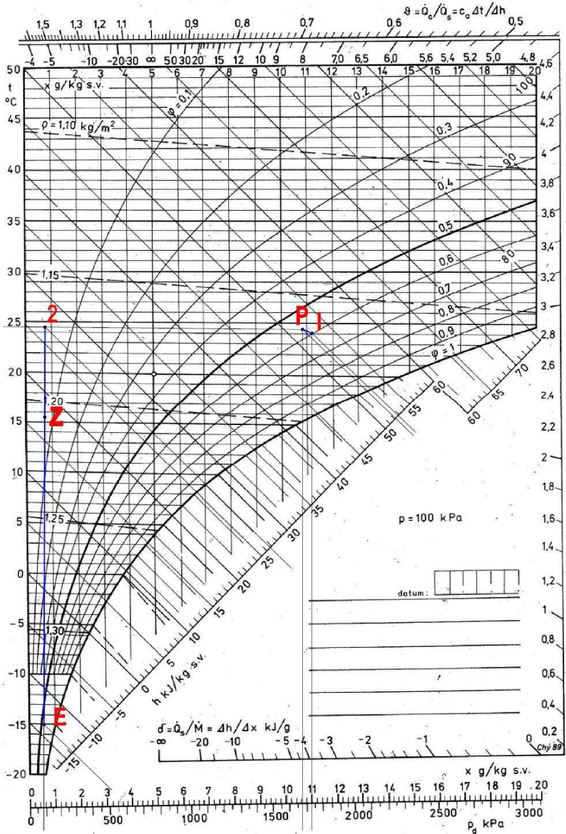
Obr. 5.2 i-x diagram zimního provozu klimatizačního zařízení
