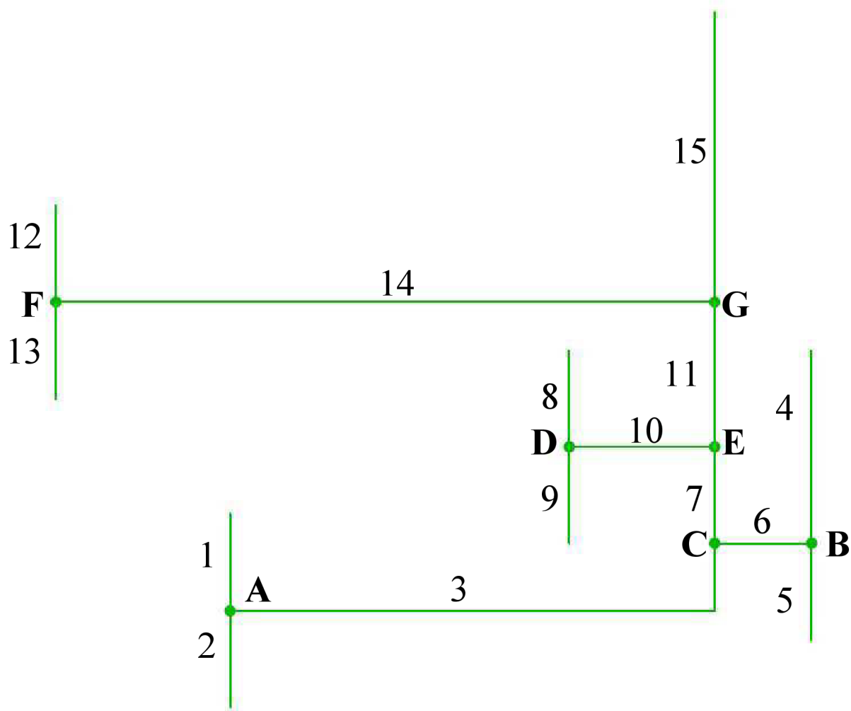
Obr. 7.1. Přívodní síť vzduchovodů
