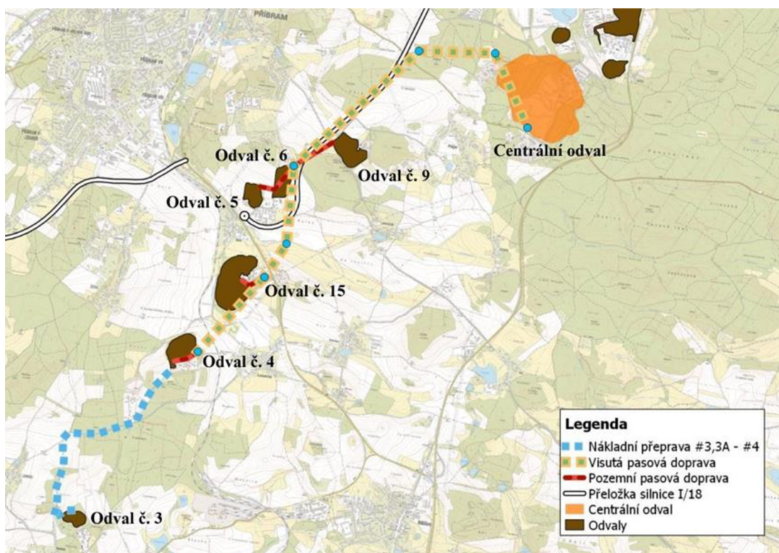
Obrázek 16: Návrh na realizaci přesunu odvalů.
