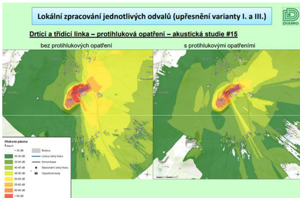
Obrázek 10: Drtící a třídící linka pro zpracování odvalů - protihluková opatření.
