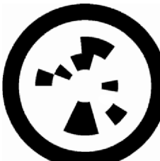
(o) Cantag [47], 2006
