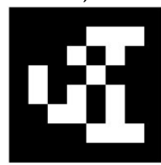
(h) AprilTag [65], 2011
