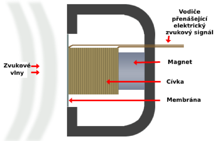
Obrázek 1 Dynamický mikrofon
