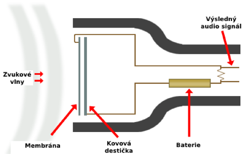
Obrázek 2 Kondenzátorový mikrofon
