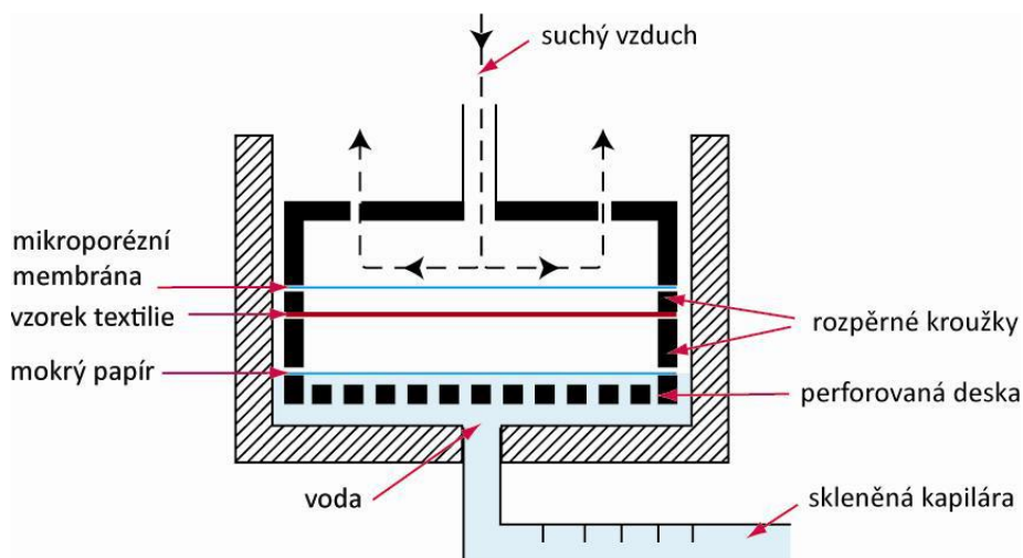
Obrázek 11: Farnworthův difuzimetr [8]
