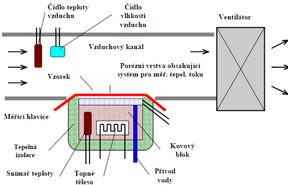
Obrázek 8: Schéma Permetestu [8]
